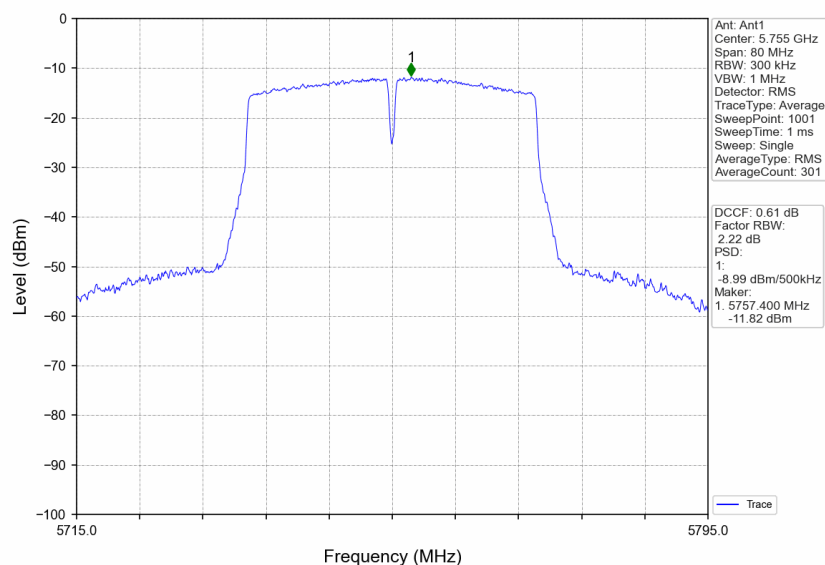
802.11n(HT40)_LCH_5755MHz_Ant1_NTNV
