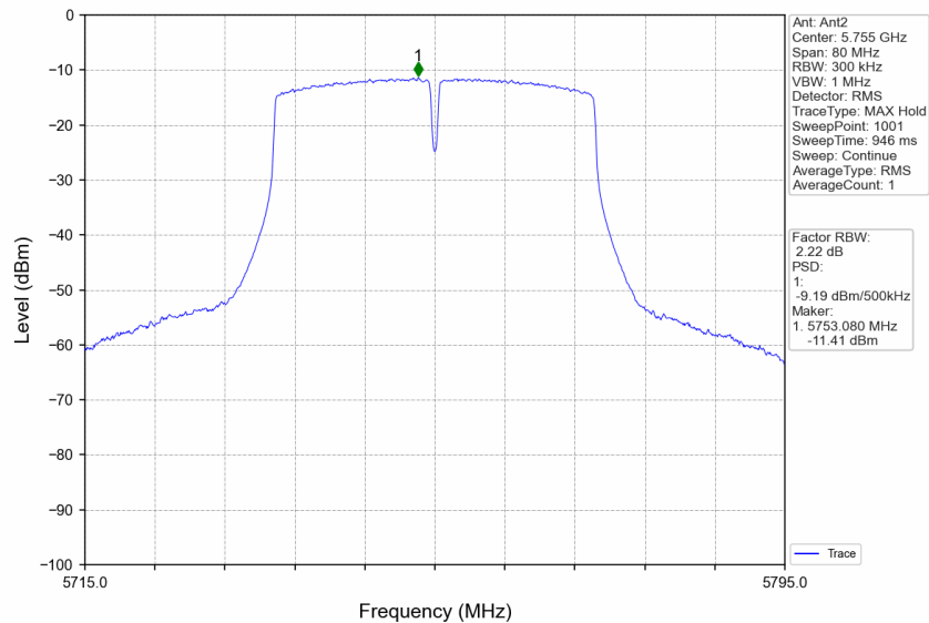
802.11n(HT40)_LCH_5755MHz_MIMO_NTNV
