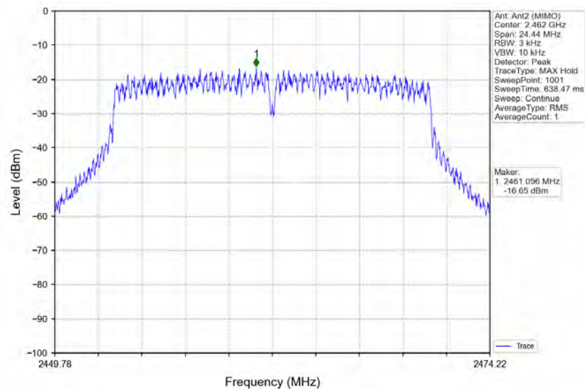
802.11n(HT20)_HCH_2462MHz_Ant2 (MIMO)_NTNV
