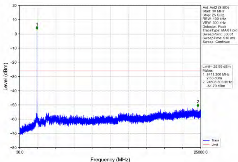
802.11b_LCH_2412MHz_Ant2 (SISO)_NTNV
