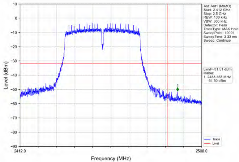
802.11n(HT40)_HCH_2452MHz_Ant1 (MIMO)_NTNV
