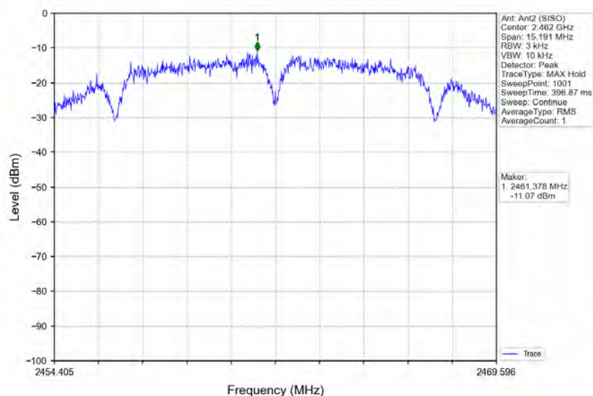
802.11b_HCH_2462MHz_Ant2 (SISO)_NTNV
