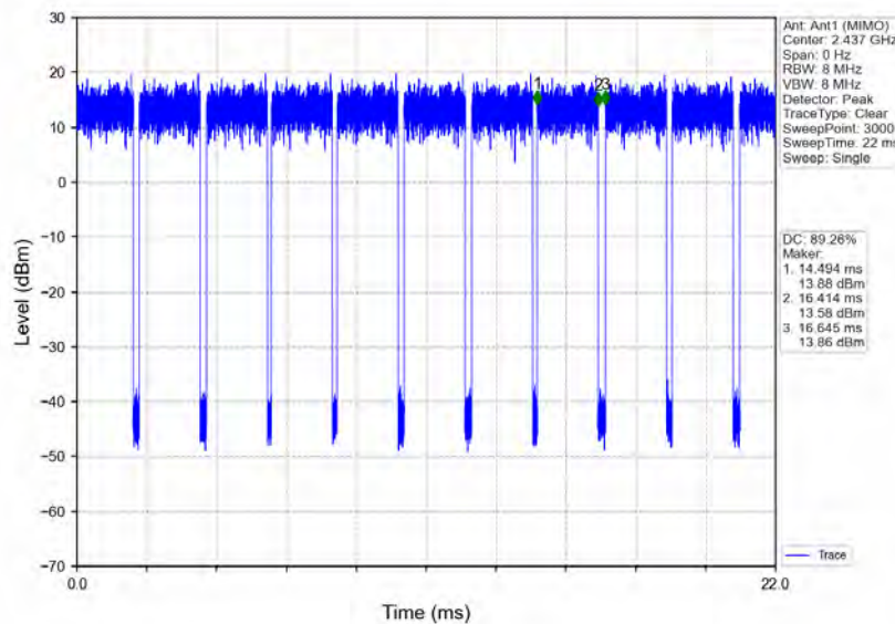
802.11n(HT20)_MCH_2437MHz_Ant1 (MIMO)_NTNV
