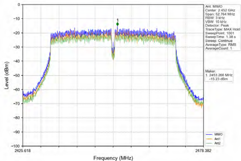
802.11n(HT40)_HCH_2452MHz_MIMO_NTNV
