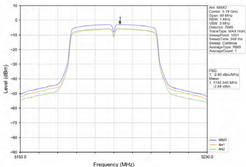
802.11n(HT40) LCH 5190MHz MIMO NTN
