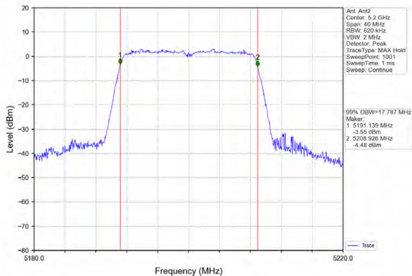
802.11n(HT20)_MCH_5200MHz_Ant2_NTNV
