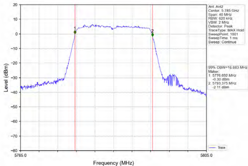
802.11a_MCH_5785MHz_Ant2_NTNV
