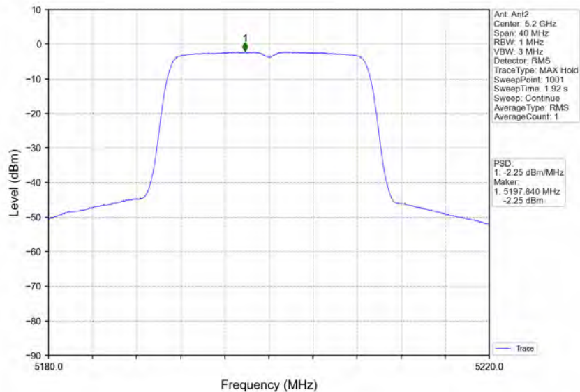
802.11n(HT20)_MCH_5200MHz_MIMO_NTNV
