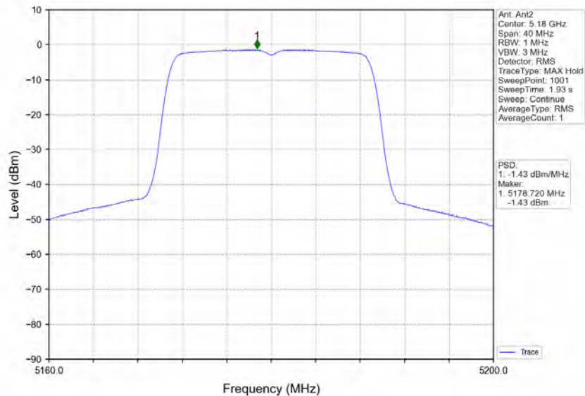
802.11ac(VHT20) LCH 5180MHz MIMO NTNV
