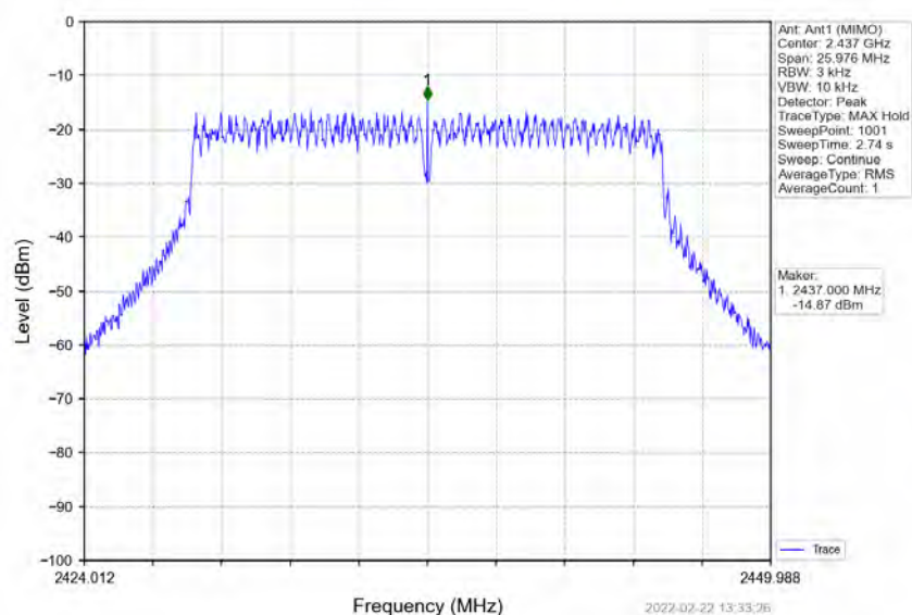
802.11n(HT20)_MCH_2437MHz_Ant1 (MIMO)_NTNV
