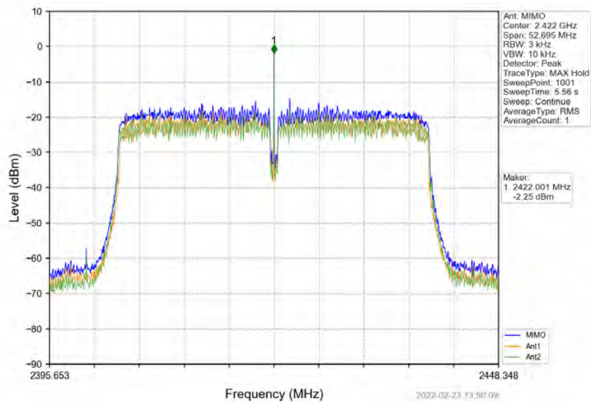
802.11n(HT40) LCH_2422MHz_MIMO_NTNV
