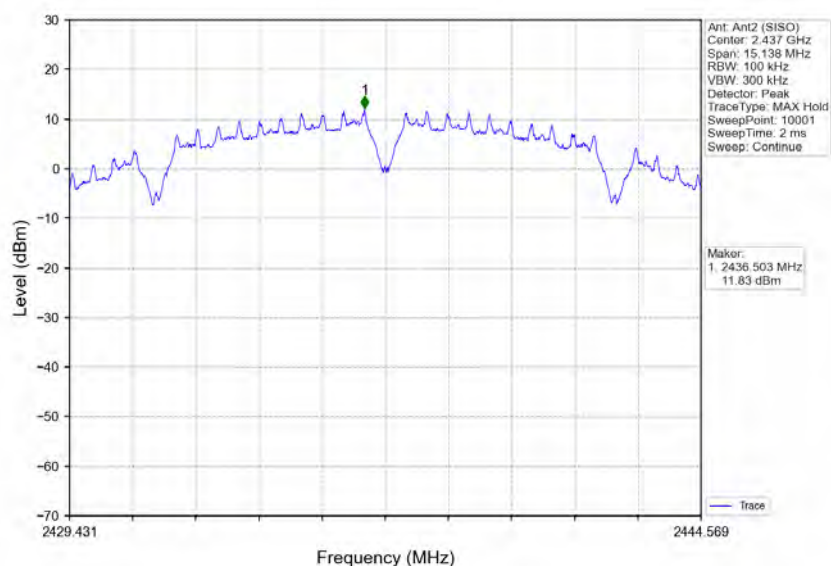
802.11b_MCH_2437MHz_Ant2 (SISO)_NTNV
