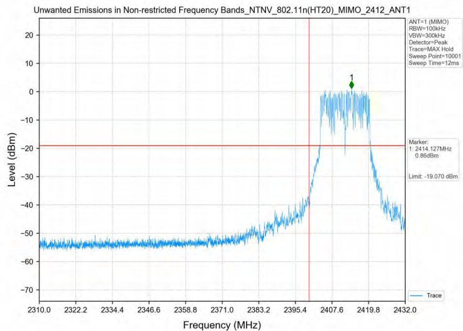
802.11n(HT20) 2412MHz MIMO Total
