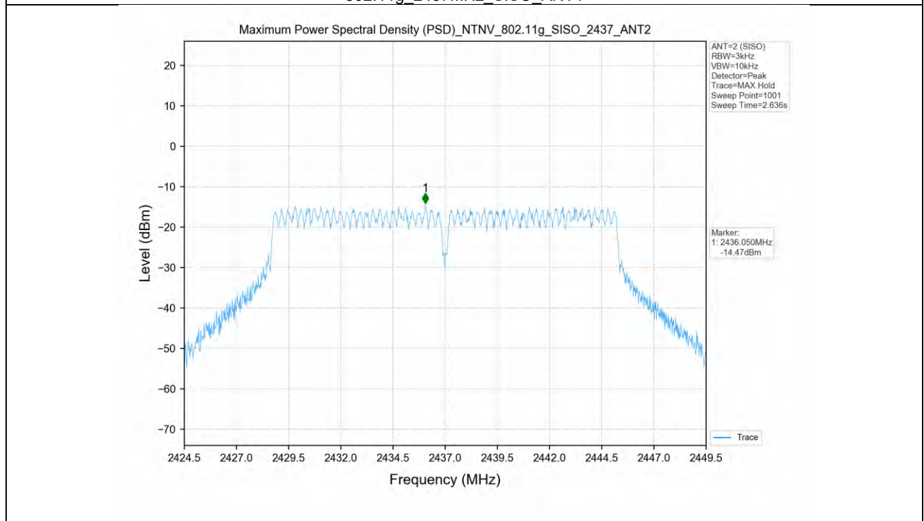
802.11g_2437MHz_SISO_ANT2
