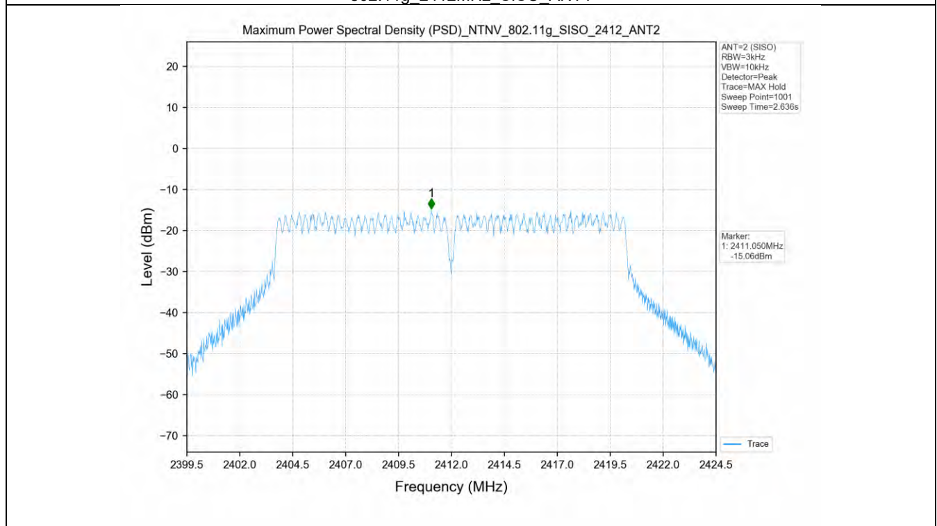
802.11g_2412MHz_SISO_ANT2
