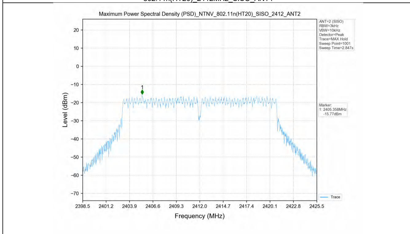
802.11n(HT20)_2412MHz_SISO_ANT2
