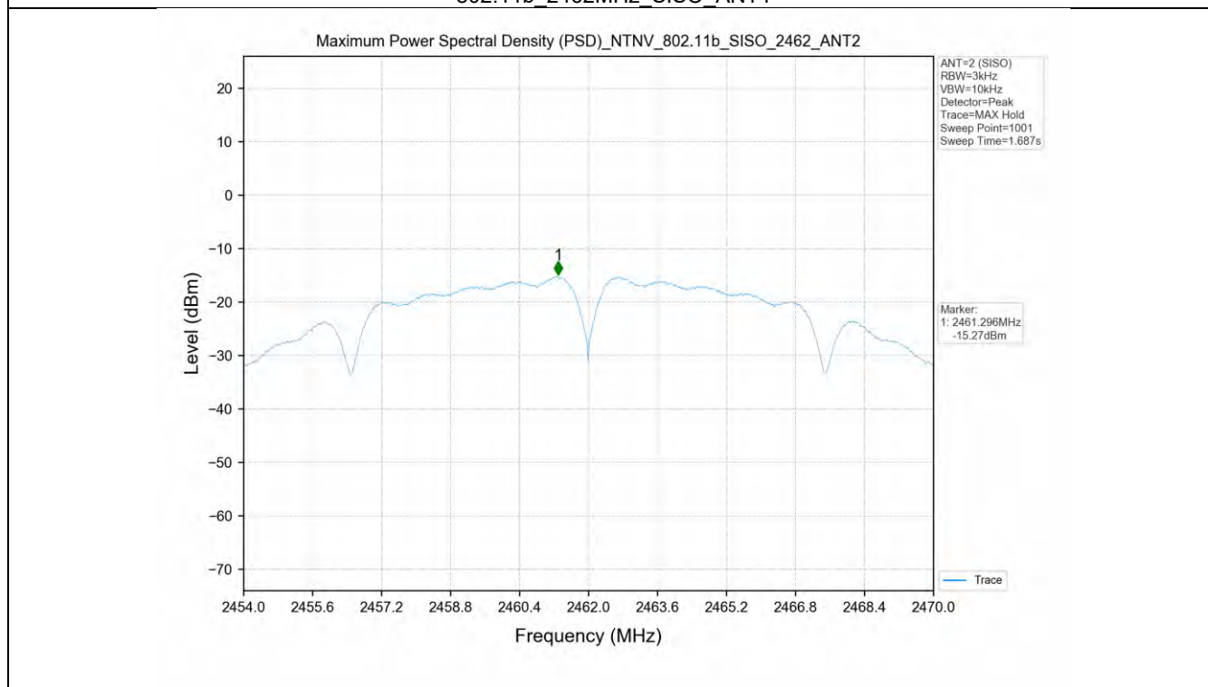
802.11b_2462MHz_SISO_ANT2
