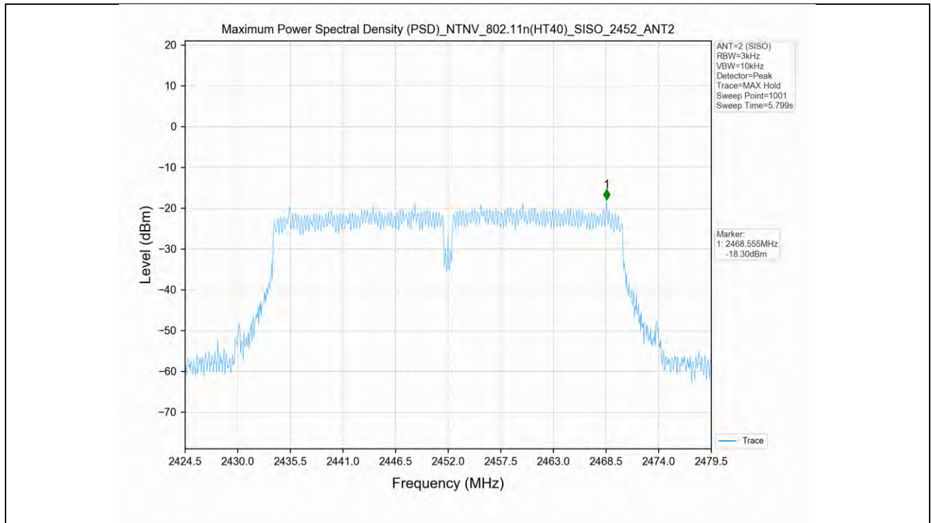
802.11n(HT40)_2452MHz_SISO_ANT2
