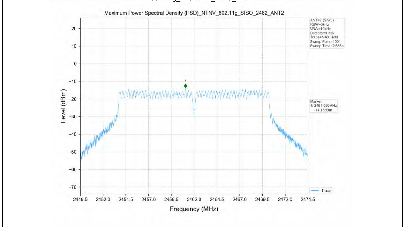
802.11g_2462MHz_SISO_ANT2
