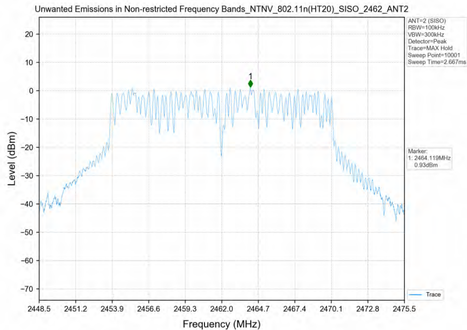
802.11n(HT20)_SISO_ANT2_REF
