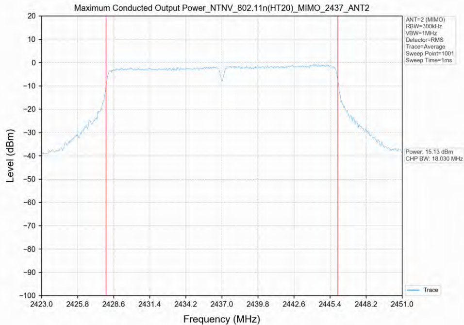
802.11n(HT20)_2437MHz_MIMO_ANT2
