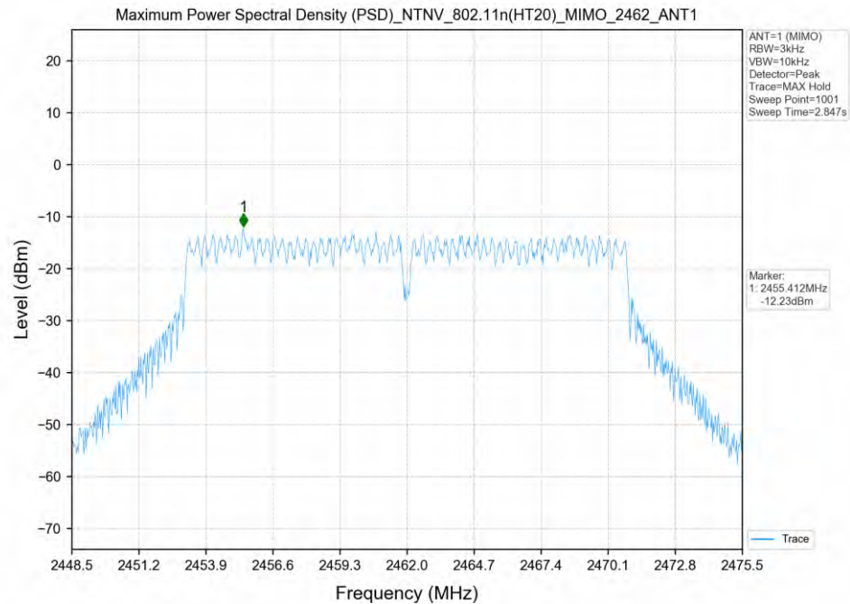
802.11n(HT20)_2462MHz_MIMO_ANT1
