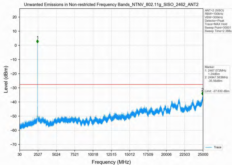
802.11g_2462MHz_SISO_ANT2
