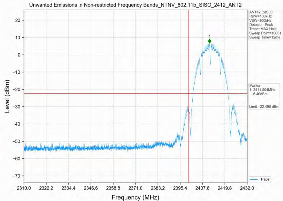
802.11b_2412MHz_SISO_ANT2
