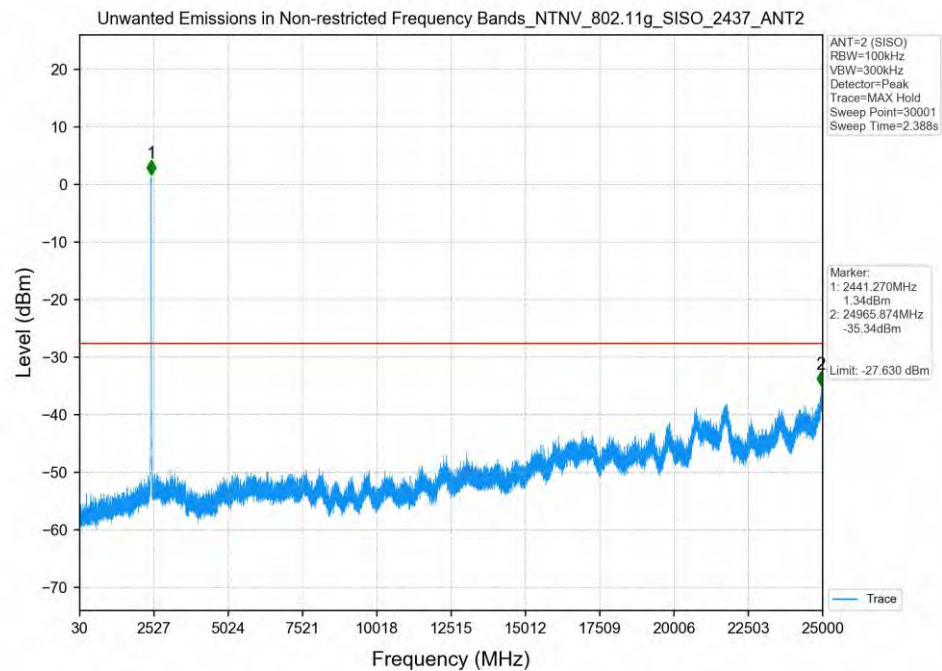
802.11g_2437MHz_SISO_ANT2
