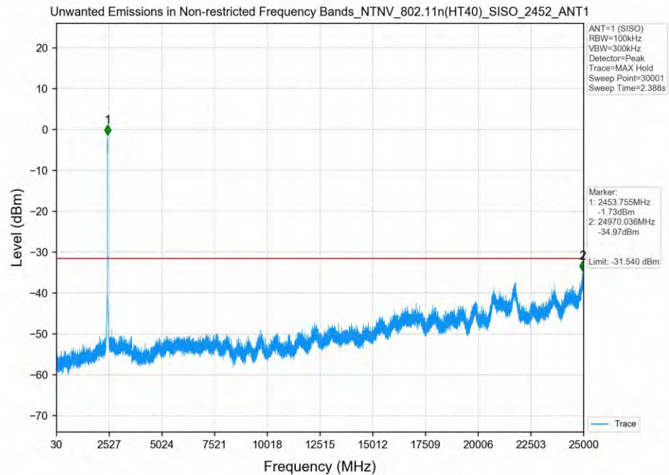
802.11n(HT40)_2452MHz_SISO_ANT1
