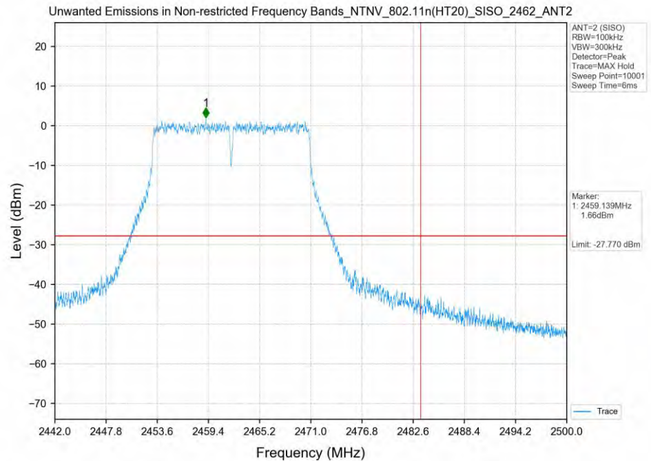
802.11n(HT20)_2462MHz_SISO_ANT2
