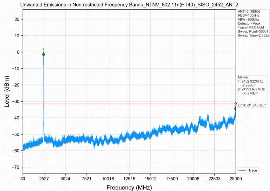
802.11n(HT40)_2452MHz_SISO_ANT2
