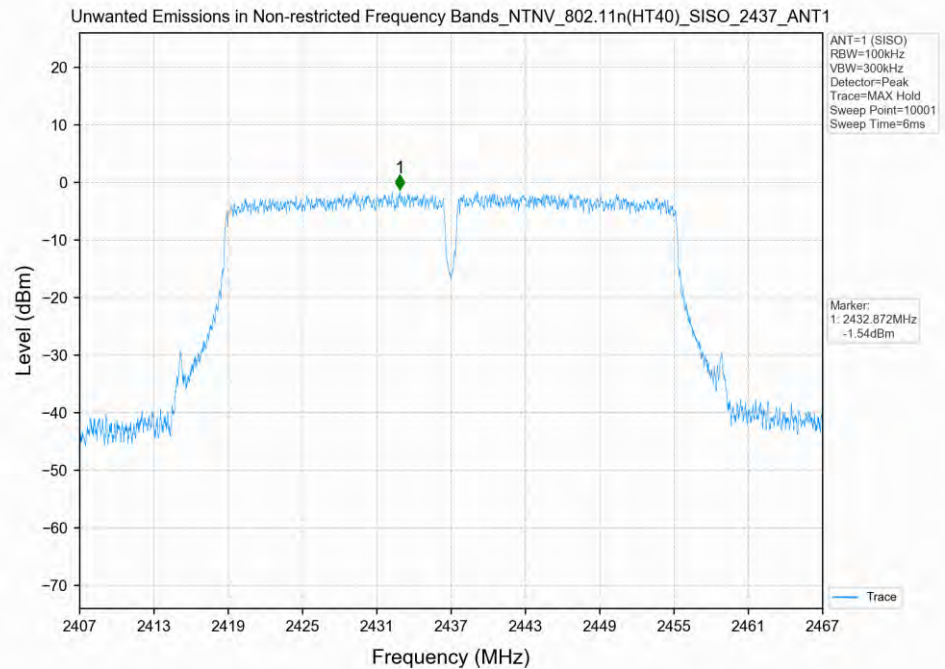
802.11n(HT40)_SISO_ANT1_REF
