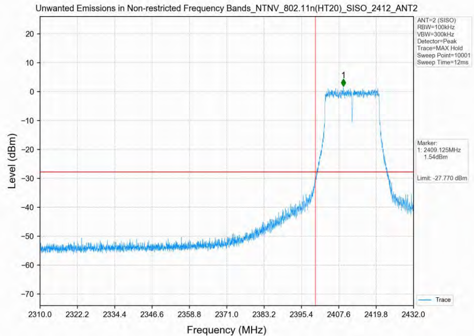
802.11n(HT20)_2412MHz_SISO_ANT2
