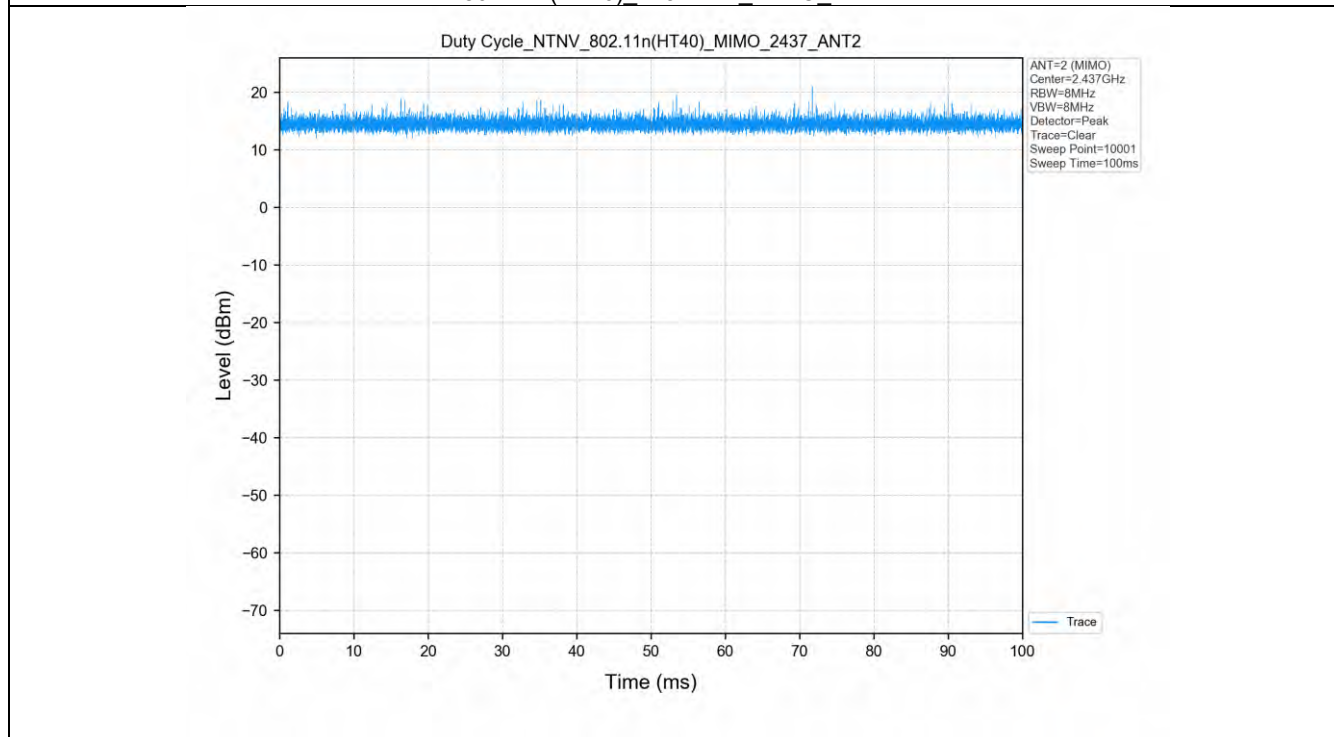
802.11n(HT40)_2437MHz_MIMO_ANT2
