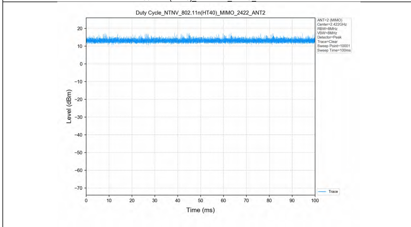
802.11n(HT40)_2422MHz_MIMO_ANT2
