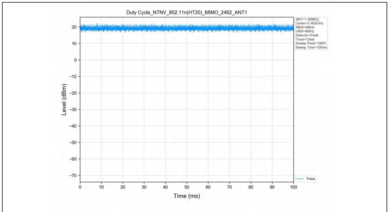
802.11n(HT20)_2462MHz_MIMO_ANT1
