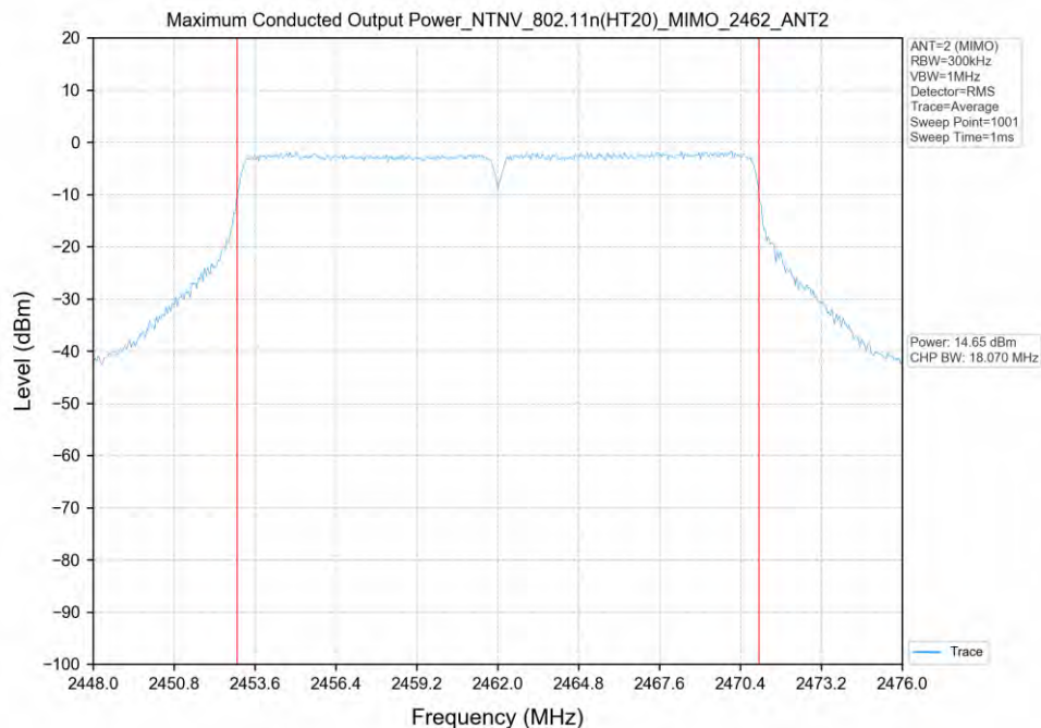
802.11n(HT20)_2462MHz_MIMO_ANT2
