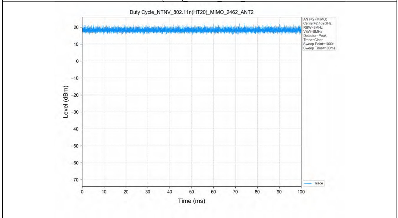
802.11n(HT20)_2462MHz_MIMO_ANT2
