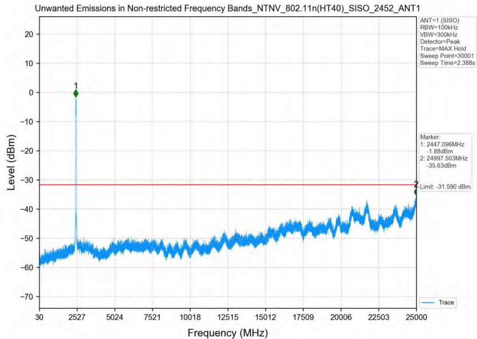
802.11n(HT40)_2452MHz_SISO_ANT1
