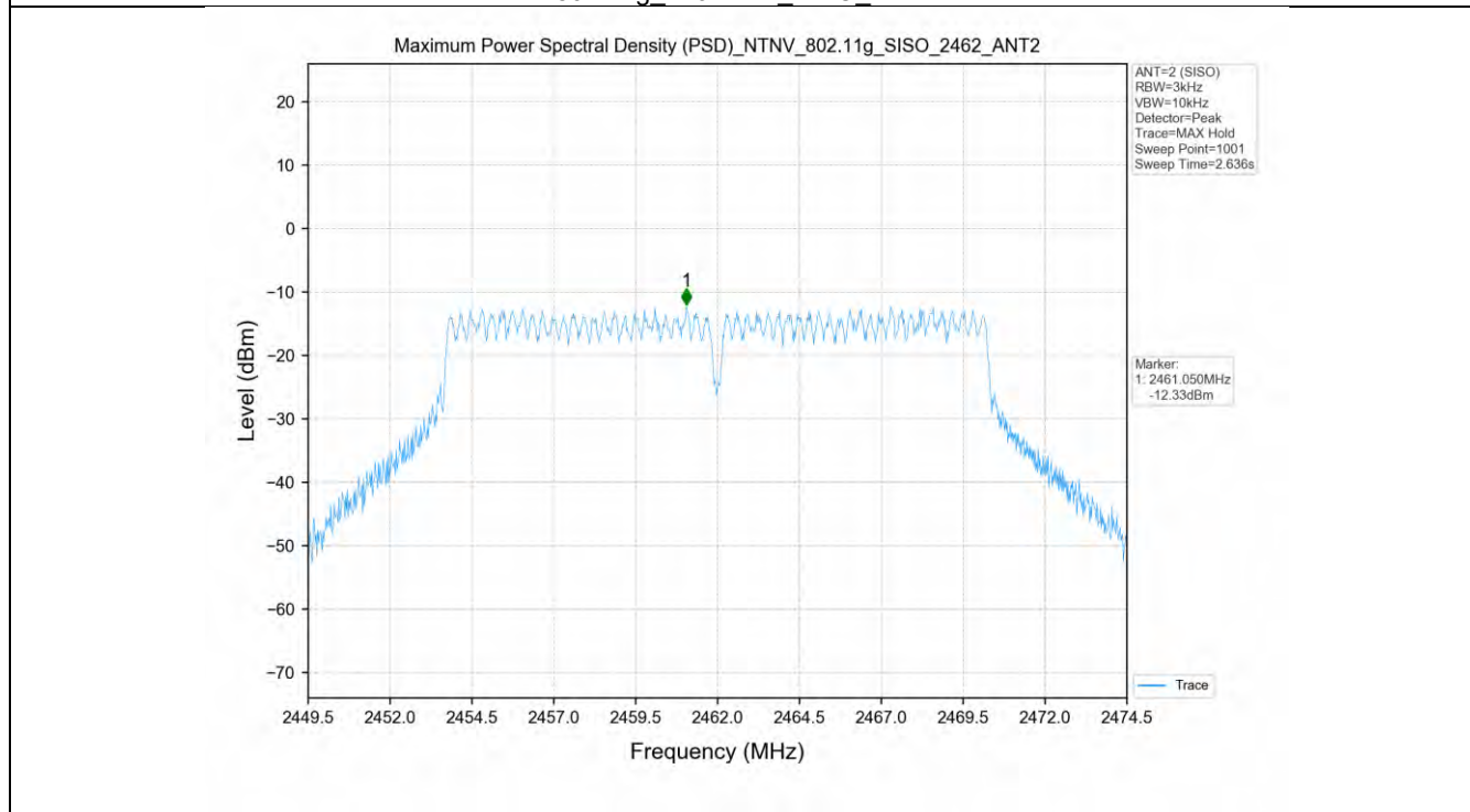
802.11g_2462MHz_SISO_ANT2
