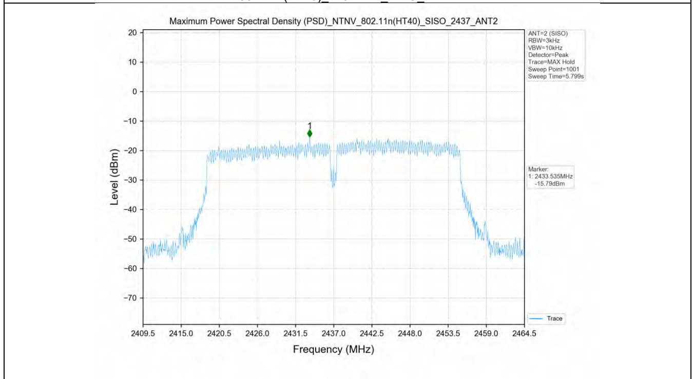
802.11n(HT40)_2437MHz_SISO_ANT2
