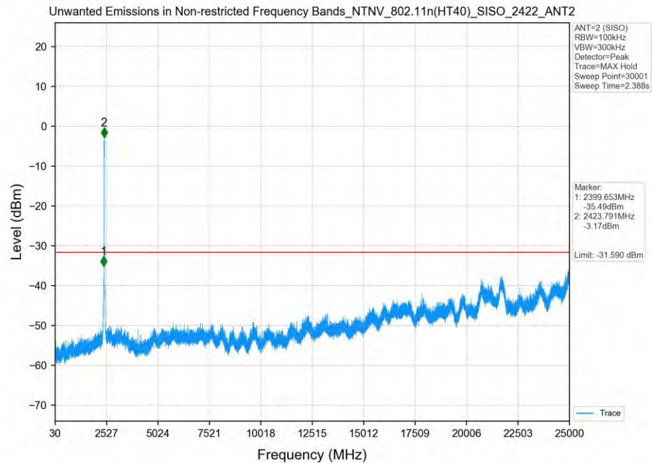
802.11n(HT40)_2422MHz_SISO_ANT2
