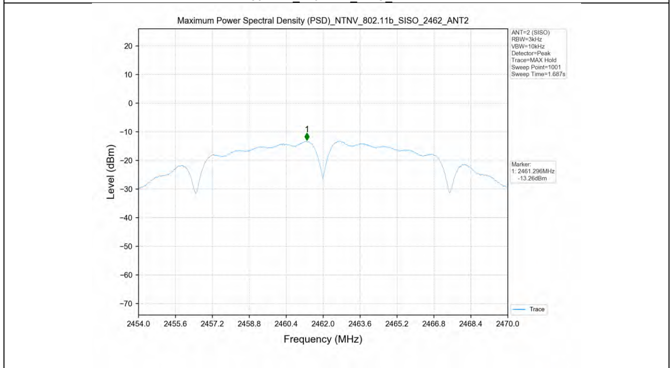
802.11b_2462MHz_SISO_ANT2
