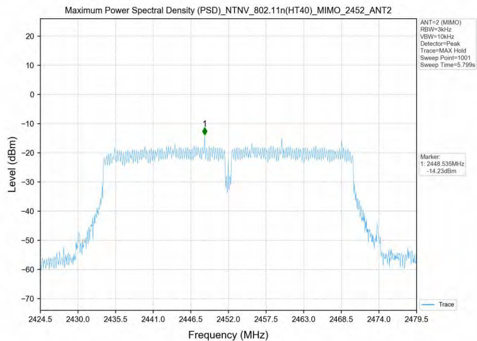
802.11n(HT40)_2452MHz_MIMO_ANT2
