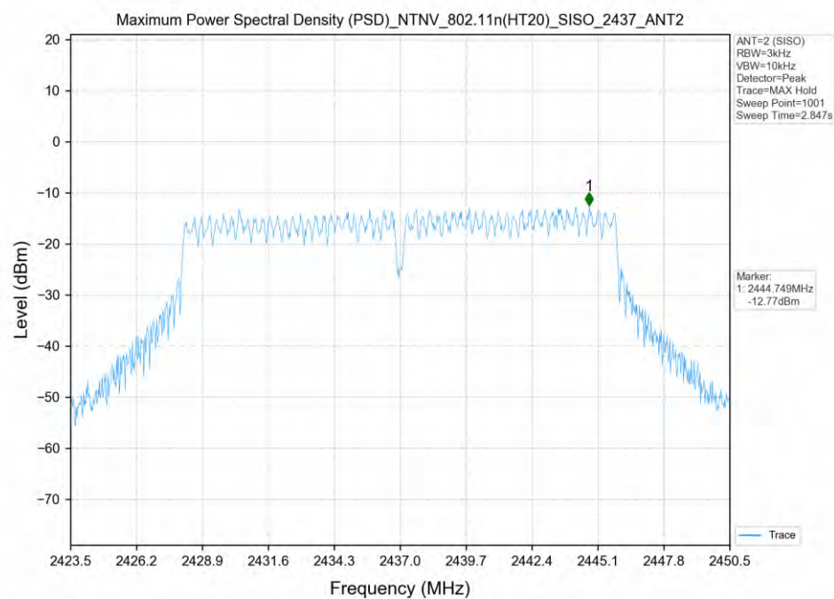
802.11n(HT20)_2437MHz_SISO_ANT2
