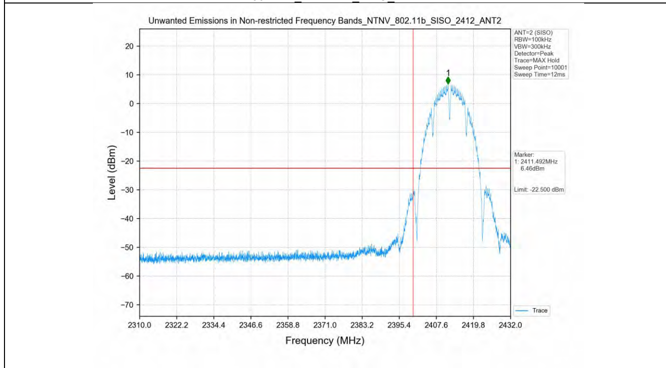
802.11b_2412MHz_SISO_ANT2
