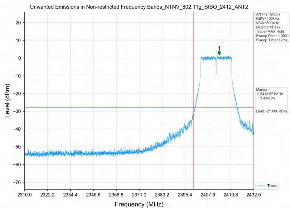
802.11g_2412MHz_SISO_ANT2
