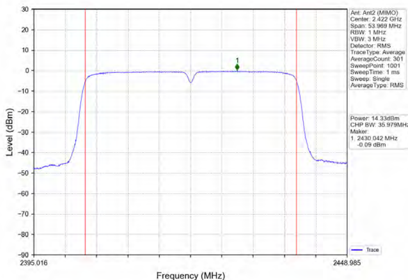
802.11n(HT40)_LCH_2422MHz_Ant2 (MIMO)_NTNV
