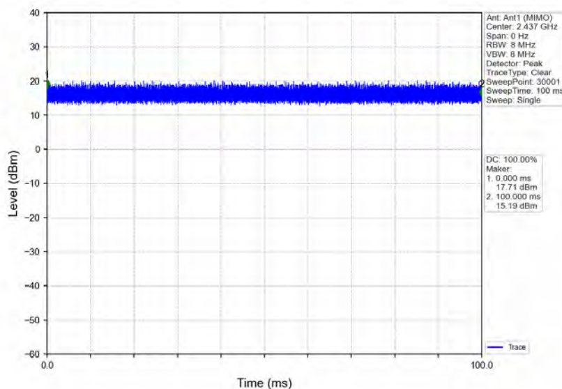
802.11n(HT20)_MCH_2437MHz_Ant1 (MIMO)_NTNV
