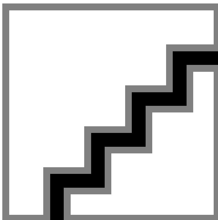
Figure 8-9 Face Parameters
