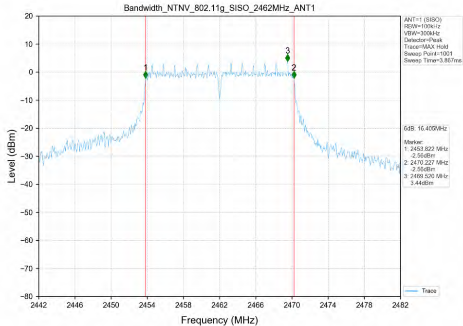
802.11g_2462MHz_SISO_ANT1
