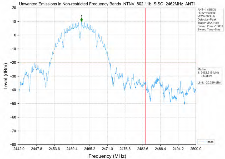
802.11b_2462MHz_SISO_ANT1
