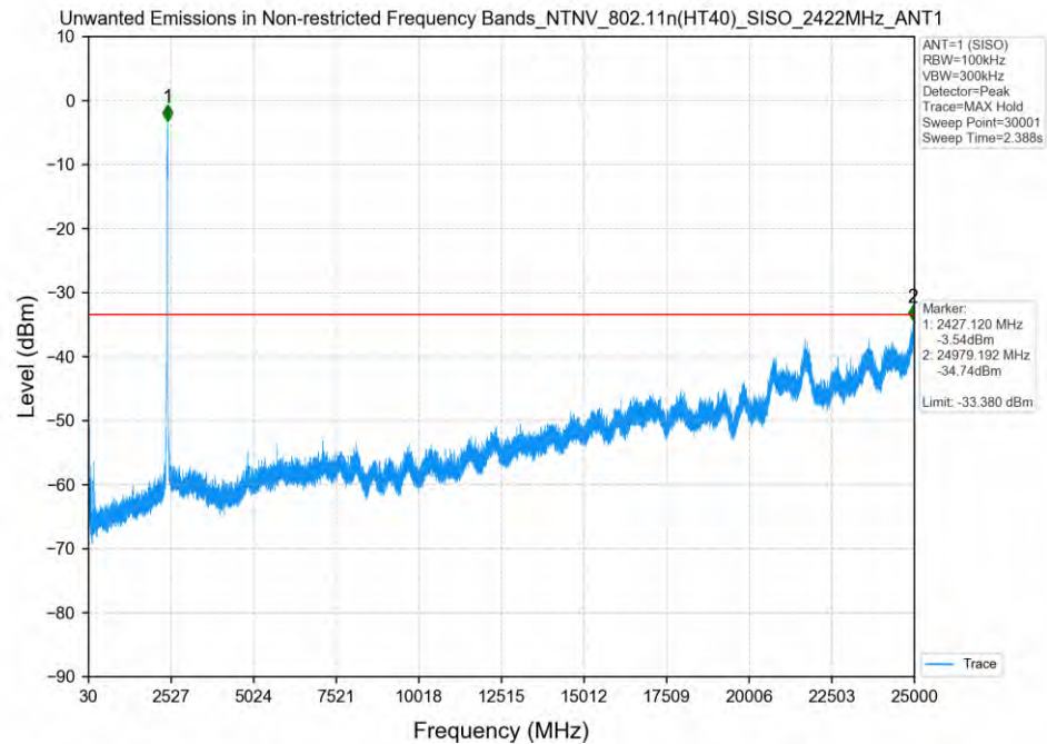
802.11n(HT40)_2422MHz_SISO_ANT1
