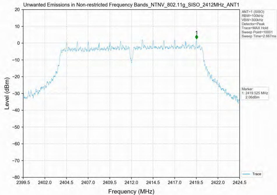
802.11g_SISO_ANT1_REF
