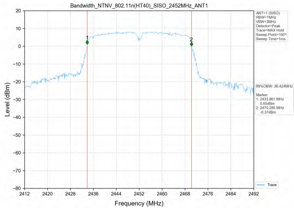
802.11n(HT40)_2452MHz_SISO_ANT1
