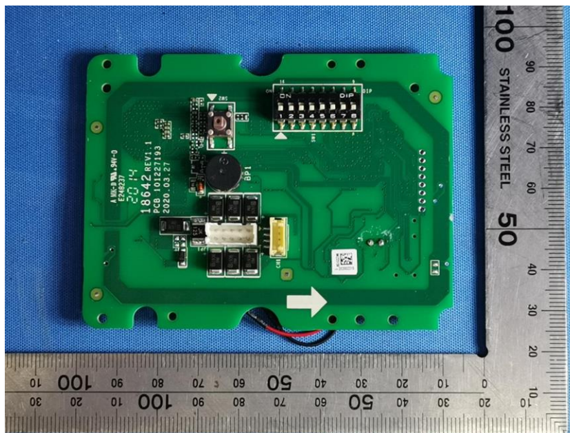
125KHz Module
