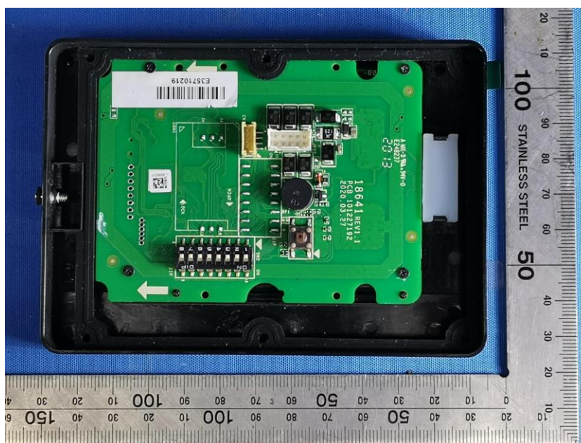
125KHz Module
