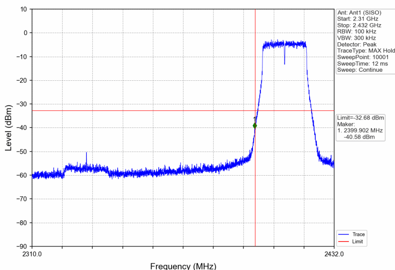
802.11n(HT20)_LCH_2412MHz_Ant1 (SISO)_NTNV
