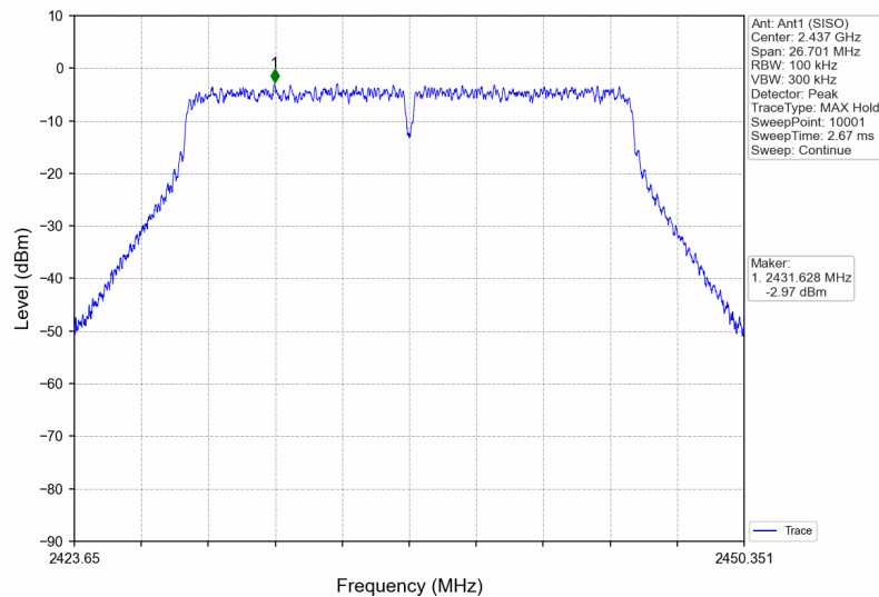
802.11n(HT20)_MCH_2437MHz_Ant1 (SISO)_NTNV
