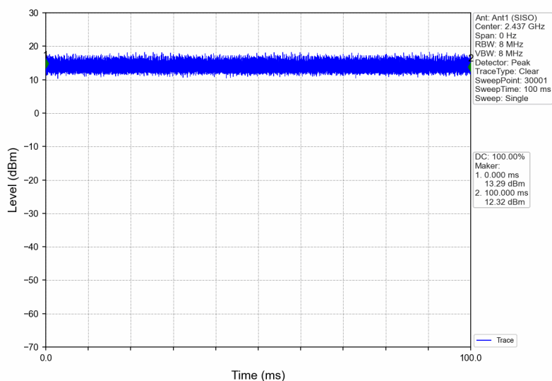
802.11n(HT20)_MCH_2437MHz_Ant1 (SISO)_NTNV
