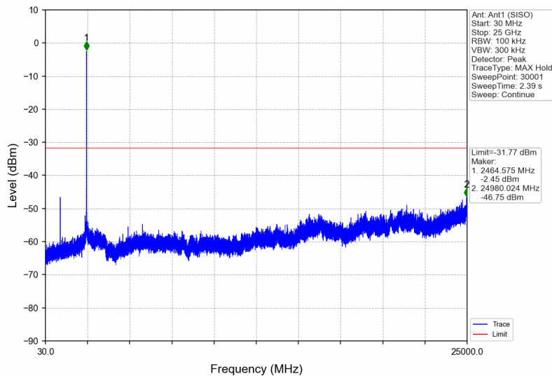
802.11g_HCH_2462MHz_Ant1 (SISO)_NTNV
