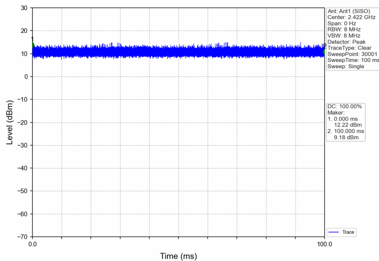
802.11n(HT40) LCH 2422MHz Ant1 (SISO) NTNV
