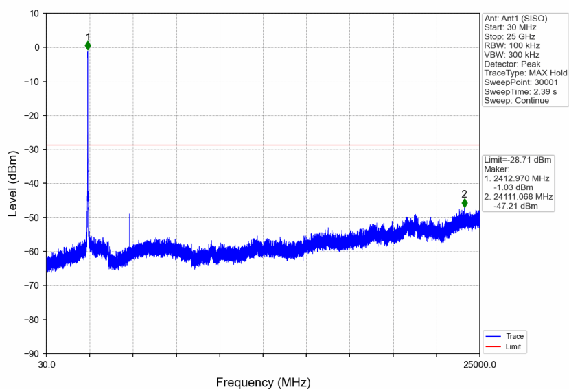
802.11n(HT20)_LCH_2412MHz_Ant1 (SISO)_NTNV
