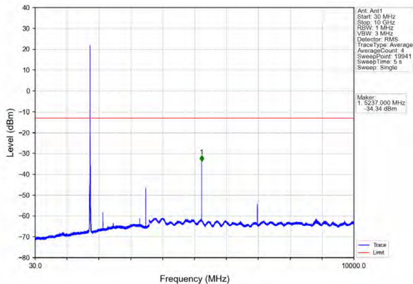
Band4_10MHz_QPSK_HCH_1750MHz_RB_1_0_NTNV
