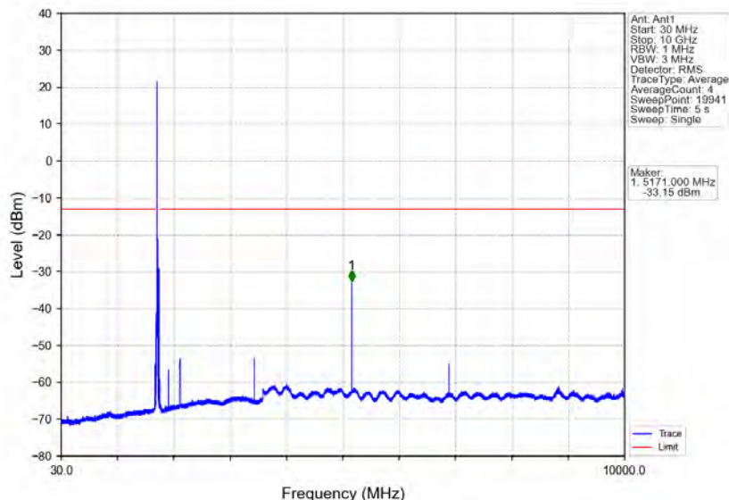
Band4_20MHz_QPSK_MCH_1732.5MHz_RB_1_0_NTNV
