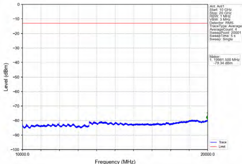
Band4_20MHz_16QAM_LCH_1720MHz_RB_100_0_NTNV
