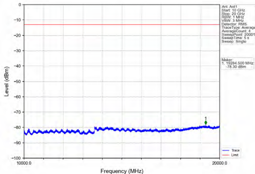
Band4 10MHz 64QAM HCH 1750MHz RB 1 0 NTNV
