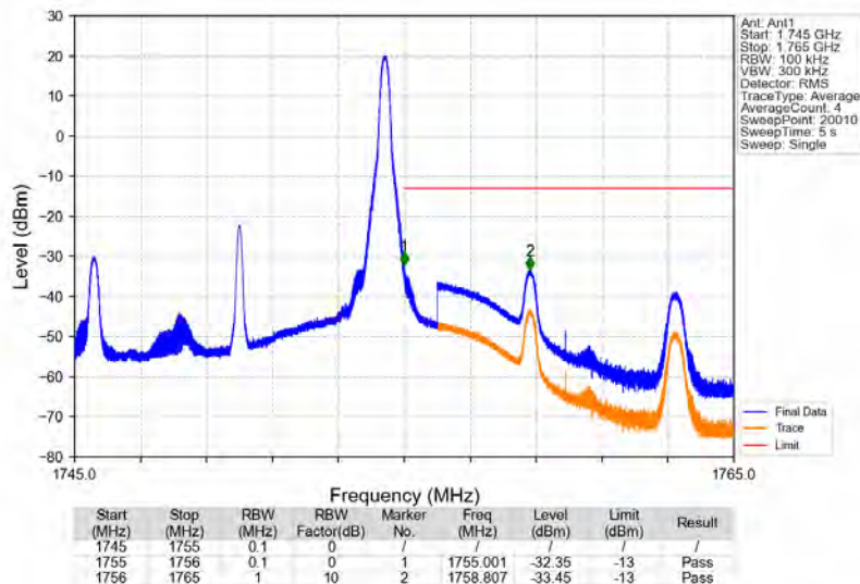
Band4_10MHz_QPSK_HCH_1750MHz_RB_1_49_NTNV
