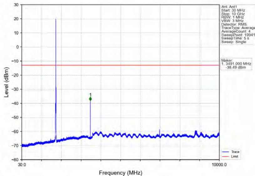
Band4 10MHz 64QAM HCH 1750MHz RB 1 0 NTNV
