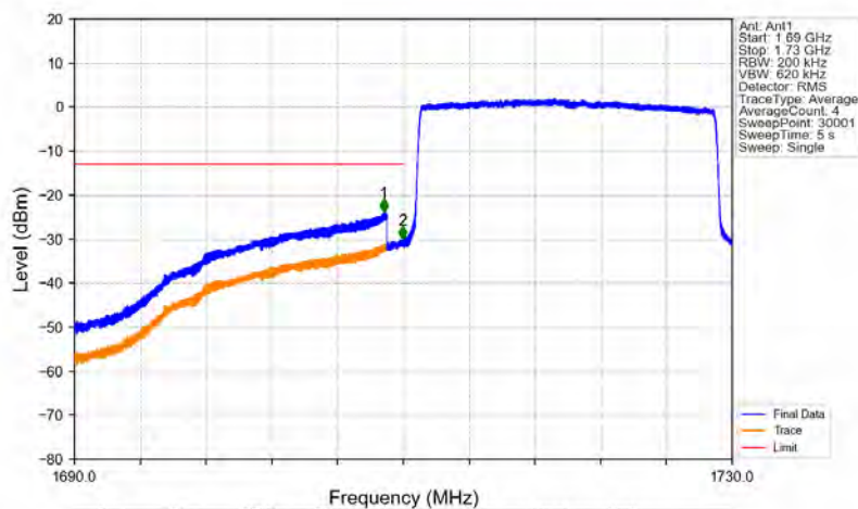
Band4_20MHz_16QAM_LCH_1720MHz_RB_100_0_NTNV
