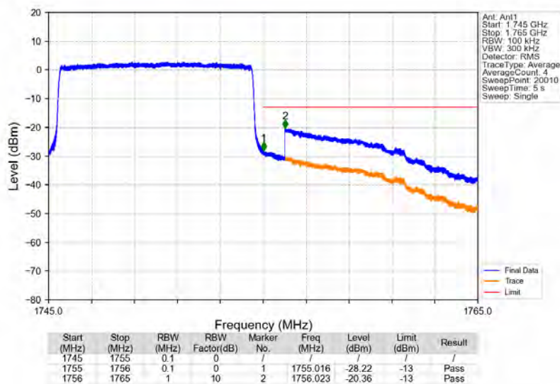
Band4_10MHz_QPSK_HCH_1750MHz_RB_50_0_NTNV
