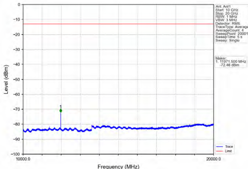
Band4 1.4MHz QPSK LCH 1710.7MHz RB 6 0 NTV
