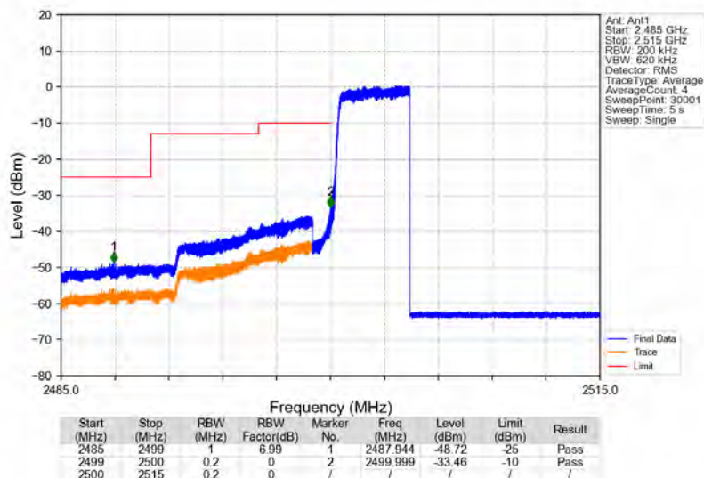
Band7_10MHz_QPSK_LCH_2505MHz_RB_50_0_NTNV
