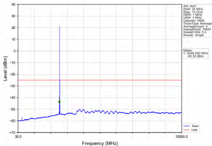
Band7_5MHz_QPSK_HCH_2567.5MHz_RB_1_0_NTNV
