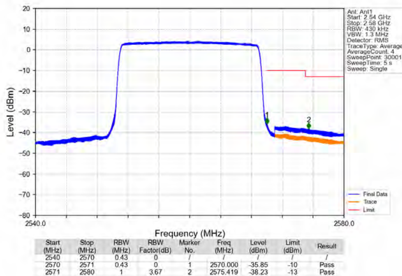
Band7_20MHz_16QAM_HCH_2560MHz_RB_100_0_NTNV
