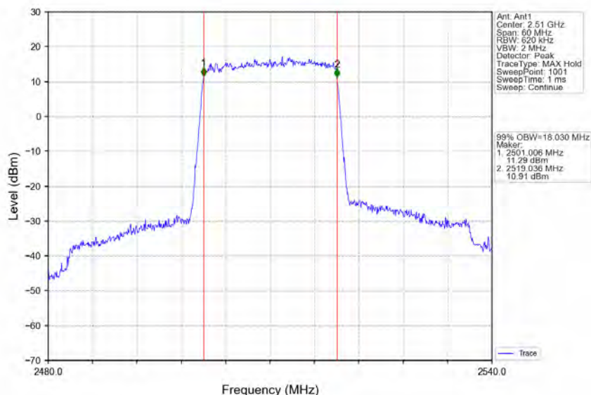
Band7_20MHz_QPSK_LCH_2510MHz_RB_100_0_NTNV
