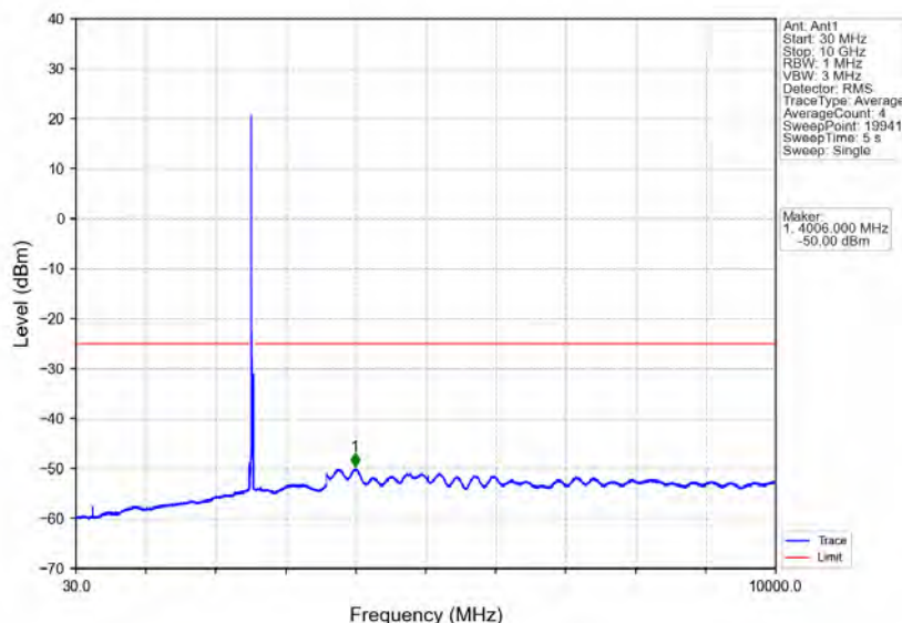
Band7_20MHz_QPSK_MCH_2535MHz_RB_1_0_NTNV
