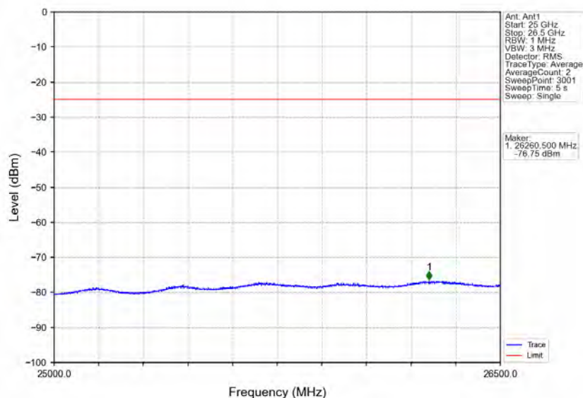
Band7_20MHz_64QAM_HCH_2560MHz_RB_1_99_NTNV
