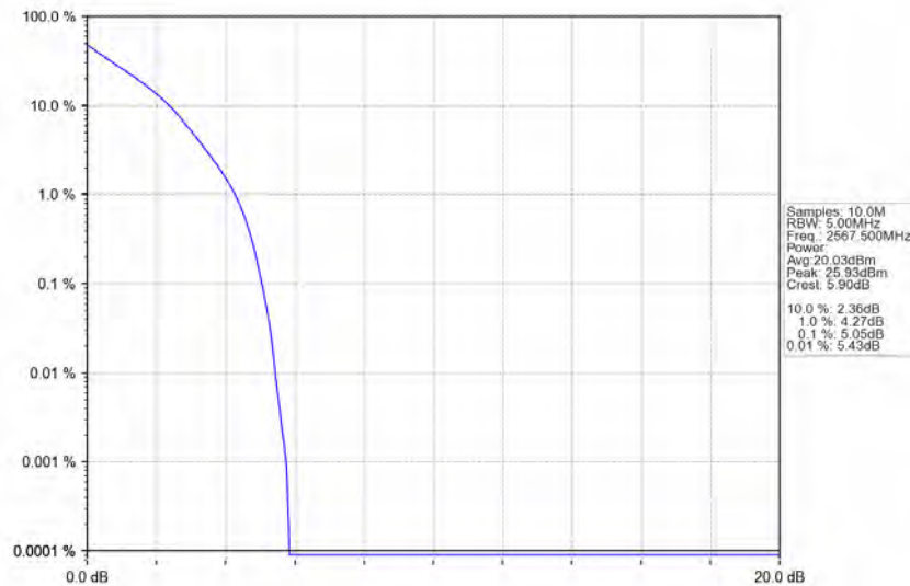
Band7_5MHz_QPSK_HCH_2567.5MHz_RB_25_0_NTNV
