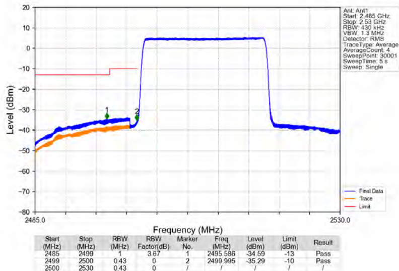
Band7_20MHz_64QAM_LCH_2510MHz_RB_100_0_NTNV
