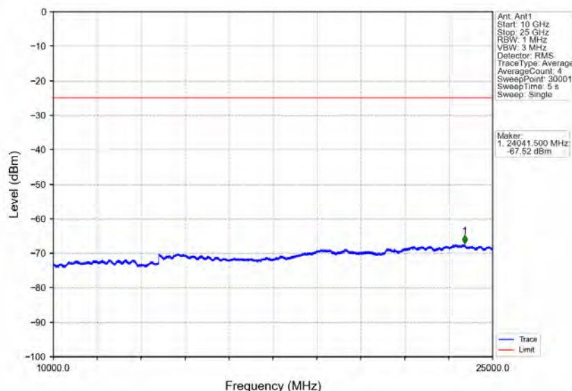
Band7_20MHz_16QAM_MCH_2535MHz_RB_1_0_NTNV
