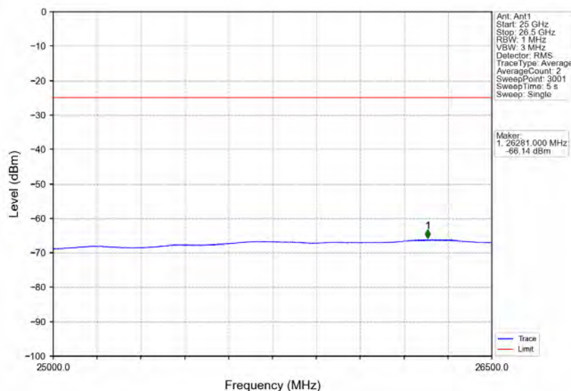
Band7_5MHz_QPSK_HCH_2567.5MHz_RB_1_24_NTNV
