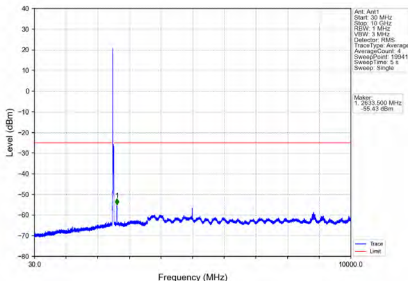
Band7 20MHz 64QAM LCH 2510MHz RB 1_0 NTNV
