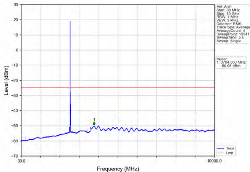
Band7_20MHz_16QAM_HCH_2560MHz_RB_1_0_NTNV
