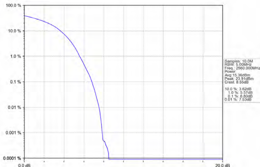
Band7_20MHz_QPSK_HCH_2560MHz_RB_100_0_NTNV
