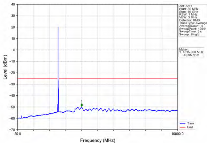
Band7_20MHz_QPSK_HCH_2560MHz_RB_1_0_NTNV
