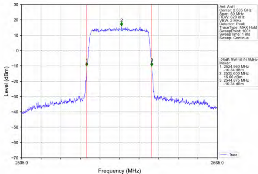
Band7_20MHz_16QAM_MCH_2535MHz_RB_100_0_NTNV
