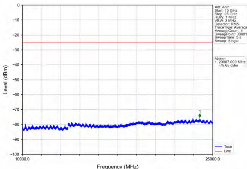
Band7_20MHz_64QAM_HCH_2560MHz_RB_1_0_NTNV
