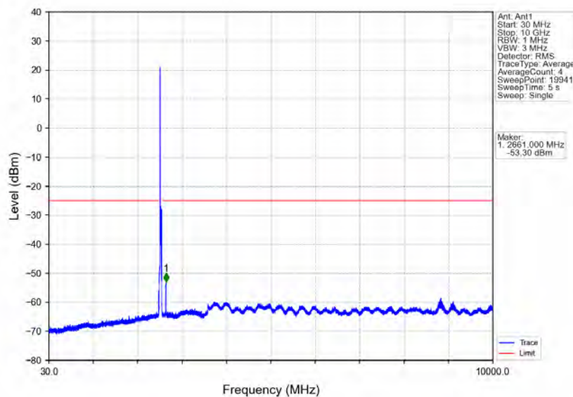
Band7_20MHz_64QAM_MCH_2535MHz_RB_1_0_NTNV
