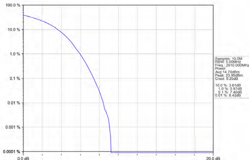
Band7_20MHz_16QAM_LCH_2510MHz_RB_100_0_NTNV
