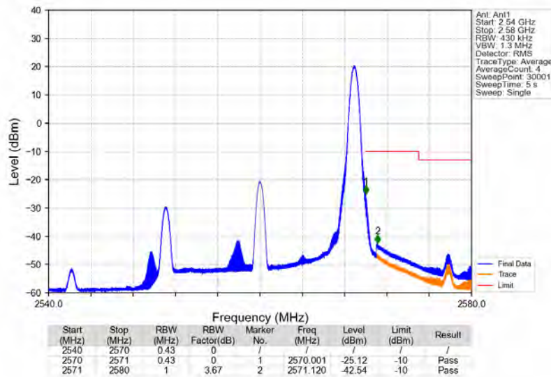
Band7_20MHz_16QAM_HCH_2560MHz_RB_1_99_NTNV
