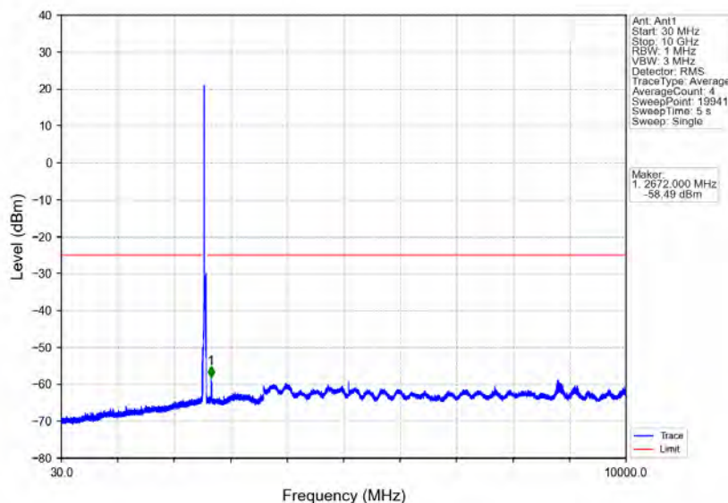
Band7_20MHz_64QAM_HCH_2560MHz_RB_1_0_NTNV
