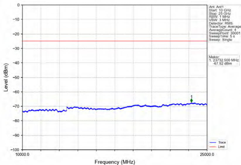
Band7_20MHz_QPSK_HCH_2560MHz_RB_1_0_NTNV
