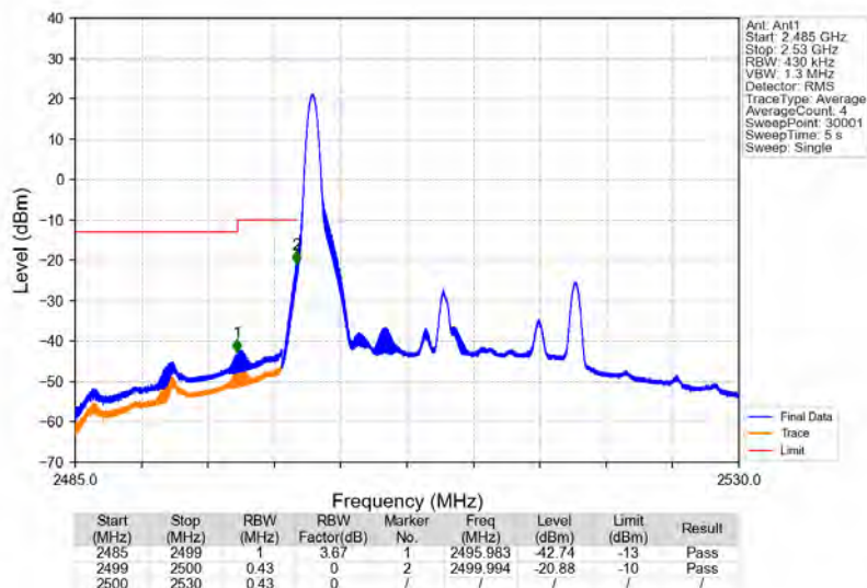
Band7 20MHz 64QAM LCH 2510MHz RB 1_0 NTNV
