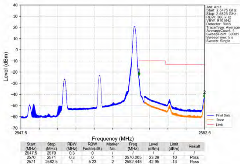
Band7_15MHz_QPSK_HCH_2562.5MHz_RB_1_74_NTNV
