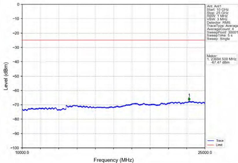
Band7_20MHz_16QAM_LCH_2510MHz_RB_1_0_NTNV
