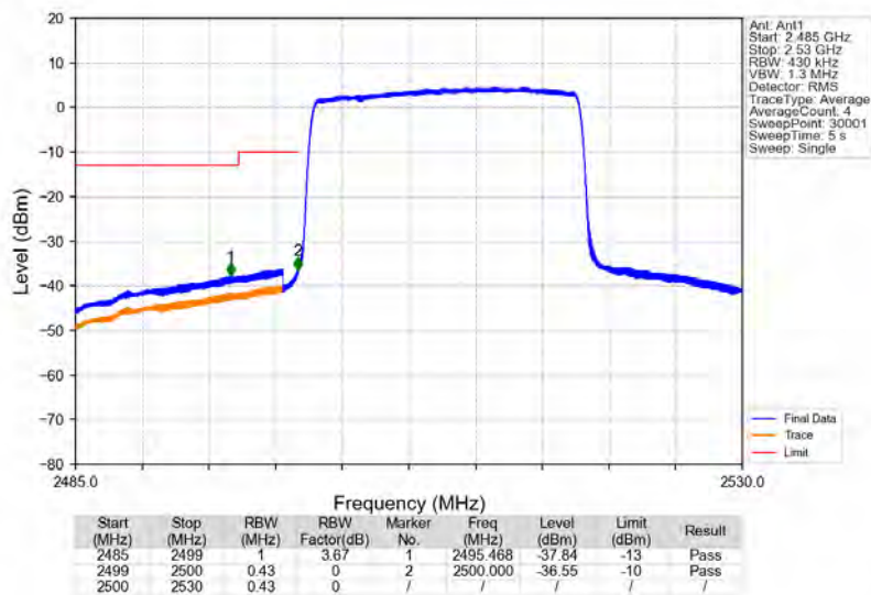
Band7_20MHz_16QAM_LCH_2510MHz_RB_100_0_NTNV
