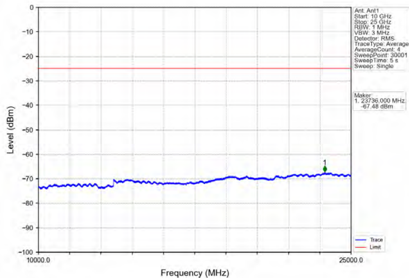
Band7_20MHz_16QAM_HCH_2560MHz_RB_1_0_NTNV
