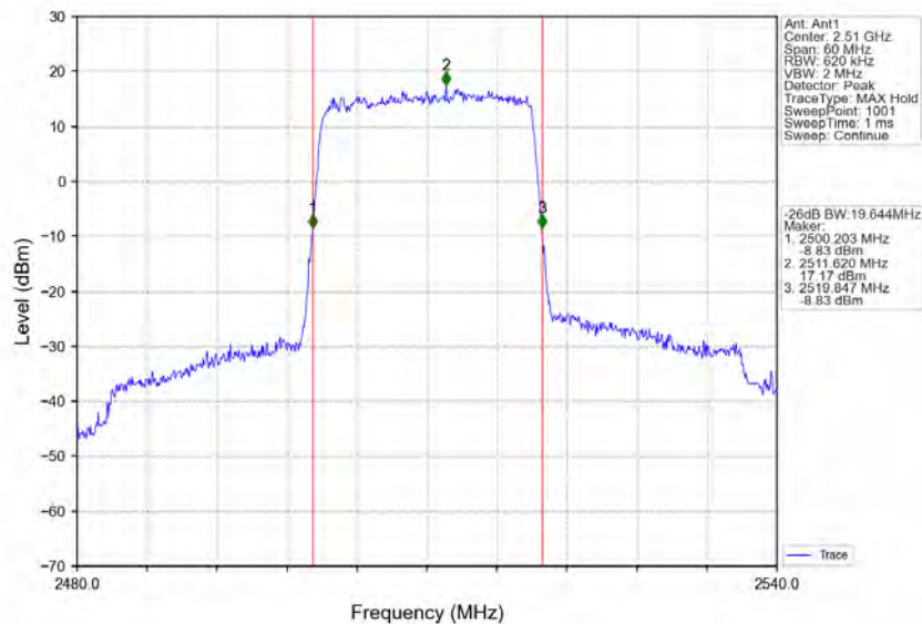
Band7_20MHz_QPSK_LCH_2510MHz_RB_100_0_NTNV
