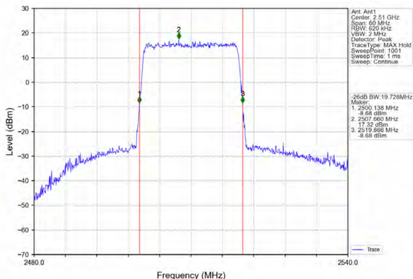
Band7_20MHz_64QAM_LCH_2510MHz_RB_100_0_NTNV
