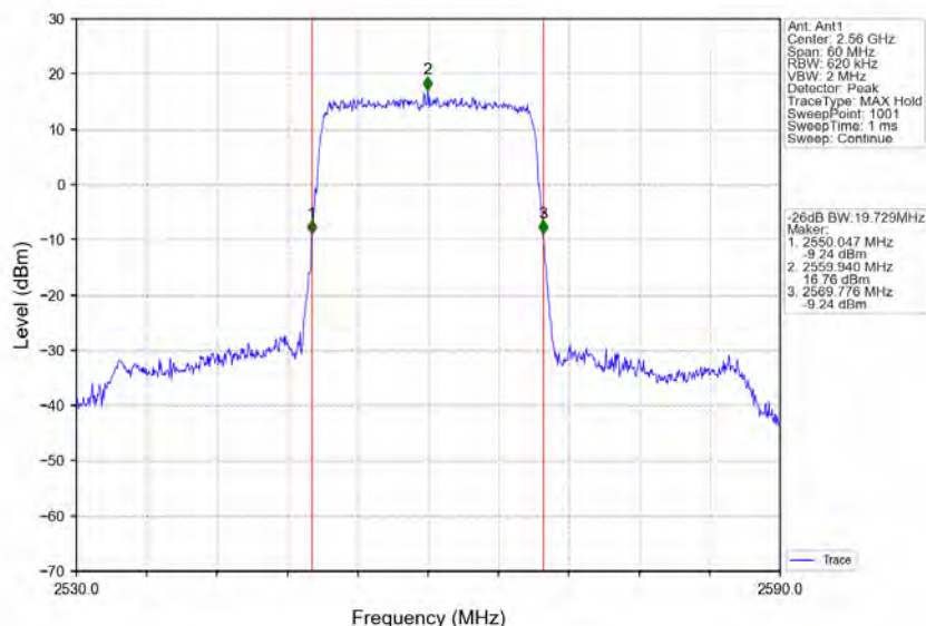
Band7_20MHz_QPSK_HCH_2560MHz_RB_100_0_NTNV
