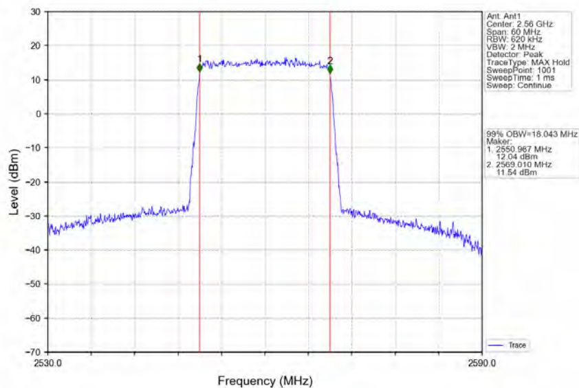
Band7 20MHz 64QAM HCH 2560MHz RB 100 0 NTN
