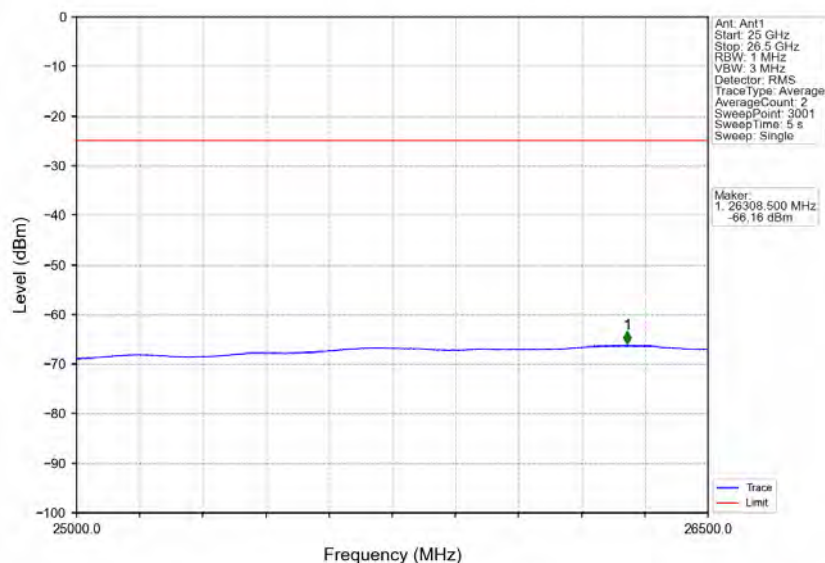
Band7_20MHz_QPSK_HCH_2560MHz_RB_1_99_NTNV
