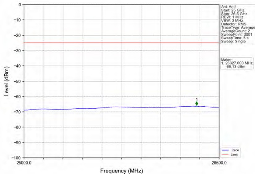
Band7_20MHz_16QAM_HCH_2560MHz_RB_1_0_NTNV
