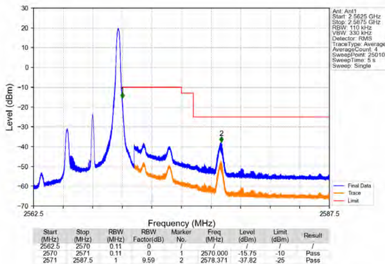
Band7_5MHz_QPSK_HCH_2567.5MHz_RB_1_24_NTNV
