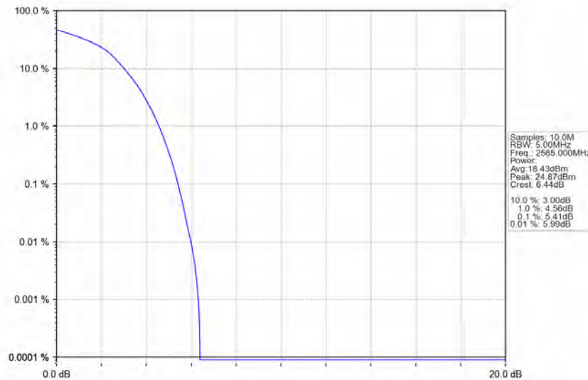
Band7_10MHz_QPSK_HCH_2565MHz_RB_50_0_NTNV
