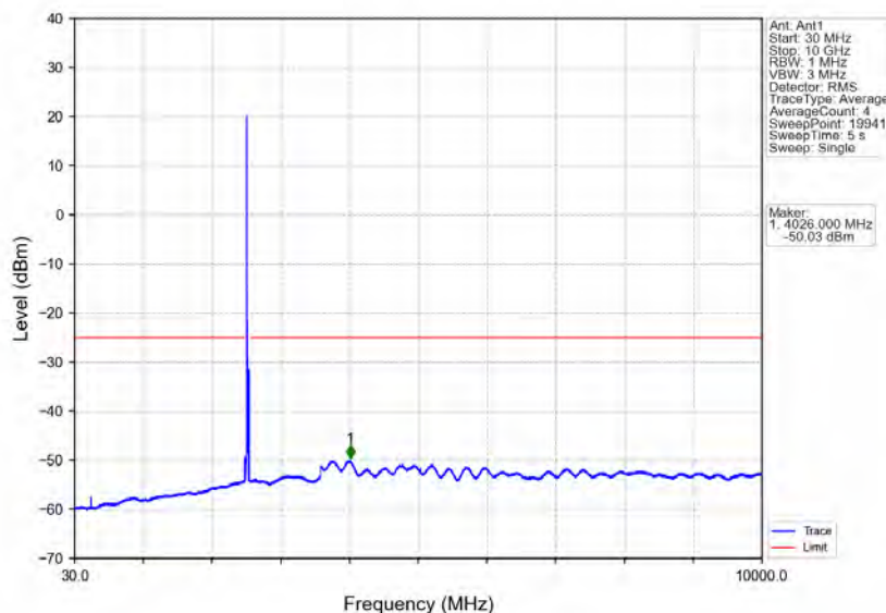
Band7_20MHz_16QAM_MCH_2535MHz_RB_1_0_NTNV
