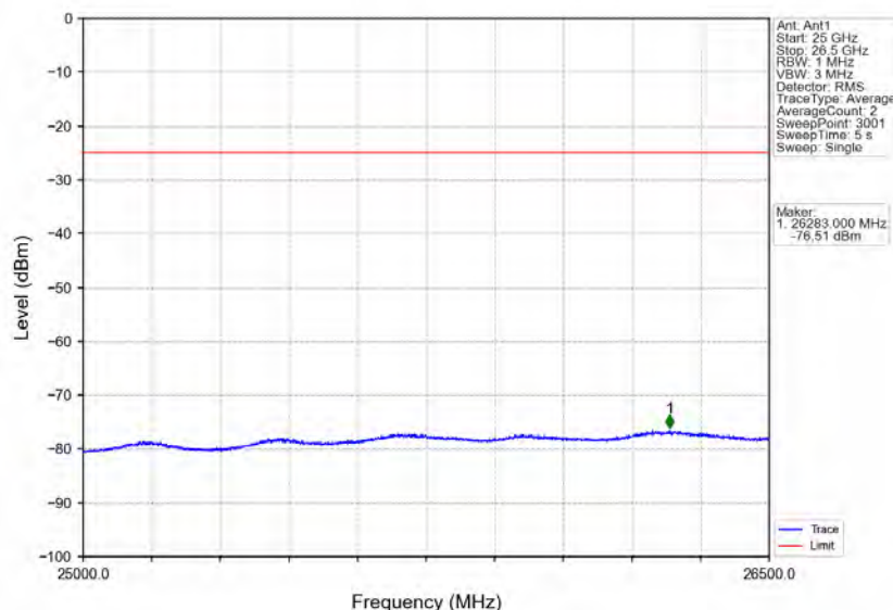
Band7_20MHz_64QAM_LCH_2510MHz_RB_1_0_NTNV
