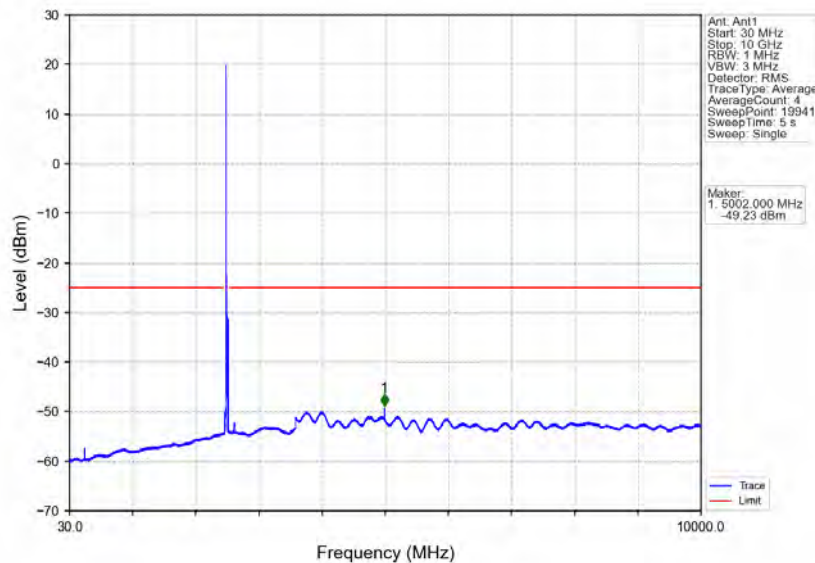
Band7_20MHz_16QAM_LCH_2510MHz_RB_1_0_NTNV
