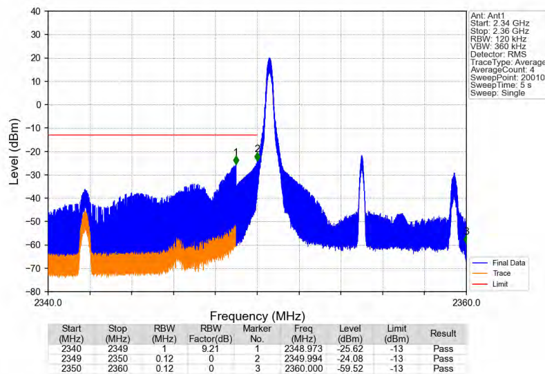
Band40b_10MHz_16QAM_LCH_2355MHz_RB_1_0_NTNV
