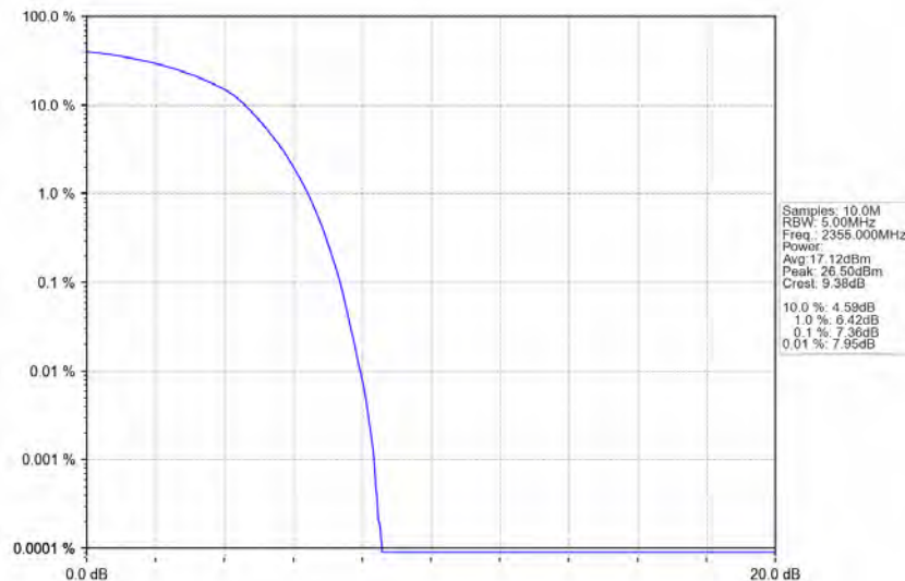
Band40b_10MHz_QPSK_HCH_2355MHz_RB_50_0_NTNV
