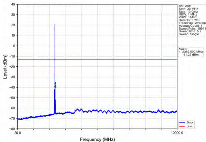
Band40b_10MHz_QPSK_MCH_2355MHz_RB_1_0_NTNV
