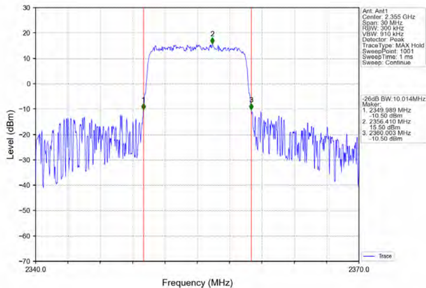
Band40b_10MHz_16QAM_MCH_2355MHz_RB_50_0_NTNV
