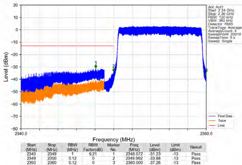
Band40b_10MHz_16QAM_LCH_2355MHz_RB_50_0_NTNV
