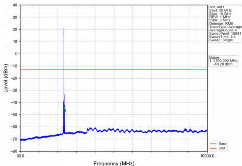
Band40b_10MHz_QPSK_HCH_2355MHz_RB_1_0_NTNV
