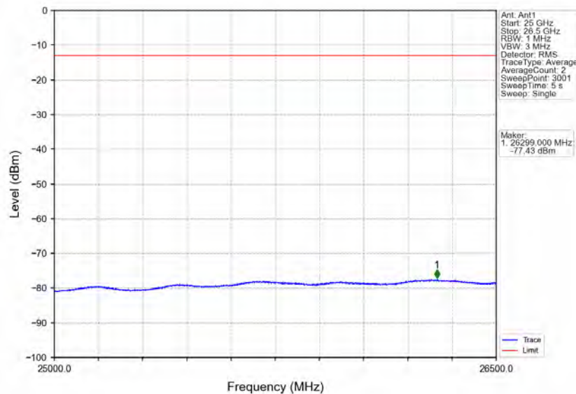
Band40b_10MHz_QPSK_MCH_2355MHz_RB_1_0_NTNV
