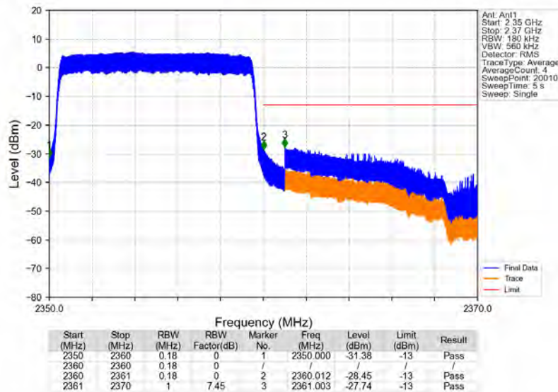
Band40b_10MHz_QPSK_HCH_2355MHz_RB_50_0_NTNV
