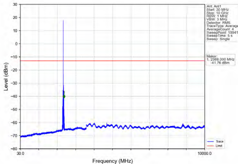
Band40b_10MHz_16QAM_LCH_2355MHz_RB_1_0_NTNV
