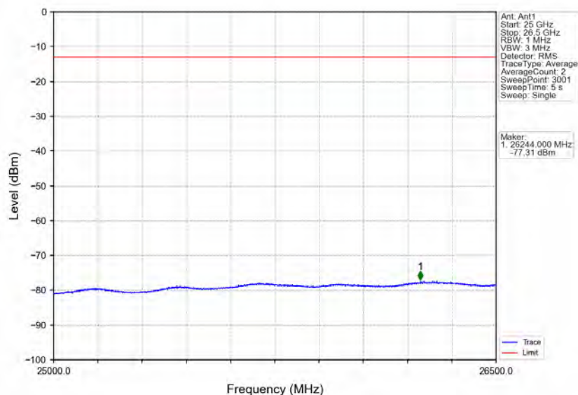
Band40b_10MHz_QPSK_HCH_2355MHz_RB_1_49_NTNV
