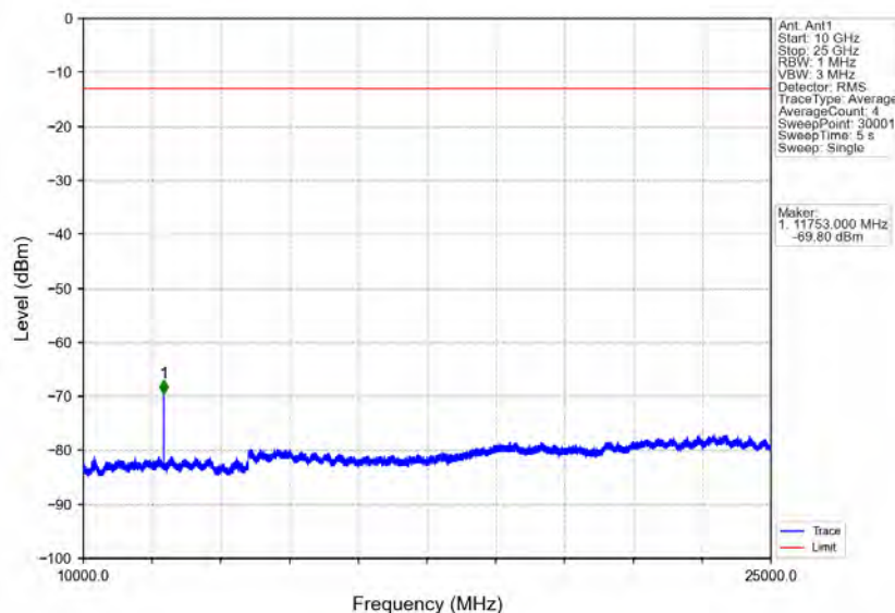
Band40b_10MHz_QPSK_LCH_2355MHz_RB_1_0_NTNV
