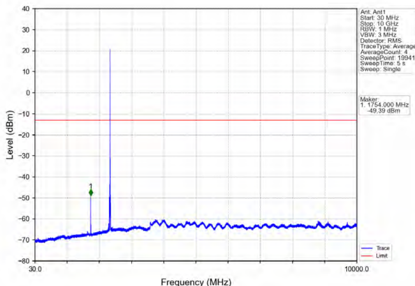
Band40b_5MHz_QPSK_MCH_2355MHz_RB_1_0_NTNV
