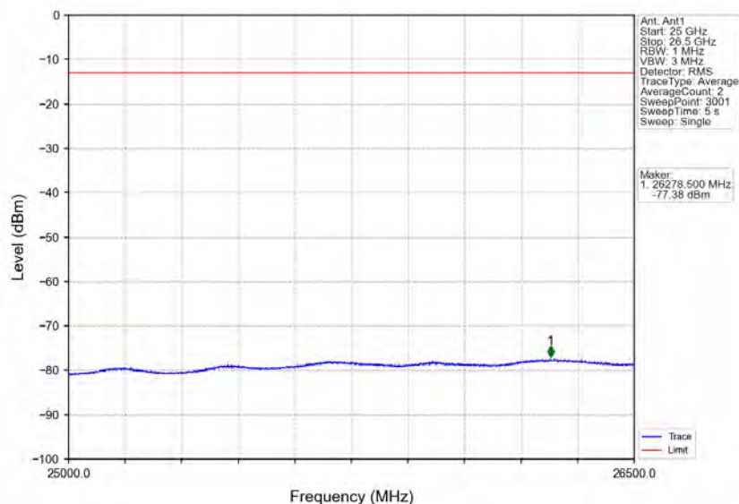
Band40b_10MHz_16QAM_LCH_2355MHz_RB_50_0_NTNV
