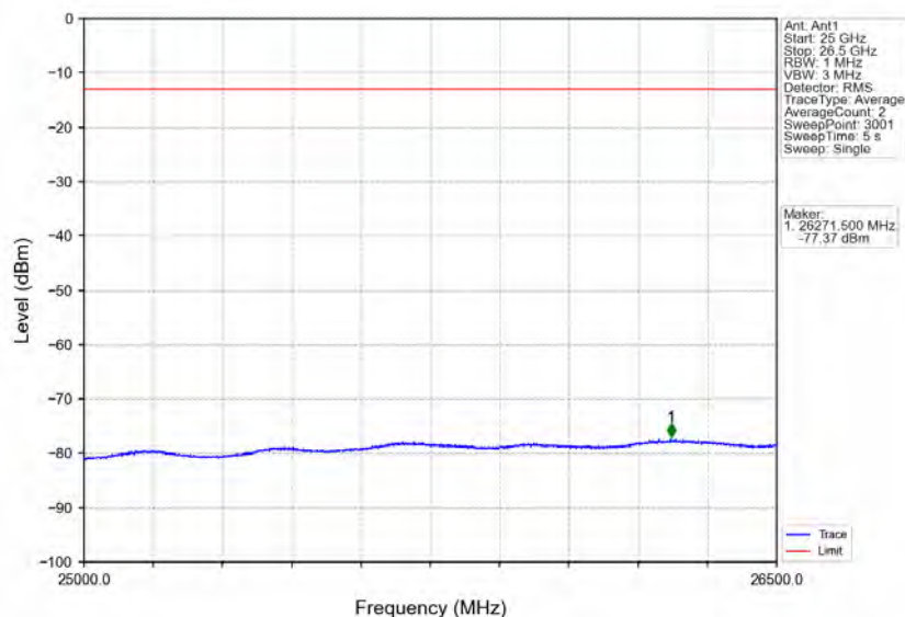
Band40b_5MHz_QPSK_HCH_2357.5MHz_RB_1_24_NTNV
