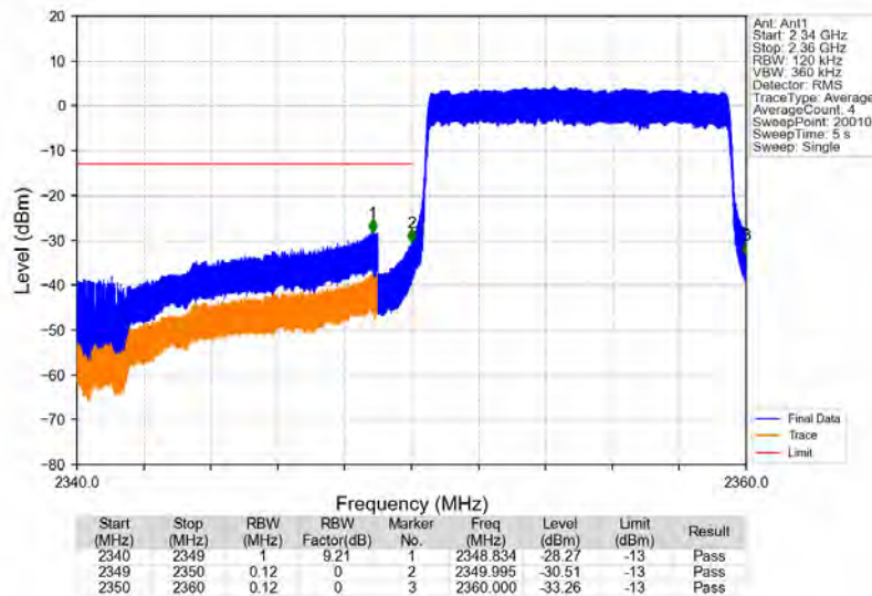
Band40b_10MHz_QPSK_LCH_2355MHz_RB_50_0_NTNV
