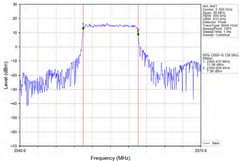
Band40b_10MHz_QPSK_HCH_2355MHz_RB_50_0_NTNV
