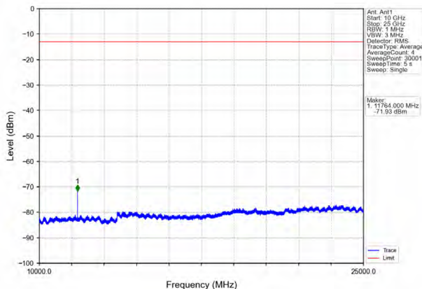
Band40b_5MHz_QPSK_MCH_2355MHz_RB_1_0_NTNV
