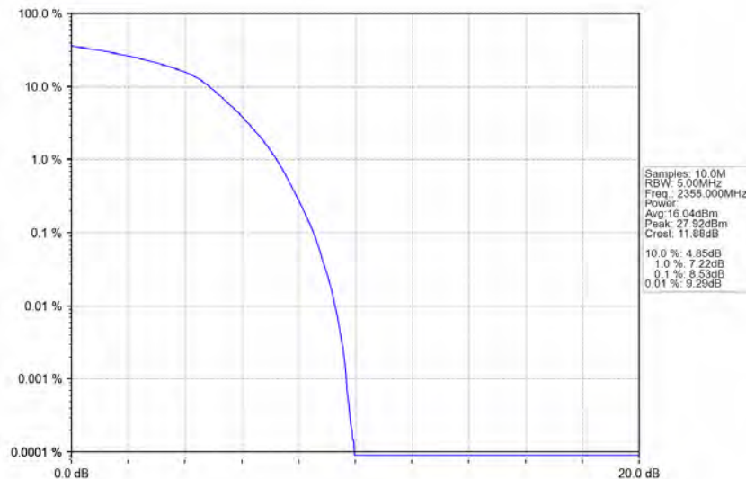
Band40b_10MHz_16QAM_LCH_2355MHz_RB_50_0_NTNV
