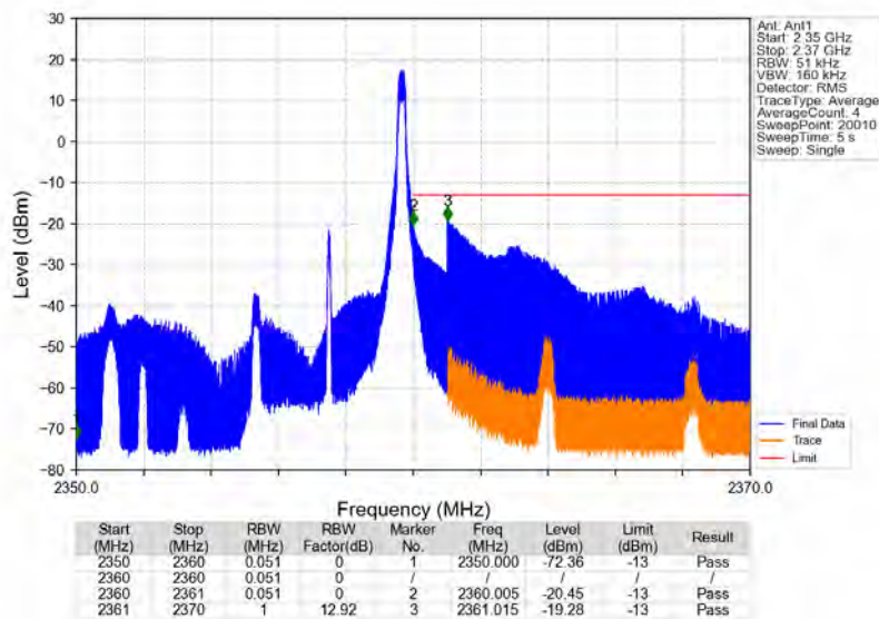
Band40b_5MHz_QPSK_HCH_2357.5MHz_RB_1_24_NTNV
