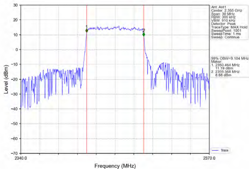
Band40b_10MHz_16QAM_MCH_2355MHz_RB_50_0_NTNV
