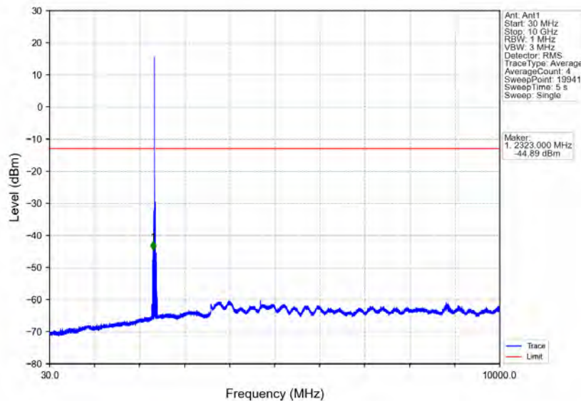
Band40b_10MHz_16QAM_MCH_2355MHz_RB_1_0_NTNV
