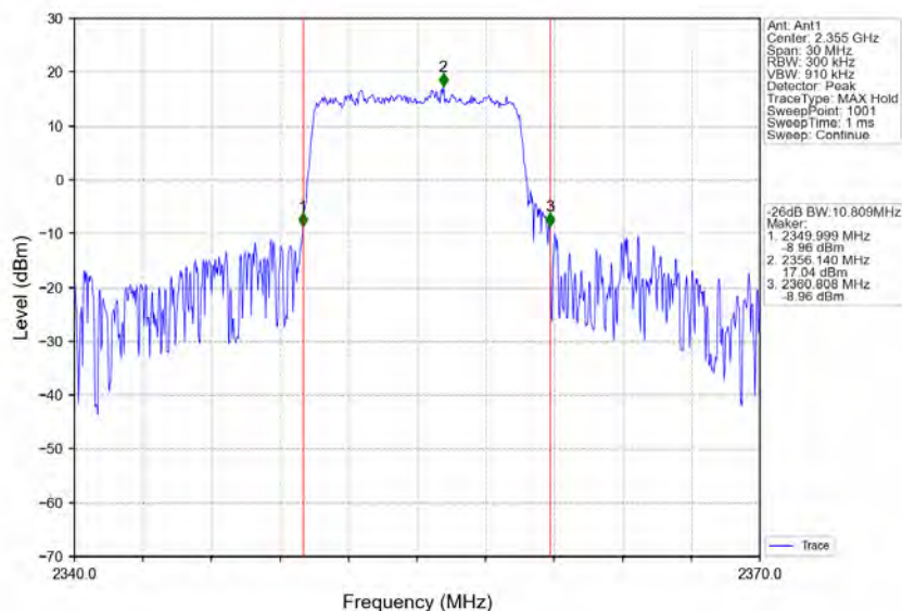
Band40b_10MHz_QPSK_HCH_2355MHz_RB_50_0_NTNV
