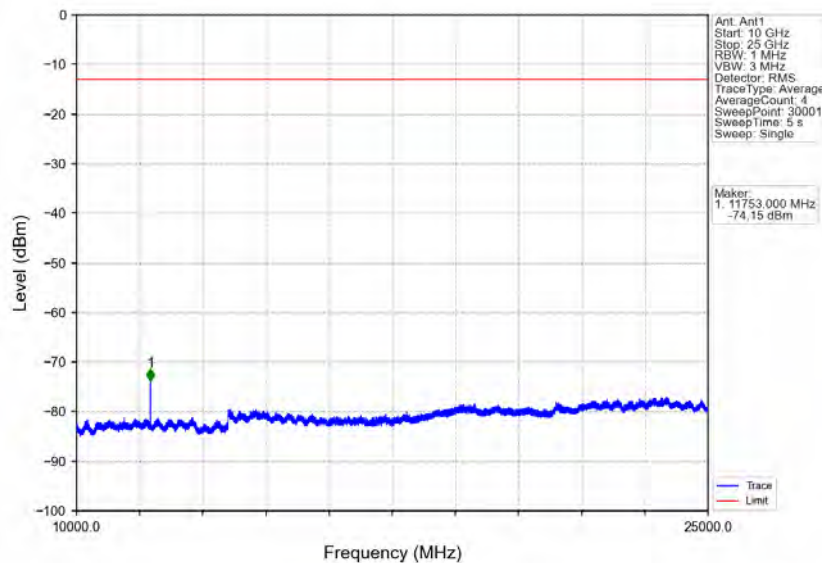
Band40b_10MHz_16QAM_MCH_2355MHz_RB_1_0_NTNV
