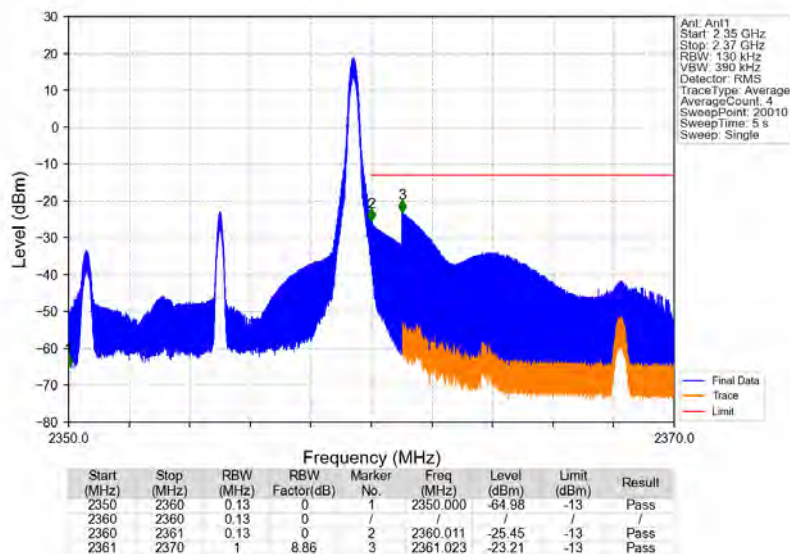
Band40b_10MHz_16QAM_HCH_2355MHz_RB_1_49_NTNV
