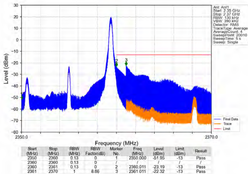
Band40b_10MHz_QPSK_HCH_2355MHz_RB_1_49_NTNV
