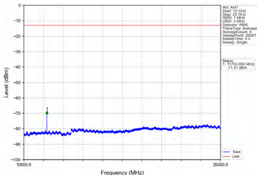
Band40b_10MHz_QPSK_HCH_2355MHz_RB_1_0_NTNV
