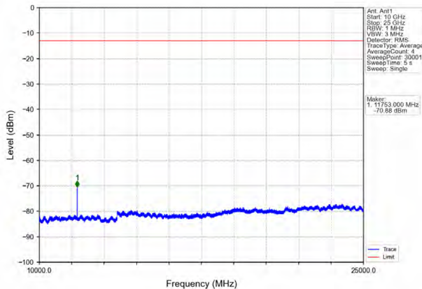
Band40b_10MHz_16QAM_LCH_2355MHz_RB_1_0_NTNV
