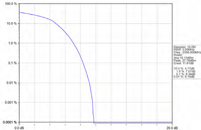
Band40b_10MHz_16QAM_MCH_2355MHz_RB_50_0_NTNV
