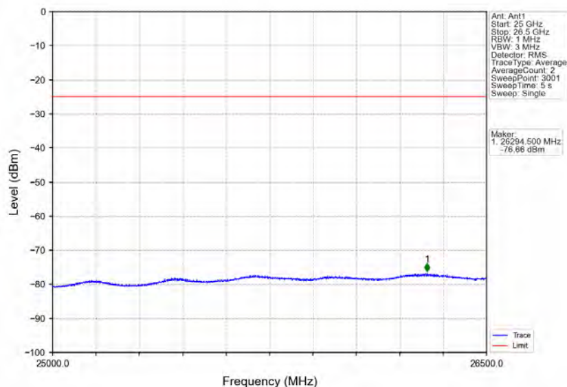
Band41_10MHz_64QAM_HCH_2685MHz_RB_1_49_NTNV
