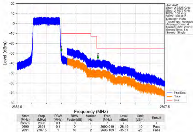
Band41_5MHz_QPSK_HCH_2687.5MHz_RB_25_0_NTNV
