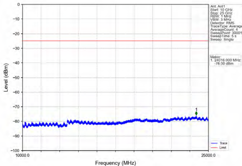
Band41_10MHz_16QAM_MCH_2593MHz_RB_1_0_NTNV
