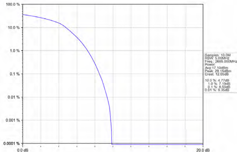
Band41_10MHz_16QAM_HCH_2685MHz_RB_50_0_NTNV
