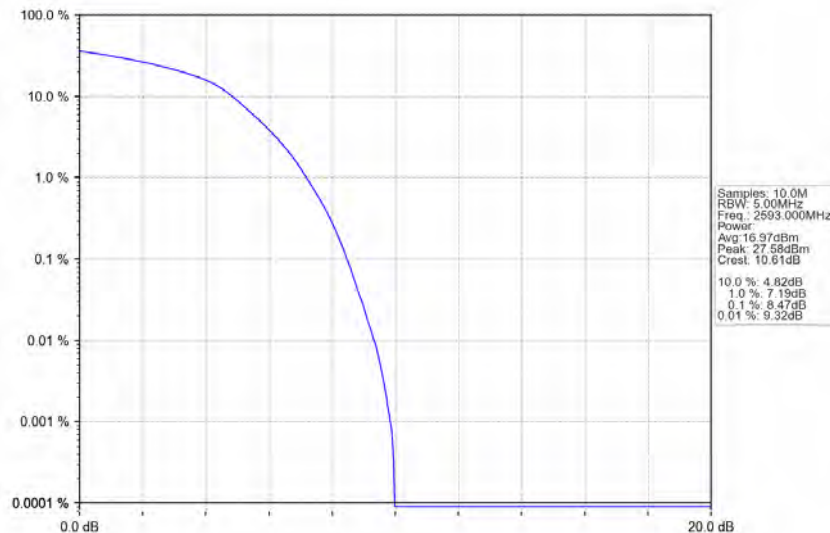
Band41_10MHz_16QAM_MCH_2593MHz_RB_50_0_NTNV
