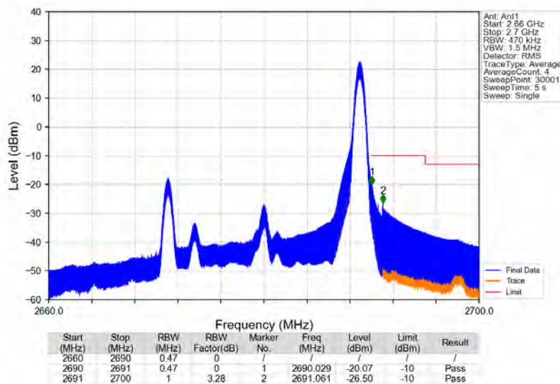
Band41_20MHz_QPSK_HCH_2680MHz_RB_1_99_NTNV
