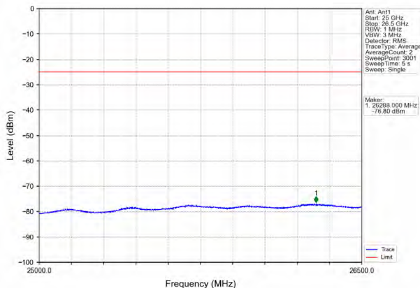
Band41_10MHz_QPSK_HCH_2685MHz_RB_1_49_NTNV
