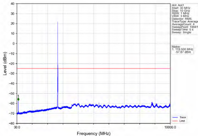
Band41_10MHz_QPSK_HCH_2685MHz_RB_1_0_NTNV
