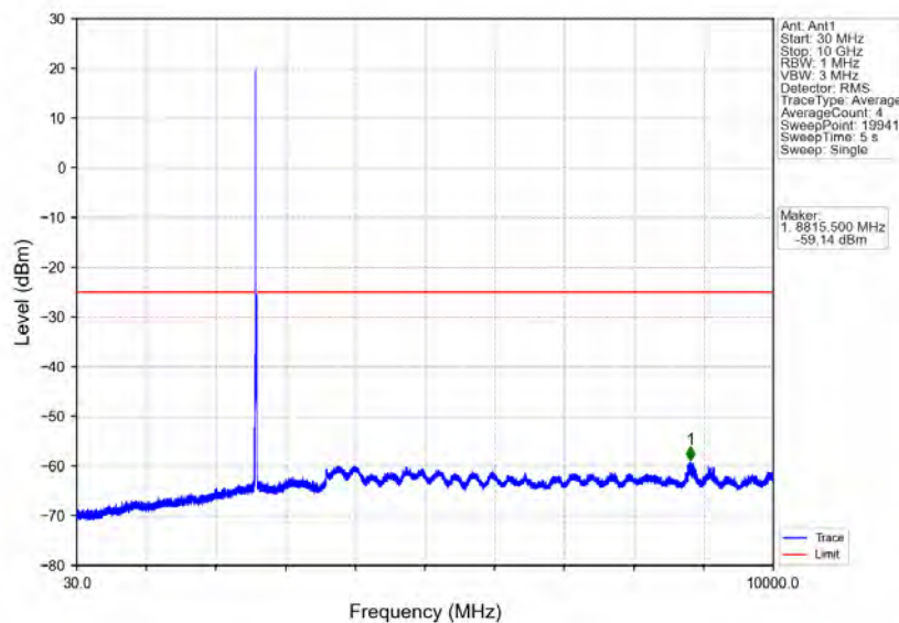
Band41_10MHz_QPSK_MCH_2593MHz_RB_1_0_NTNV
