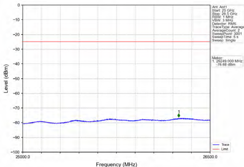
Band41_20MHz_QPSK_HCH_2680MHz_RB_1_99_NTNV
