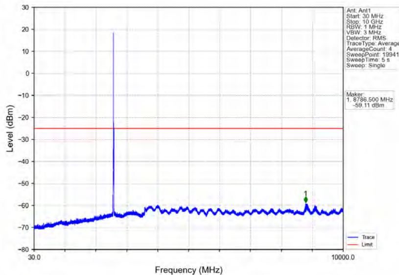
Band41_10MHz_16QAM_MCH_2593MHz_RB_1_0_NTNV
