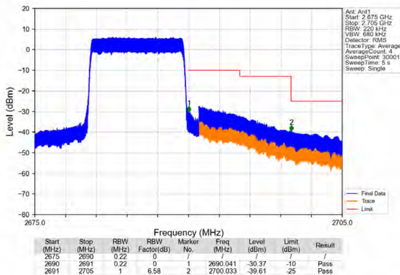
Band41_10MHz_16QAM_HCH_2685MHz_RB_50_0_NTNV
