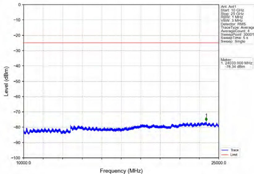
Band41_10MHz_QPSK_HCH_2685MHz_RB_1_0_NTNV
