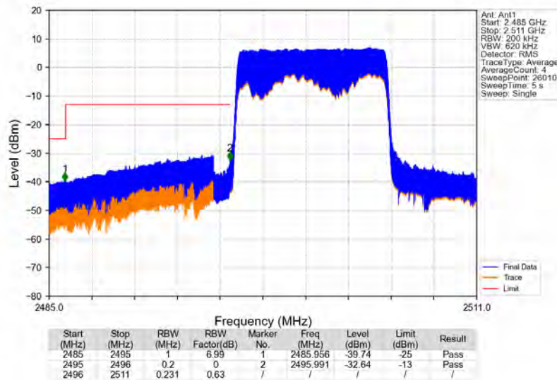
Band41_10MHz_16QAM_LCH_2501MHz_RB_50_0_NTNV
