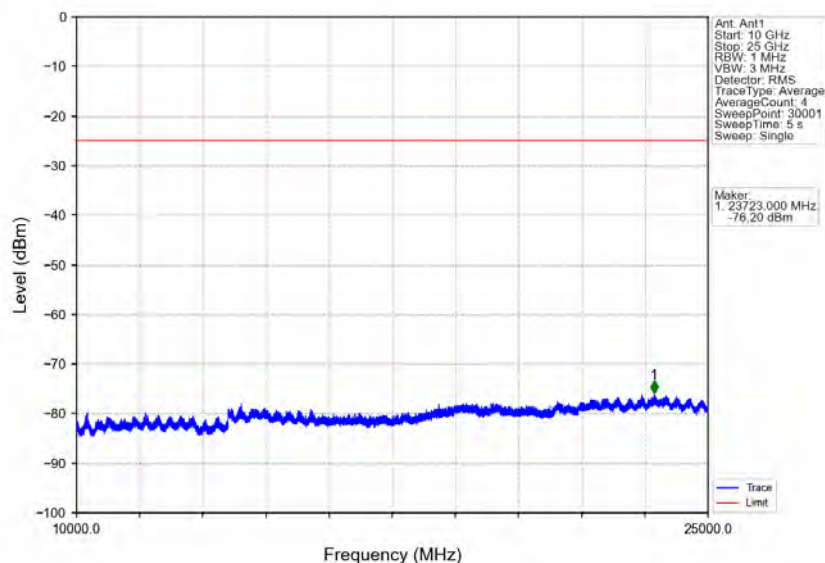
Band41_20MHz_QPSK_MCH_2593MHz_RB_1_0_NTNV
