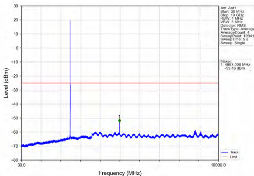
Band41_5MHz_QPSK_LCH_2498.5MHz_RB_1_0_NTNV
