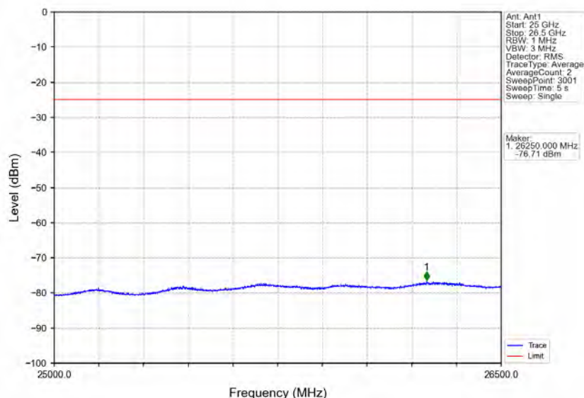
Band41_10MHz_16QAM_HCH_2685MHz_RB_1_0_NTNV
