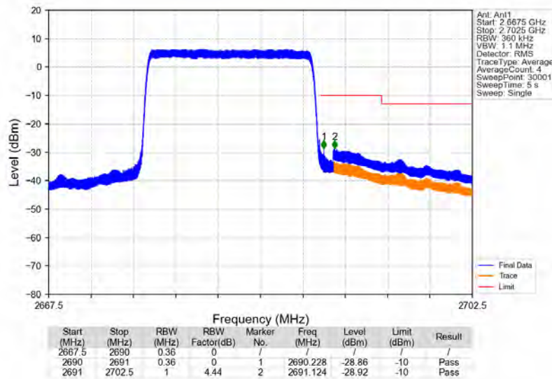
Band41_15MHz_QPSK_HCH_2682.5MHz_RB_75_0_NTNV
