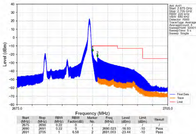
Band41_10MHz_QPSK_HCH_2685MHz_RB_1_49_NTNV
