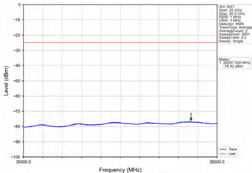
Band41_10MHz_QPSK_LCH_2501MHz_RB_1_0_NTNV
