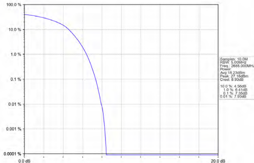
Band41_10MHz_QPSK_HCH_2685MHz_RB_50_0_NTNV
