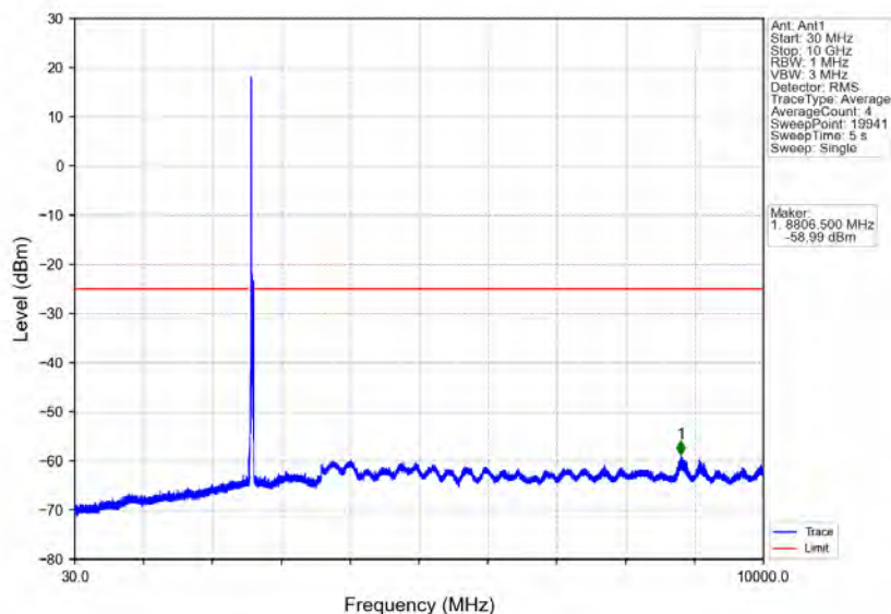
Band41_20MHz_16QAM_MCH_2593MHz_RB_1_0_NTNV
