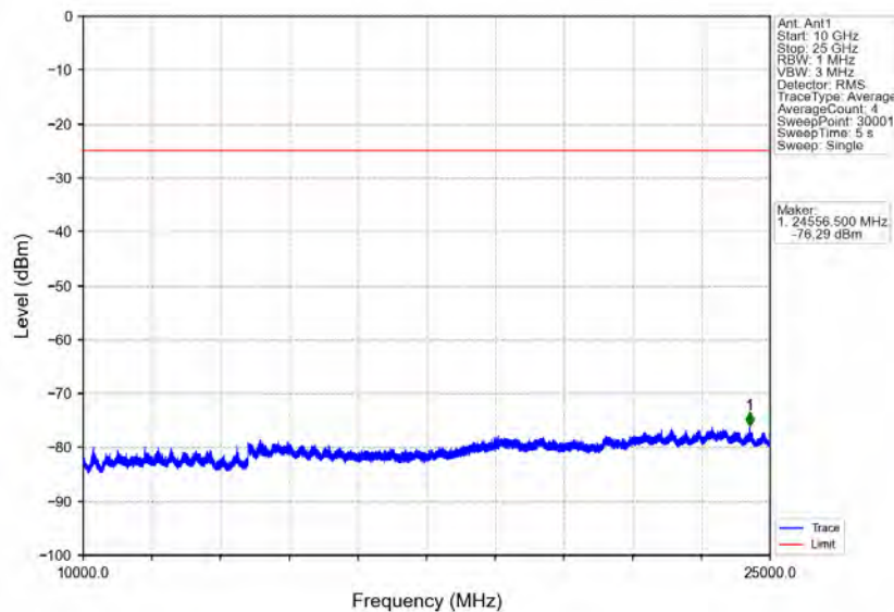
Band41_5MHz_QPSK_HCH_2687.5MHz_RB_1_0_NTNV
