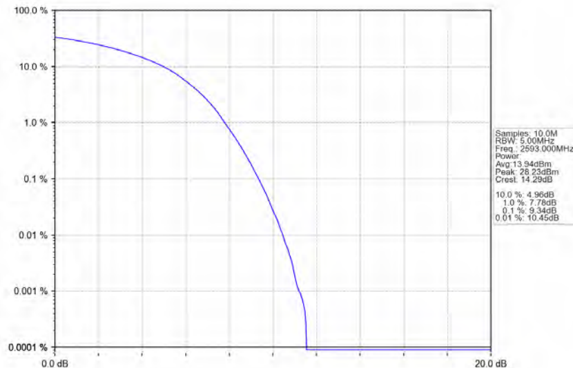
Band41_20MHz_16QAM_MCH_2593MHz_RB_100_0_NTNV
