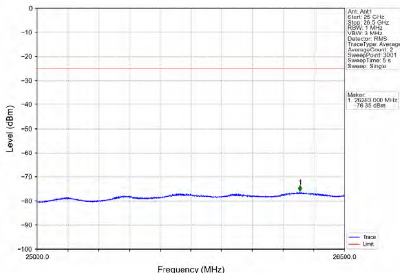
Band41_15MHz_QPSK_LCH_2503.5MHz_RB_1_0_NTNV
