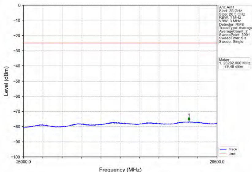
Band41_20MHz_QPSK_LCH_2506MHz_RB_1_0_NTNV
