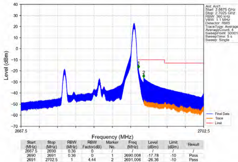
Band41_15MHz_QPSK_HCH_2682.5MHz_RB_1_74_NTNV
