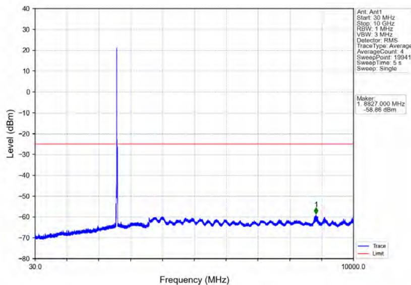
Band41_15MHz_QPSK_MCH_2593MHz_RB_1_0_NTNV
