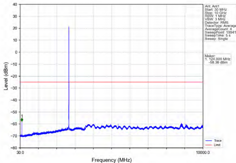
Band41_5MHz_QPSK_HCH_2687.5MHz_RB_1_0_NTNV
