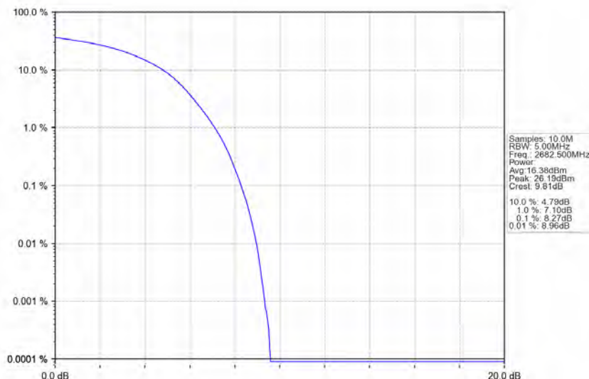
Band41_15MHz_QPSK_HCH_2682.5MHz_RB_75_0_NTNV
