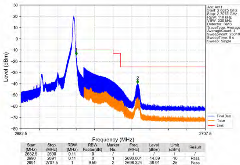
Band41_5MHz_QPSK_HCH_2687.5MHz_RB_1_24_NTNV
