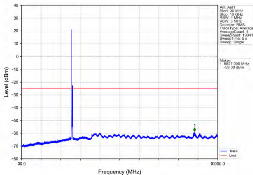
Band41_20MHz_QPSK_MCH_2593MHz_RB_1_0_NTNV
