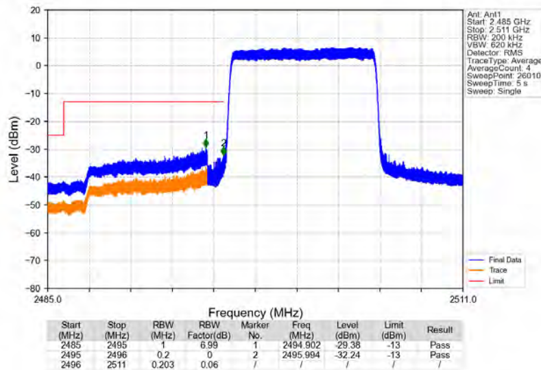
Band41_10MHz_QPSK_LCH_2501MHz_RB_50_0_NTNV
