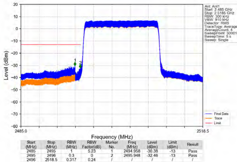
Band41_15MHz_QPSK_LCH_2503.5MHz_RB_75_0_NTNV
