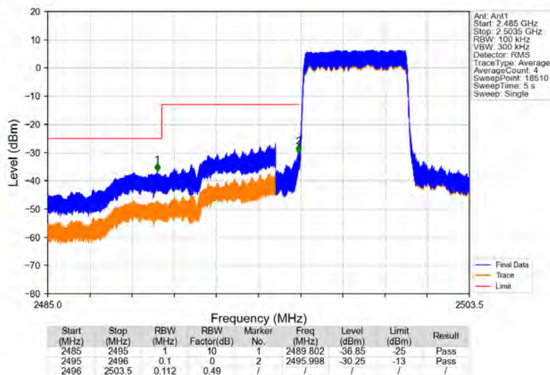
Band41_5MHz_QPSK_LCH_2498.5MHz_RB_25_0_NTNV
