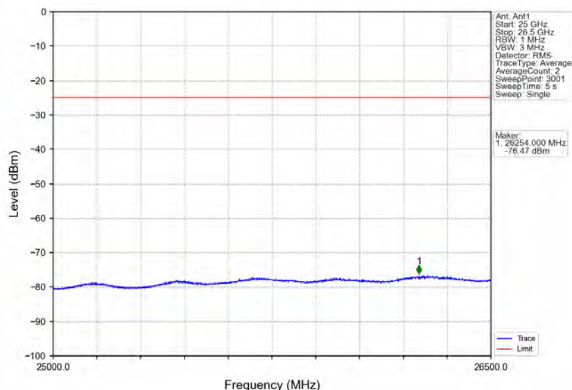
Band41_10MHz_QPSK_MCH_2593MHz_RB_1_0_NTNV
