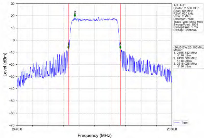
Band41_20MHz_QPSK_LCH_2506MHz_RB_100_0_NTNV
