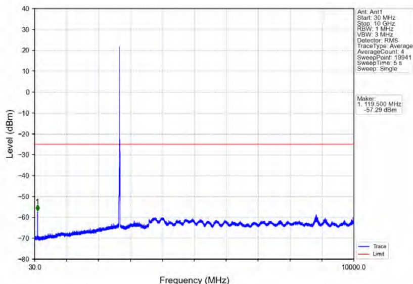
Band41_10MHz_16QAM_HCH_2685MHz_RB_1_0_NTNV
