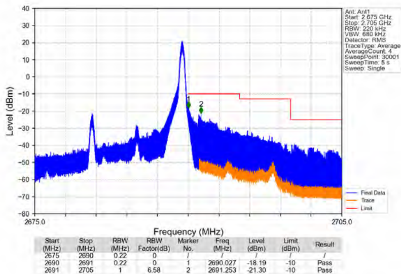
Band41_10MHz_64QAM_HCH_2685MHz_RB_1_49_NTNV
