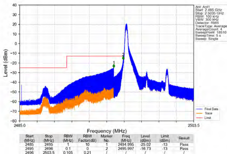
Band41_5MHz_QPSK_LCH_2498.5MHz_RB_1_0_NTNV
