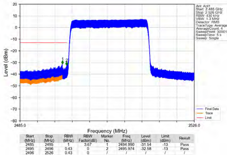
Band41_20MHz_QPSK_LCH_2506MHz_RB_100_0_NTNV
