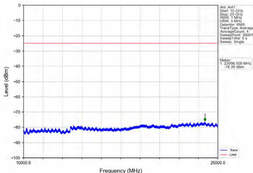
Band41_20MHz_QPSK_HCH_2680MHz_RB_1_0_NTNV
