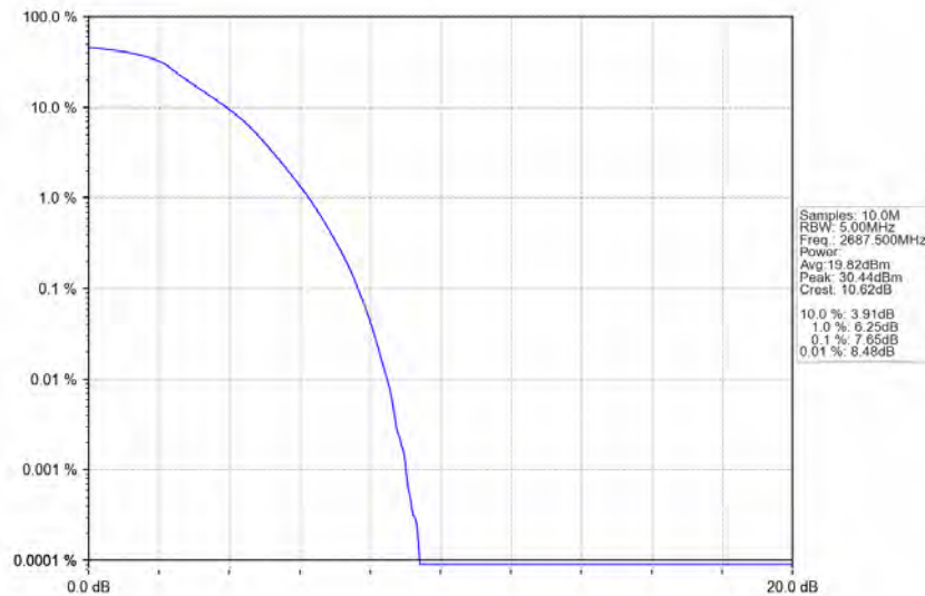
Band41_5MHz_QPSK_HCH_2687.5MHz_RB_25_0_NTNV
