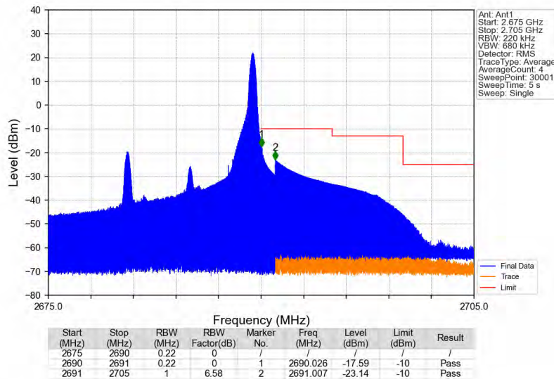
Band41_10MHz_16QAM_HCH_2685MHz_RB_1_49_NTNV
