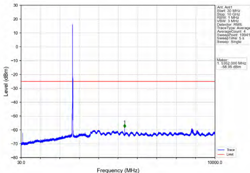
Band41_15MHz_QPSK_HCH_2682.5MHz_RB_1_0_NTNV
