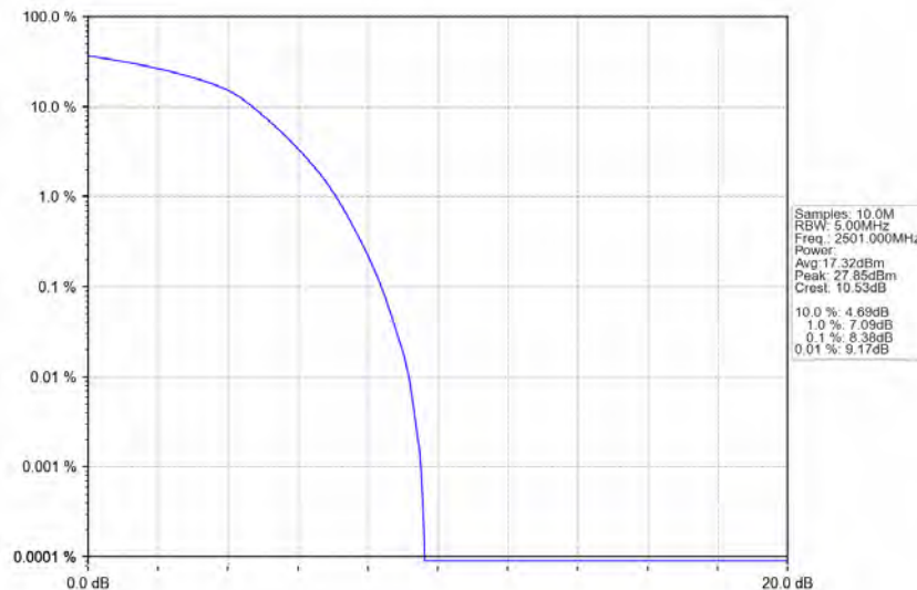
Band41_10MHz_16QAM_LCH_2501MHz_RB_50_0_NTNV
