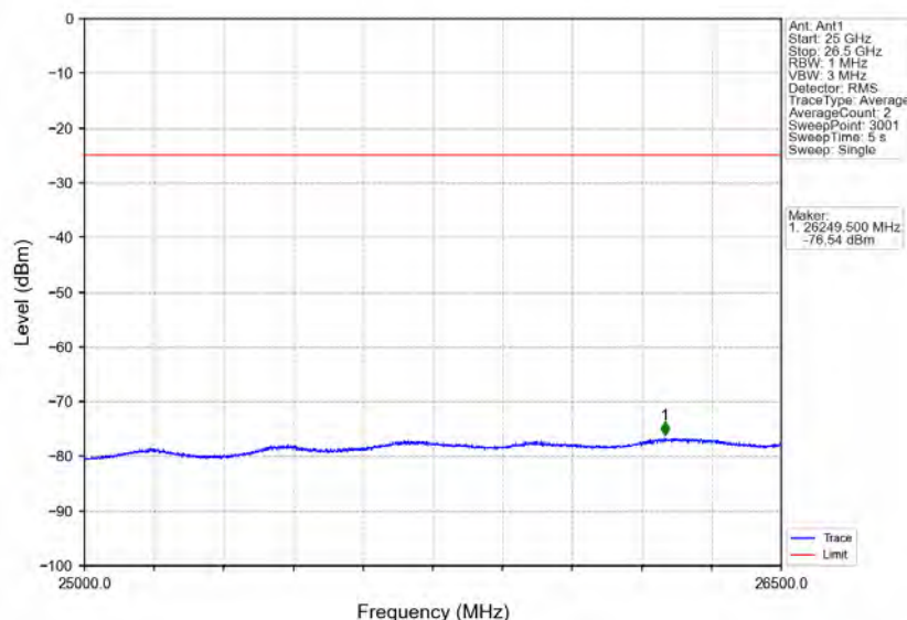
Band41_5MHz_QPSK_LCH_2498.5MHz_RB_1_0_NTNV
