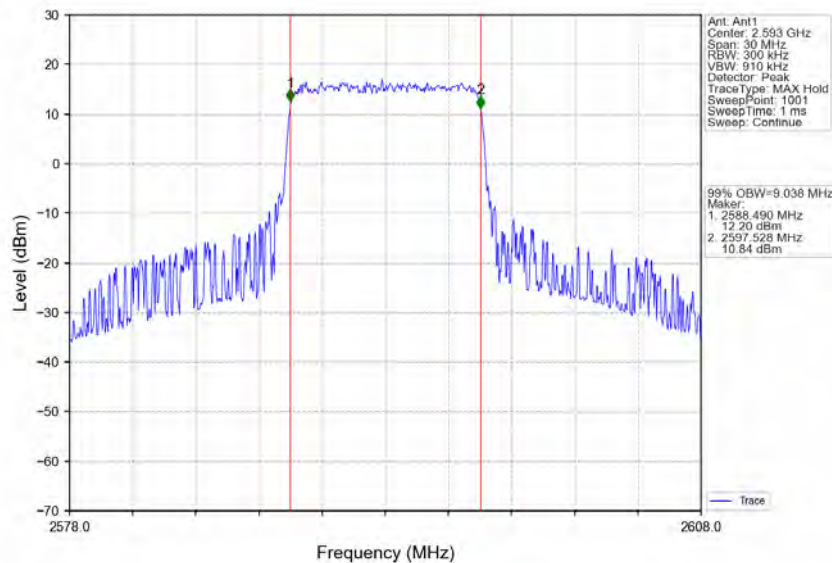
Band41_10MHz_16QAM_MCH_2593MHz_RB_50_0_NTNV
