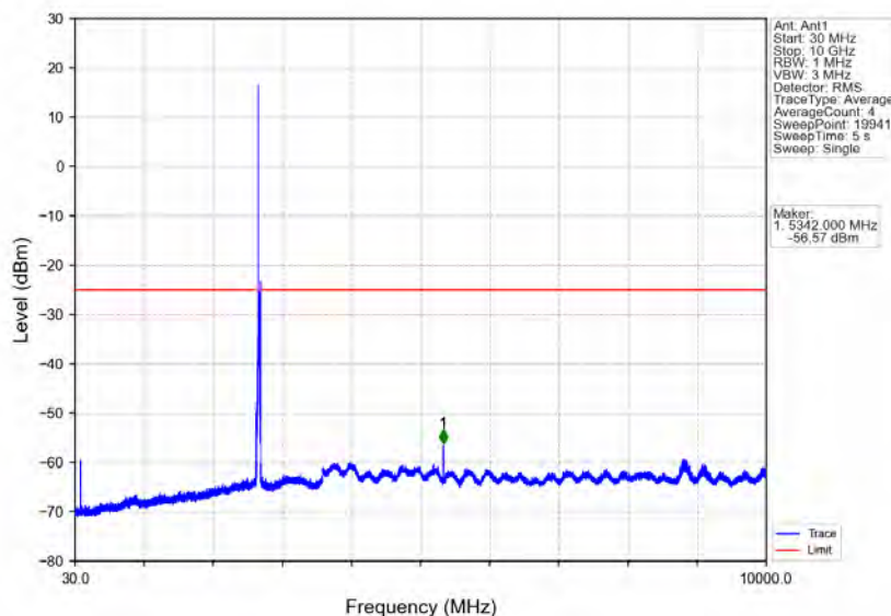
Band41_20MHz_QPSK_HCH_2680MHz_RB_1_0_NTNV
