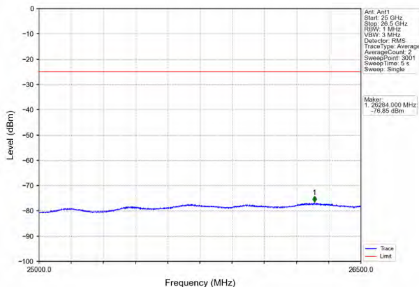
Band41_5MHz_QPSK_HCH_2687.5MHz_RB_1_24_NTNV
