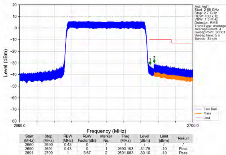
Band41_20MHz_QPSK_HCH_2680MHz_RB_100_0_NTNV
