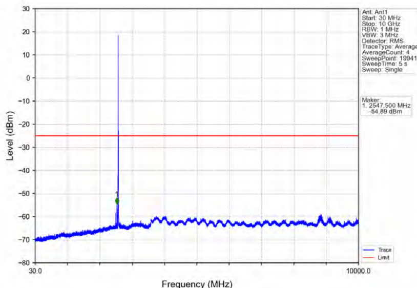
Band41_5MHz_QPSK_MCH_2593MHz_RB_1_0_NTNV
