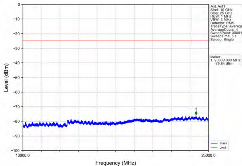
Band41_5MHz_QPSK_MCH_2593MHz_RB_1_0_NTNV
