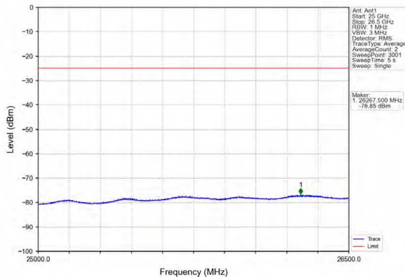
Band41_15MHz_QPSK_HCH_2682.5MHz_RB_1_74_NTNV
