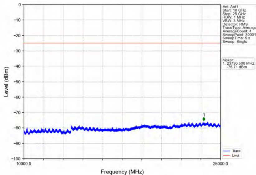
Band41_10MHz_16QAM_LCH_2501MHz_RB_1_0_NTNV
