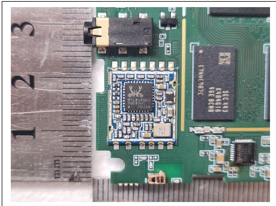
Antenna
