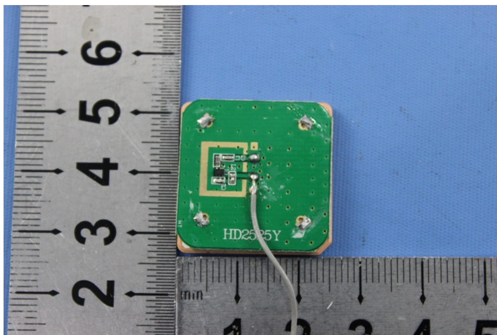
GPS Antenna
