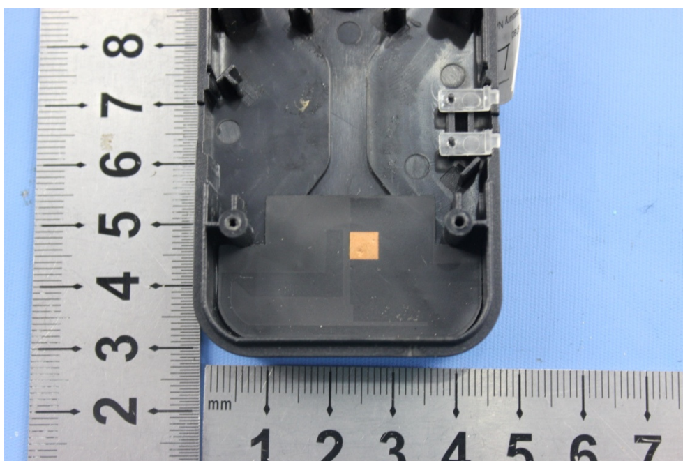
GSM Antenna
