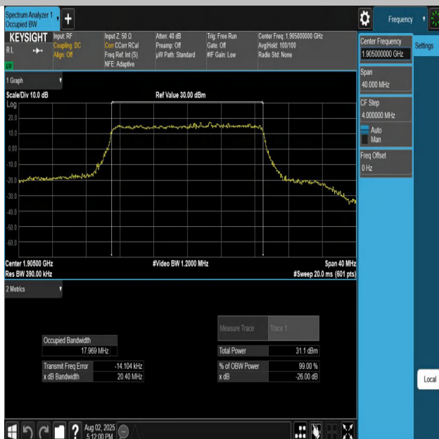
Band25-20MHz-QPSK-26590-100RB#0-PASS
