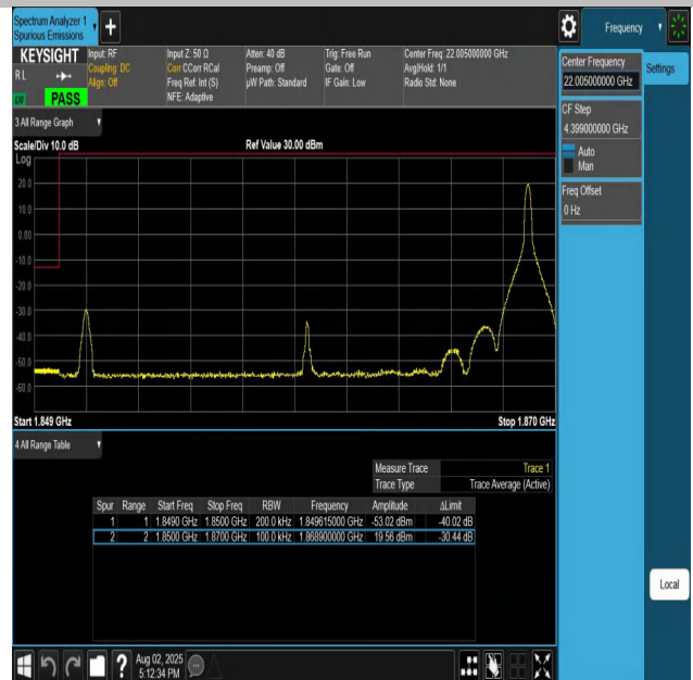
Band25-20MHz-QPSK-26140-1RB#99-PASS
