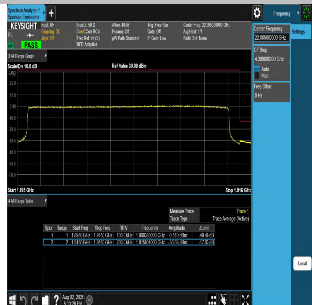
Band25-20MHz-QPSK-26590-100RB#0-PASS
