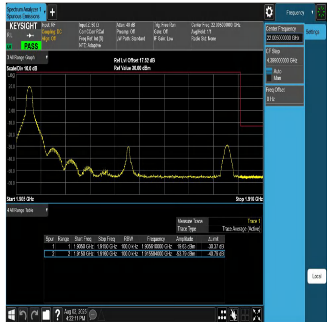
Band25-10MHz-QPSK-26640-1RB#0-PASS
