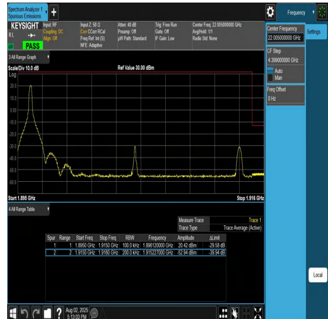
Band25-20MHz-QPSK-26590-1RB#0-PASS
