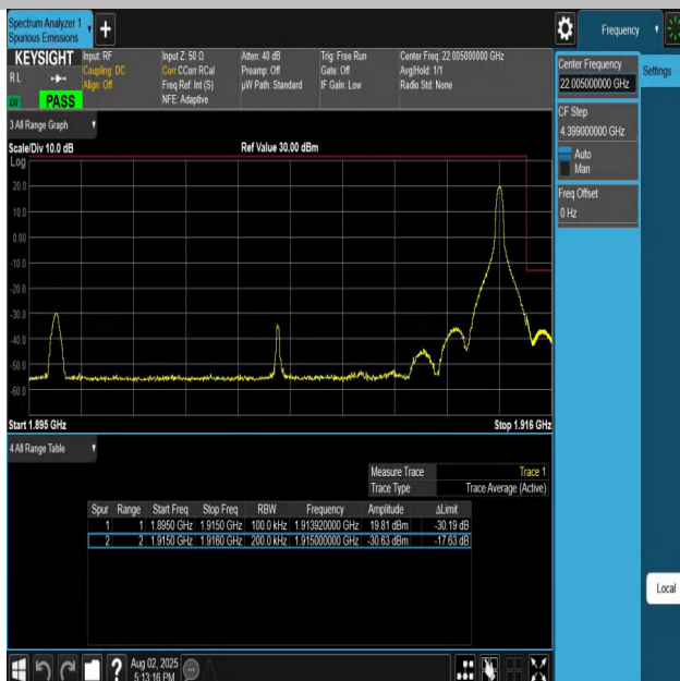
Band25-20MHz-QPSK-26590-1RB#99-PASS
