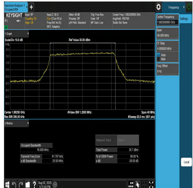
Band25-20MHz-QPSK-26365-100RB#0-PASS
