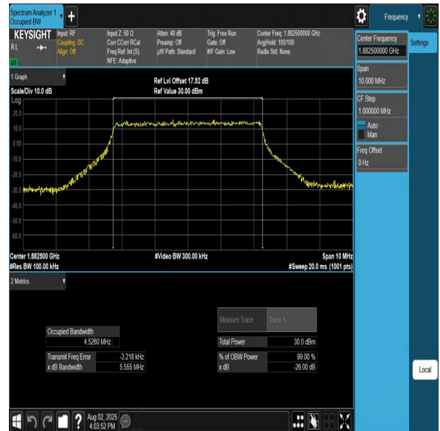
Band25-5MHz-QPSK-26365-25RB#0-PASS
