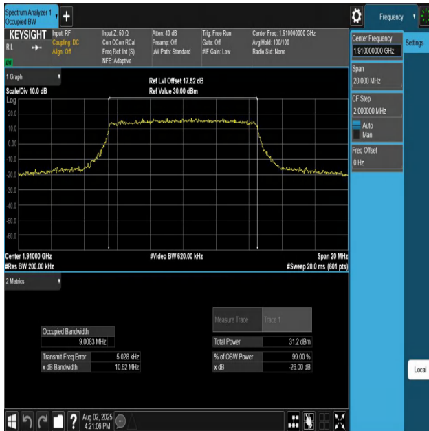
Band25-10MHz-QPSK-26640-50RB#0-PASS
