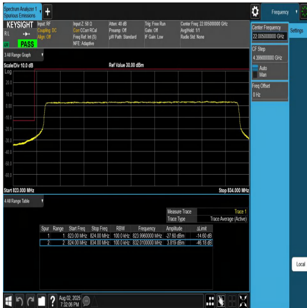
Band26(824-849)-10MHz-QPSK-26840-50RB#0-PASS
