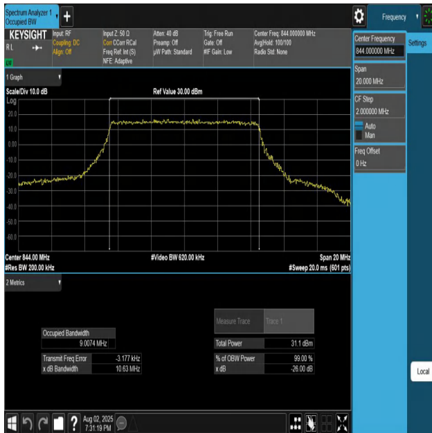
Band26(824-849)-10MHz-QPSK-26990-50RB#0-PASS
