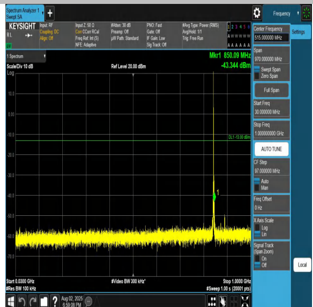
Band26(824-849)-3MHz-QPSK-27025-1RB#0-30~1000-P ASS
