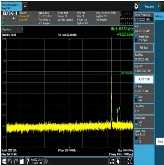
Band26(824-849)-3MHz-QPSK-26915-1RB#0-30~1000-P ASS
