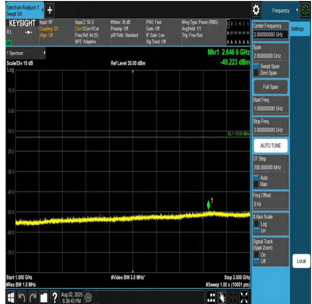
Band26(824-849)-1.4MHz-QPSK-26797-1RB#0-1000~300 0-PASS
