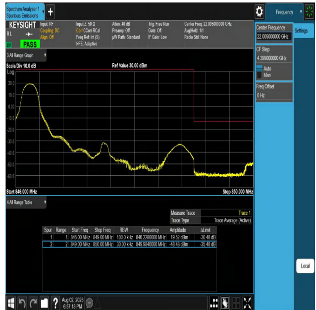
Band26(824-849)-3MHz-QPSK-27025-1RB#0-PASS
