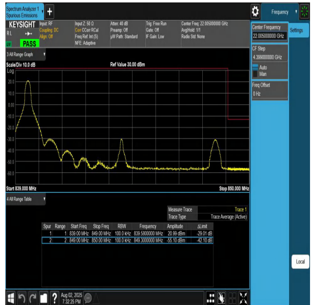
Band26(824-849)-10MHz-QPSK-26990-1RB#0-PASS
