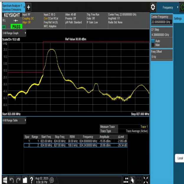
Band26(824-849)-3MHz-QPSK-26805-1RB#0-PASS
