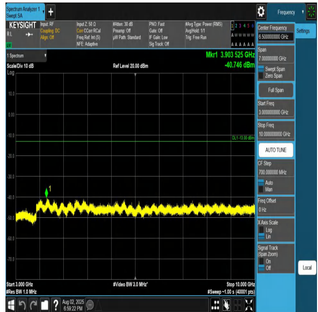
Band26(824-849)-3MHz-QPSK-27025-1RB#0-3000~1000 0-PASS
