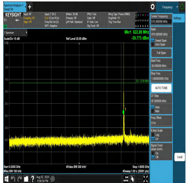
Band26(824-849)-3MHz-QPSK-26805-1RB#0-30~1000-P ASS
