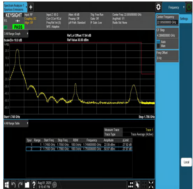
Band4-10MHz-QPSK-20350-1RB#0-PASS
