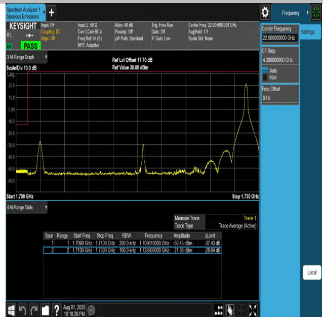
Band4-20MHz-QPSK-20050-1RB#99-PASS
