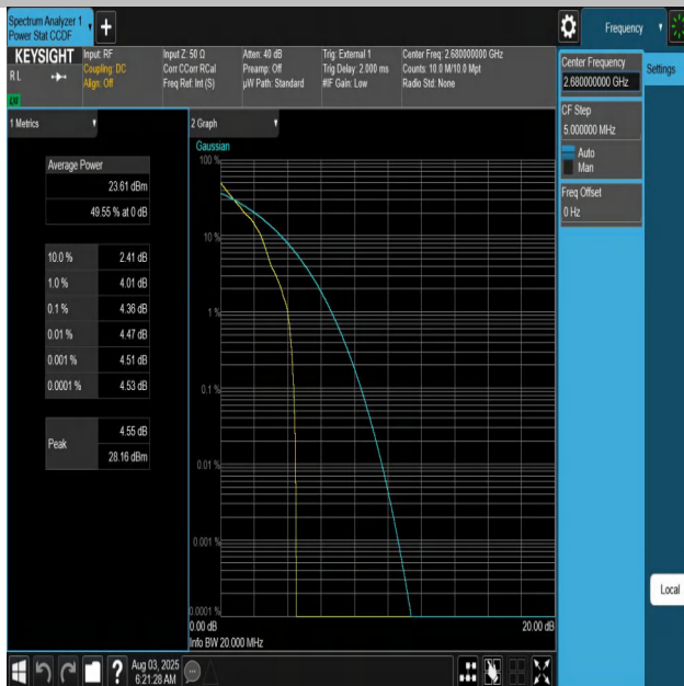
Band41-20MHz-QPSK-41490-1RB#0-PASS
