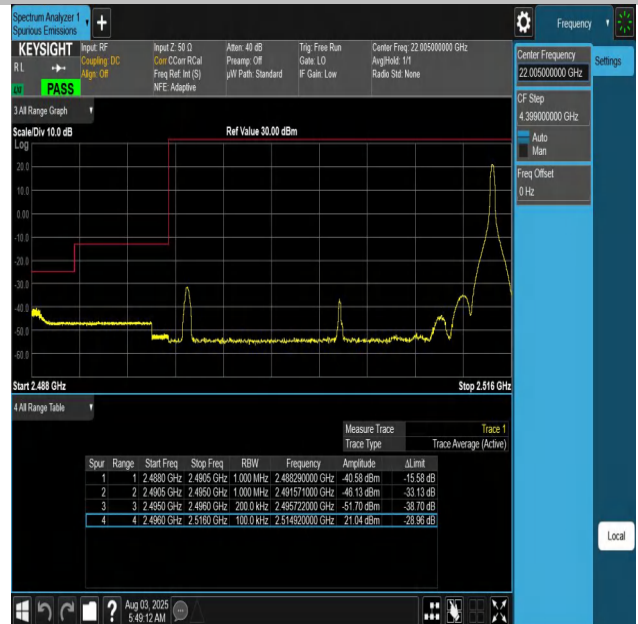
Band41-20MHz-QPSK-39750-1RB#99-PASS
