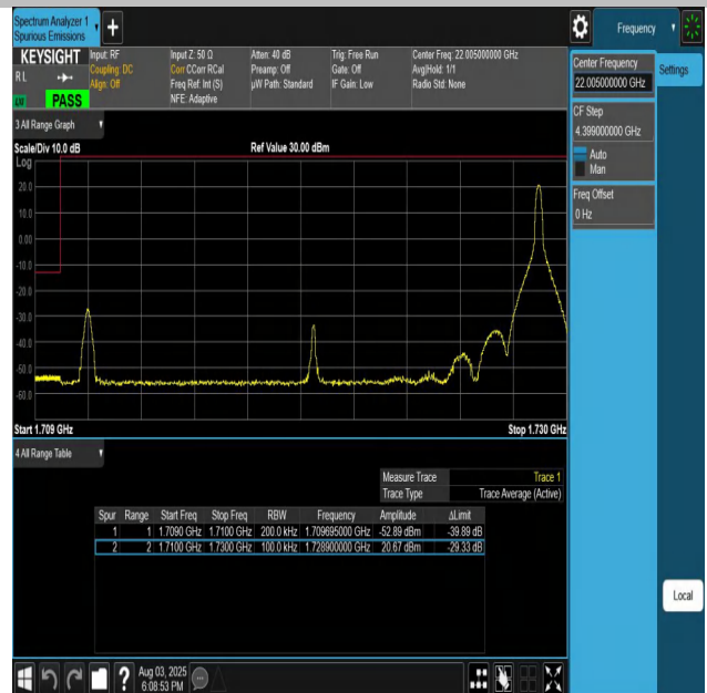
Band66-20MHz-QPSK-132072-1RB#99-PASS
