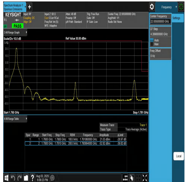
Band66-20MHz-QPSK-132572-1RB#0-PASS
