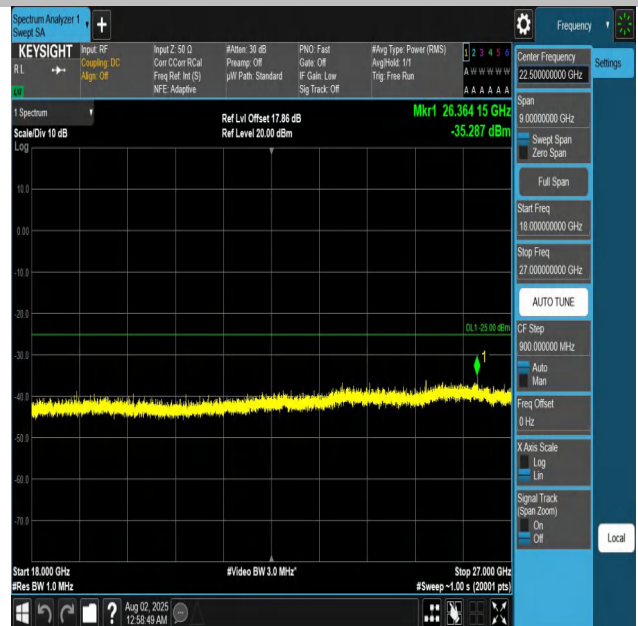
Band7-15MHz-QPSK-20825-1RB#0-18000~27000-PASS
