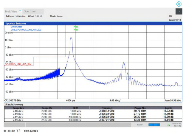
NTVN-n41-PC2-30-20-L-DFT-QPSK-Edge_1RB_Left-PASS
