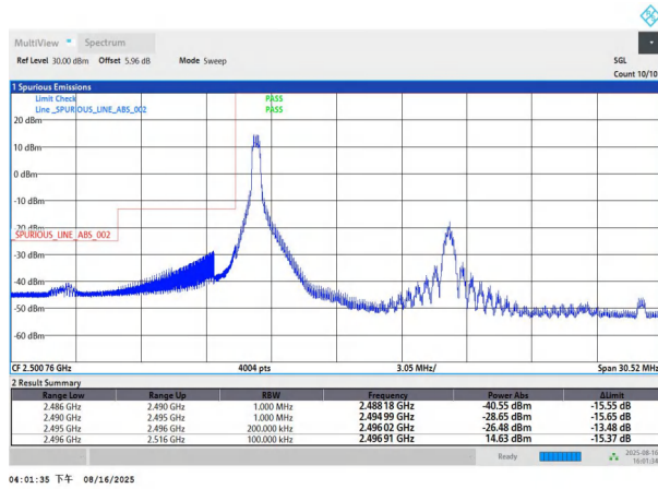
NTVN-n41-PC2-30-20-L-DFT-BPSK-Edge_1RB_Left-PASS
