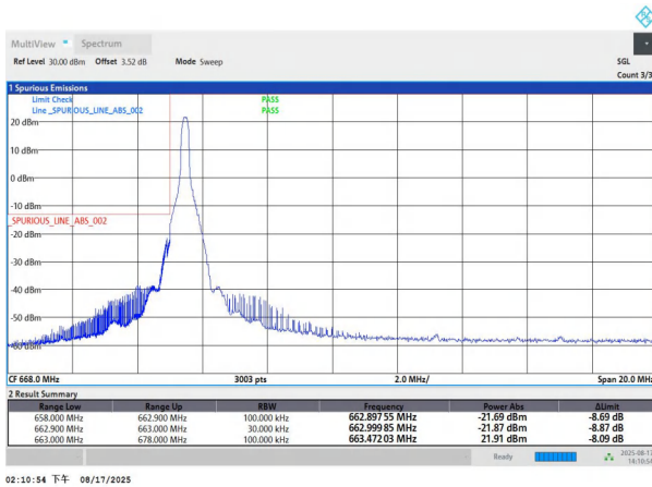
NTNV-n71-PC3-15-15-L-DFT-QPSK-Edge_1RB_Left-PASS
