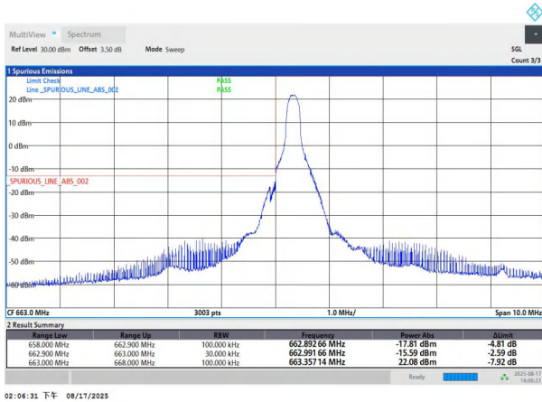
NTNV-n71-PC3-15-5-L-DFT-QPSK-Edge_1RB_Left-PASS
