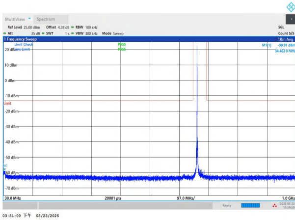
NTNV-n71-PC3-15-20-M-DFT-BPSK-Edge_1RB_Left-30-1000-P ASS
