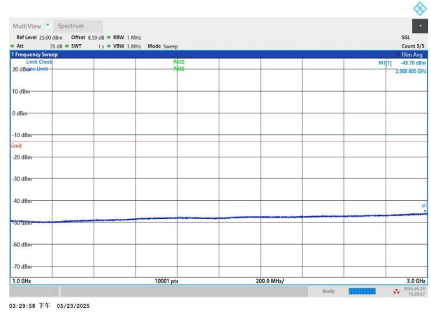
NTNV-n71-PC3-15-10-M-CP-QPSK-Edge_1RB_Left-1000-3000-P ASS
