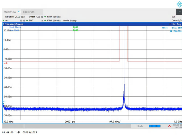
NTNV-n71-PC3-15-15-H-DFT-QPSK-Edge_1RB_Left-30-1000-P ASS
