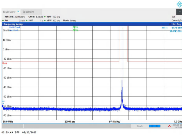
NTNV-n71-PC3-15-15-M-DFT-QPSK-Edge_1RB_Left-30-1000-P ASS
