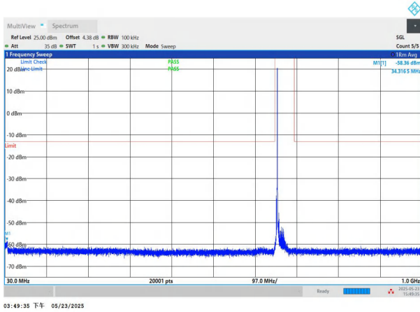
NTNV-n71-PC3-15-20-L-CP-QPSK-Edge_1RB_Left-30-1000-PA SS
