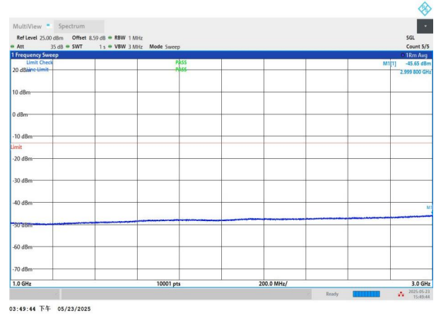
NTNV-n71-PC3-15-20-L-CP-QPSK-Edge_1RB_Left-1000-3000-P ASS
