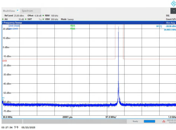
NTNV-n71-PC3-15-10-M-DFT-QPSK-Edge_1RB_Left-30-1000-P ASS
