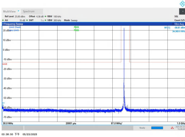
NTNV-n71-PC3-15-15-M-DFT-BPSK-Edge_1RB_Left-30-1000-P ASS
