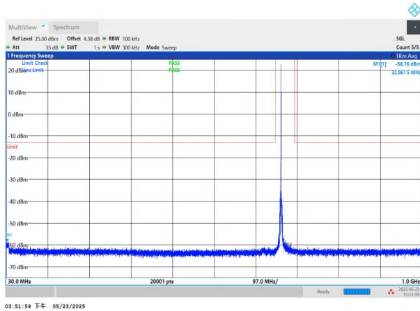
NTNV-n71-PC3-15-20-M-DFT-QPSK-Edge_1RB_Left-30-1000-P ASS
