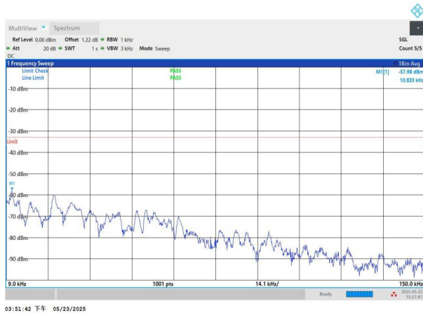
NTNV-n71-PC3-15-20-M-DFT-QPSK-Edge_1RB_Left-0.009-0.15 -PASS
