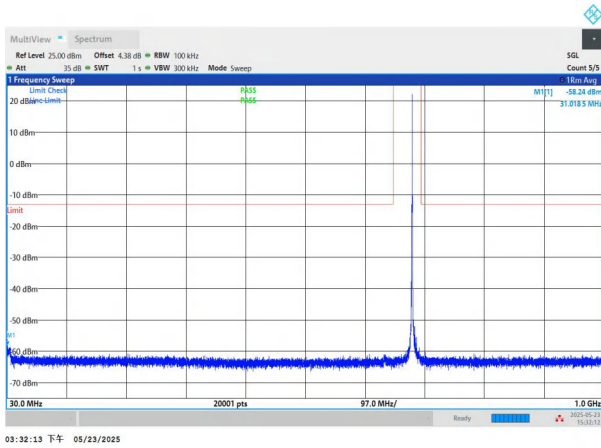
NTNV-n71-PC3-15-10-H-DFT-QPSK-Edge_1RB_Left-30-1000-P- ASS
