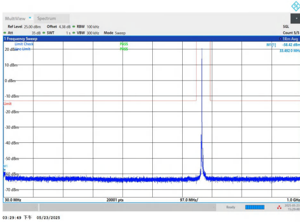
NTNV-n71-PC3-15-10-M-CP-QPSK-Edge_1RB_Left-30-1000-PA SS
