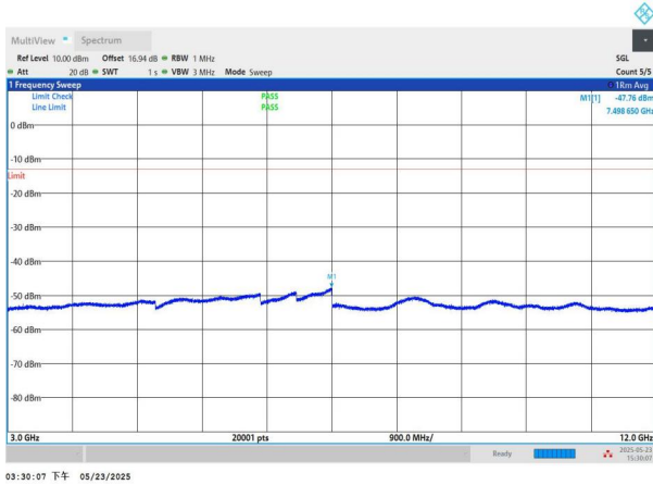
NTNV-n71-PC3-15-10-M-CP-QPSK-Edge_1RB_Left-3000-12000 -PASS
