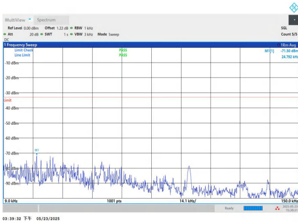
NTNV-n71-PC3-15-15-M-DFT-QPSK-Edge_1RB_Left-0.009-0.15 -PASS
