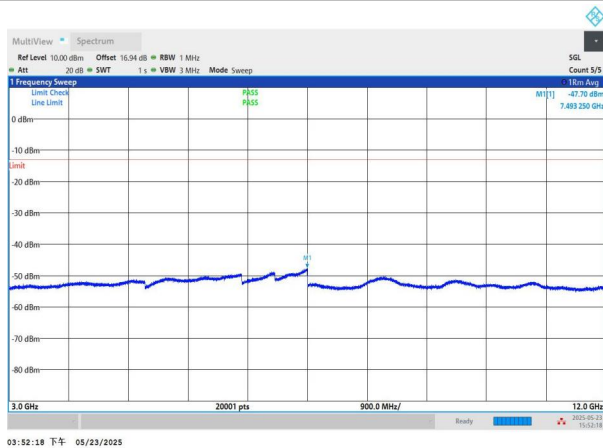
NTNV-n71-PC3-15-20-M-DFT-QPSK-Edge_1RB_Left-3000-1200 0-PASS
