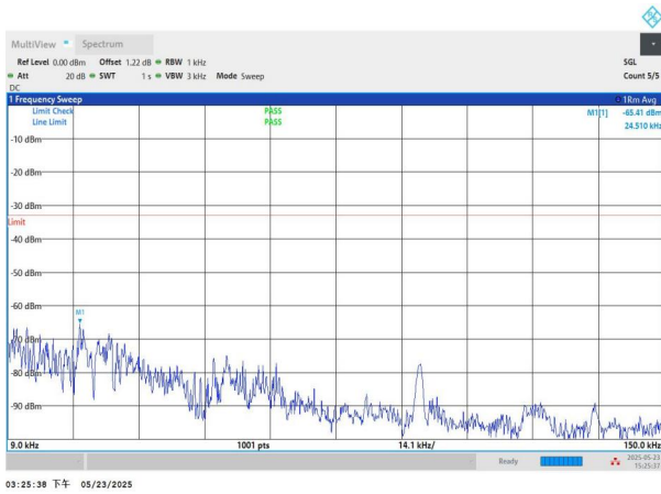
NTNV-n71-PC3-15-10-M-DFT-QPSK-Edge_1RB_Left-0.009-0.15 -PASS
