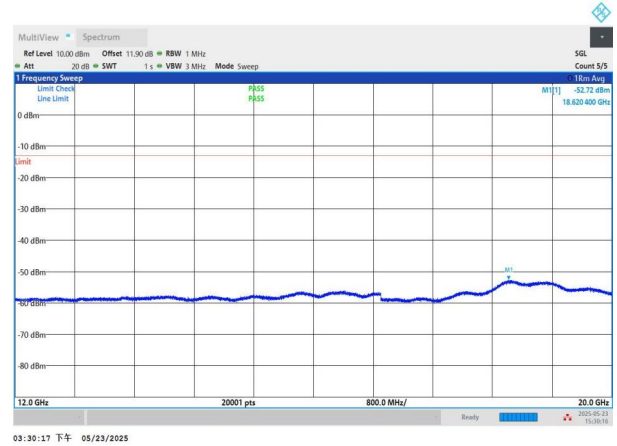
NTNV-n71-PC3-15-10-M-CP-QPSK-Edge_1RB_Left-12000-20000 -PASS
