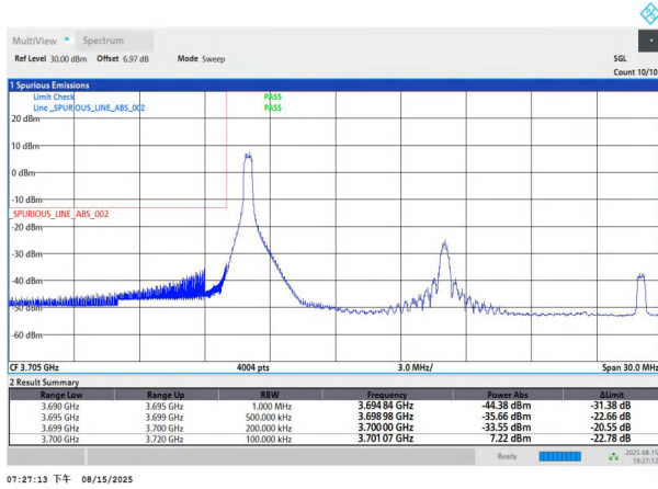
NTNV-n77(3700-3980)-PC2-30-20-L-DFT-BPSK-Edge_1RB_Left-PA SS
