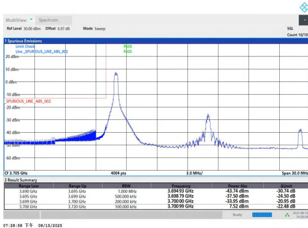
NTNV-n77(3700-3980)-PC2-30-20-L-DFT-QPSK-Edge_1RB_Left-PA SS
