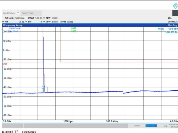
NTNV-n77(3700-3980)-PC2-30-20-L-DFT-BPSK-Edge_1RB_Left- 3000-6000-PASS
