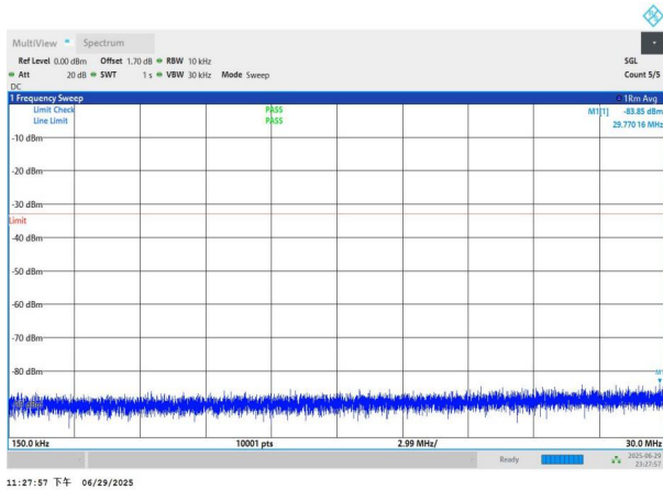
NTNV-n77(3700-3980)-PC2-30-30-L-DFT-QPSK-Edge_1RB_Left- 0.15-30-PASS
