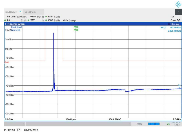
NTNV-n77(3700-3980)-PC2-30-20-M-DFT-QPSK-Edge_1RB_Left -3000-6000-PASS
