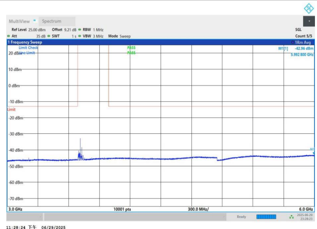
NTNV-n77(3700-3980)-PC2-30-30-L-DFT-QPSK-Edge_1RB_Left- 3000-6000-PASS
