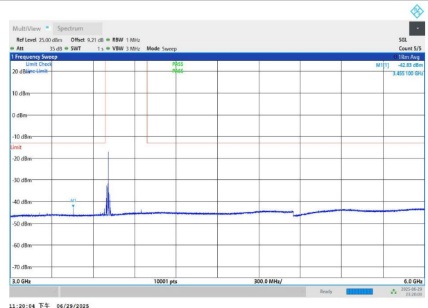
NTNV-n77(3700-3980)-PC2-30-20-L-DFT-QPSK-Edge_1RB_Left- 3000-6000-PASS
