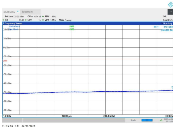
NTNV-n77(3700-3980)-PC2-30-20-L-DFT-QPSK-Edge_1RB_Left- 1000-3000-PASS
