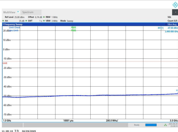
NTNV-n77(3700-3980)-PC2-30-30-L-DFT-QPSK-Edge_1RB_Left- 1000-3000-PASS
