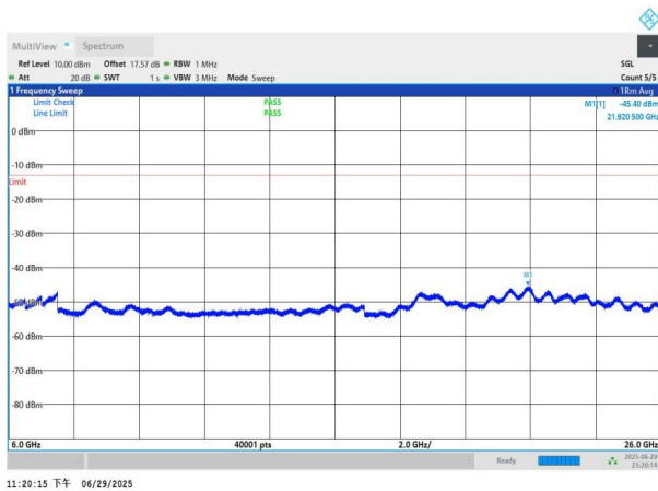
NTNV-n77(3700-3980)-PC2-30-20-L-DFT-QPSK-Edge_1RB_Left- 6000-26000-PASS
