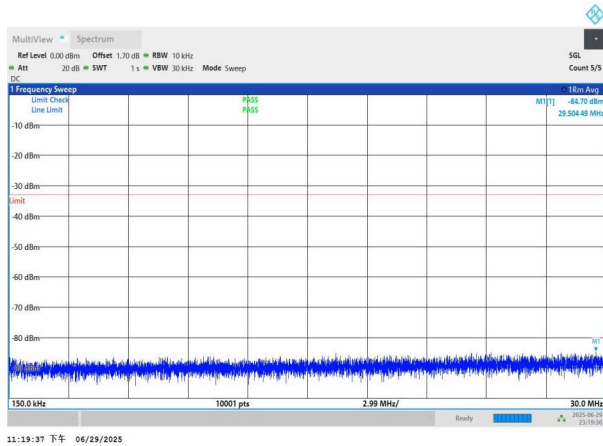
NTNV-n77(3700-3980)-PC2-30-20-L-DFT-QPSK-Edge_1RB_Left- 0.15-30-PASS
