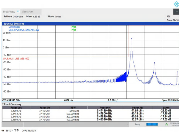
NTNV-n77(3450-3550)-PC2-30-20-L-DFT-QPSK-Edge_1RB_Left-PASS
