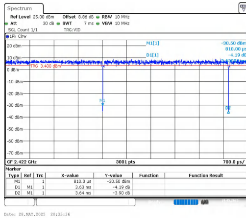
NTNV-11AX40MIMO-Ant1-2422
