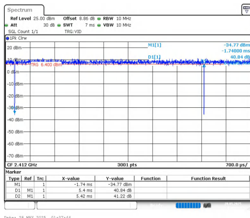
NTNV-11AX20MIMO-Ant1-2412
