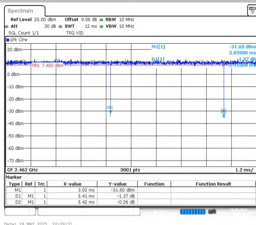
NTNV-11AX20MIMO-Ant1-2462
