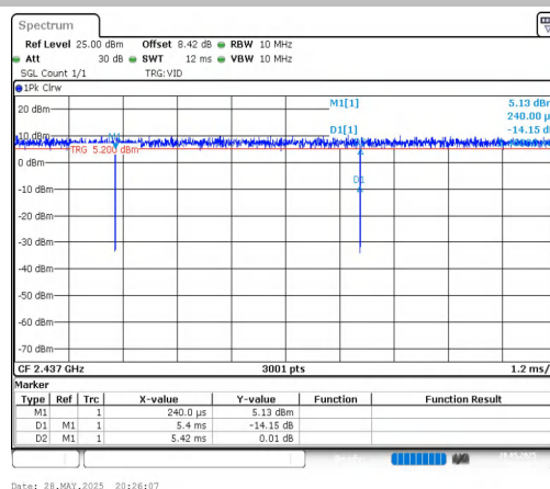
NTNV-11AX20MIMO-Ant2-2437
