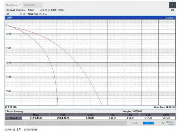
Band2-5MHz-QPSK-18900-25RB#0-PASS
