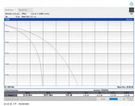
Band2-10MHz-QPSK-18650-50RB#0-PASS
