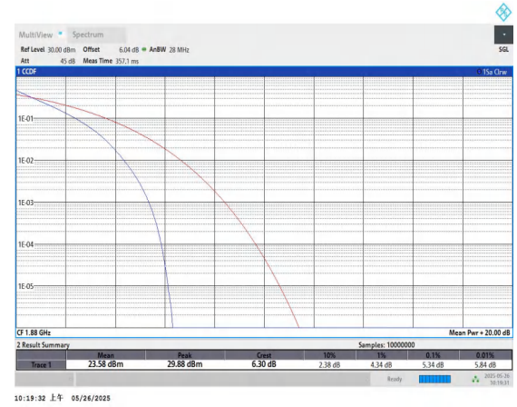
Band2-10MHz-QPSK-18900-50RB#0-PASS
