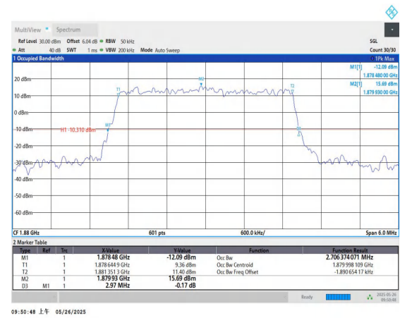
Band2-3MHz-QPSK-18900-15RB#0-PASS
