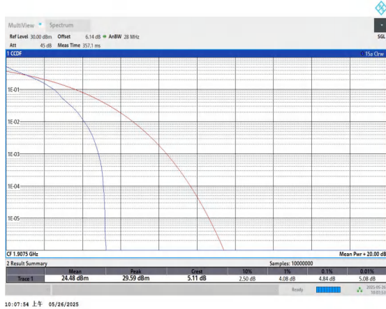
Band2-5MHz-QPSK-19175-1RB#0-PASS
