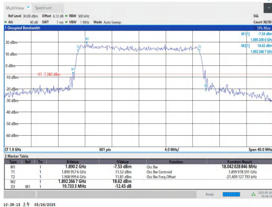
Band2-20MHz-QPSK-19100-100RB#0-PASS
