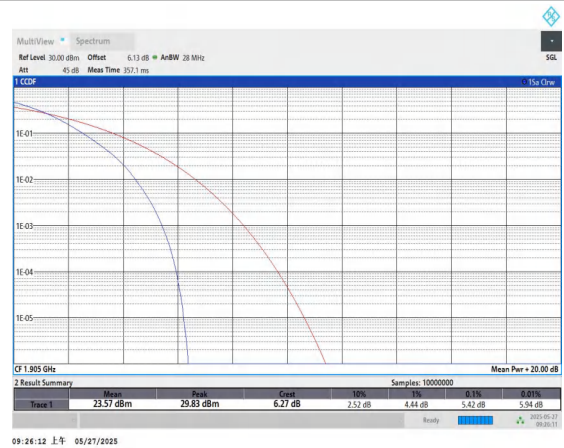
Band25-20MHz-QPSK-26590-100RB#0-PASS
