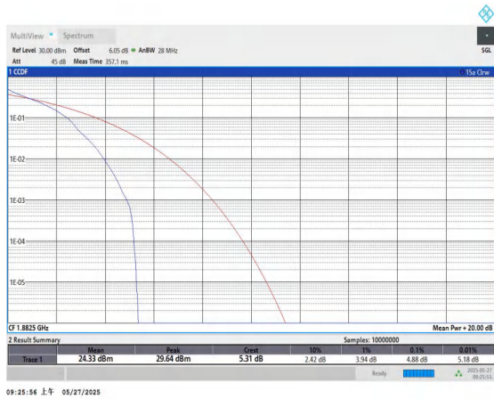
Band25-20MHz-QPSK-26365-1RB#0-PASS
