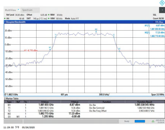
Band25-1.4MHz-QPSK-26365-6RB#0-PASS
