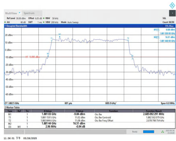
Band25-3MHz-QPSK-26365-15RB#0-PASS
