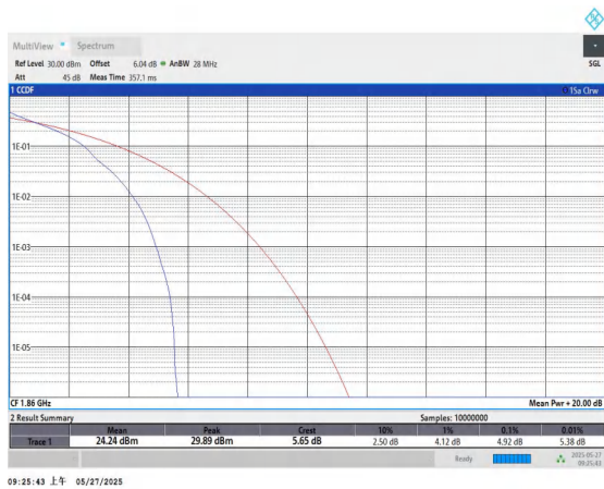
Band25-20MHz-QPSK-26140-1RB#0-PASS
