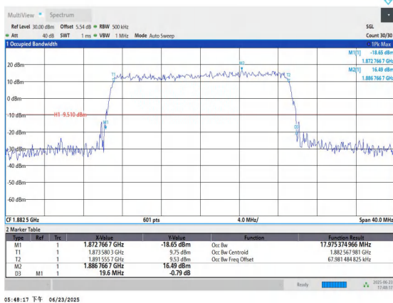
Band25-20MHz-16QAM-26365-100RB#0-PASS
