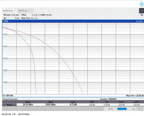
Band25-20MHz-QPSK-26590-1RB#0-PASS
