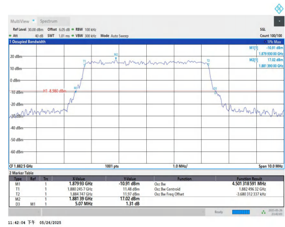
Band25-5MHz-QPSK-26365-25RB#0-PASS
