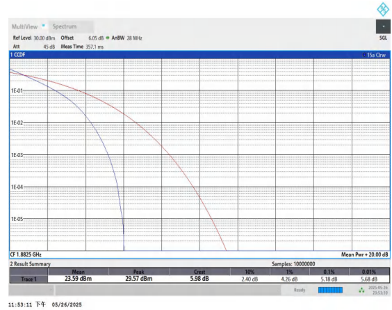
Band25-10MHz-QPSK-26365-50RB#0-PASS
