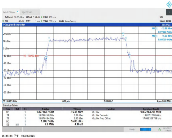
Band25-10MHz-16QAM-26365-50RB#0-PASS
