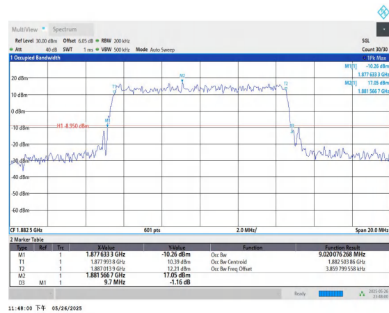
Band25-10MHz-QPSK-26365-50RB#0-PASS
