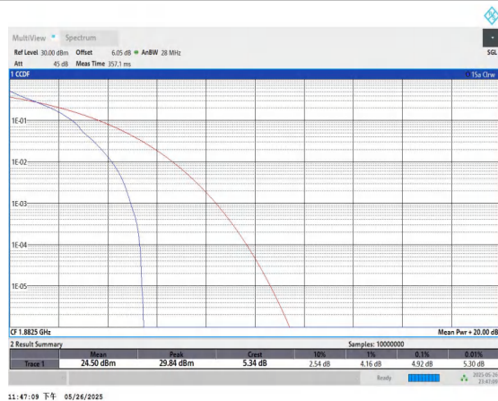
Band25-5MHz-QPSK-26365-1RB#0-PASS
