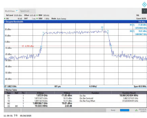
Band25-20MHz-QPSK-26365-100RB#0-PASS
