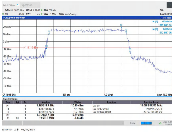
Band25-20MHz-QPSK-26590-100RB#0-PASS
