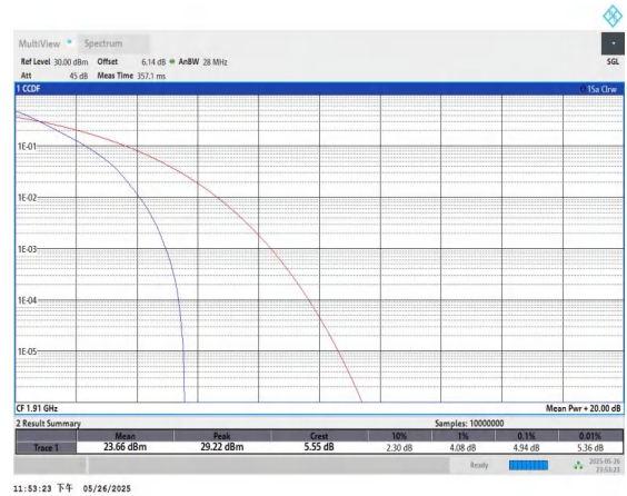
Band25-10MHz-QPSK-26640-50RB#0-PASS
