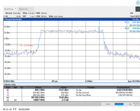
26(824-849)-10MHz-16QAM-26990-50RB#0-PASS
