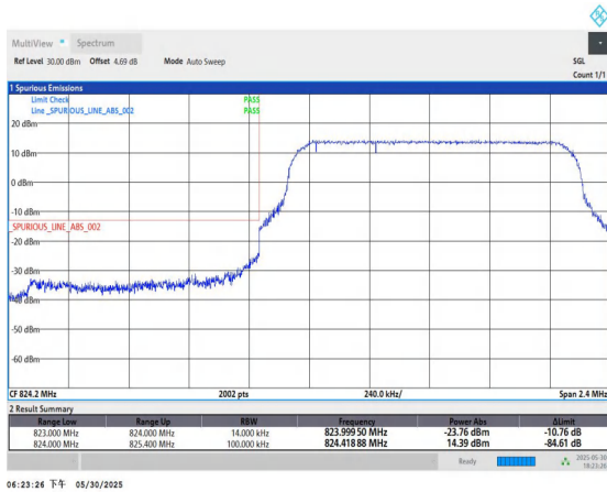
26(824-849)-1.4MHz-QPSK-26797-6RB#0-PASS
