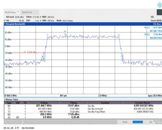
26(824-849)-10MHz-QPSK-26915-50RB#0-PASS
