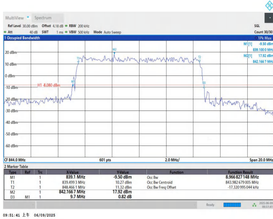
26(824-849)-10MHz-QPSK-26990-50RB#0-PASS
