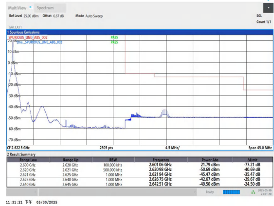
Band38-20MHz-QPSK-38150-1RB#0-PASS
