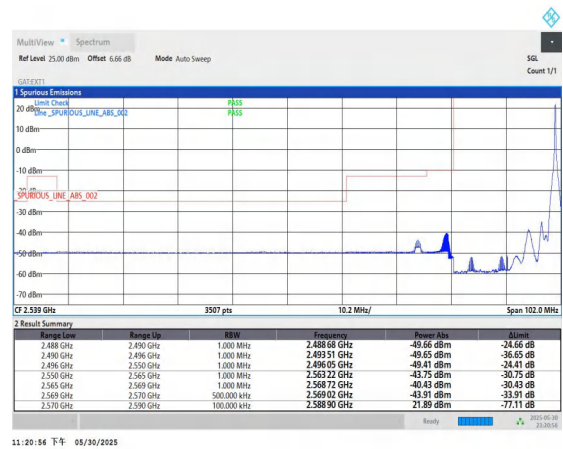
Band38-20MHz-QPSK-37850-1RB#99-PASS
