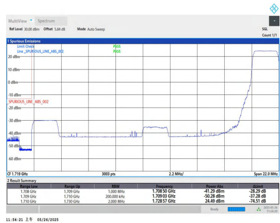
Band4-20MHz-QPSK-20050-1RB#99-PASS
