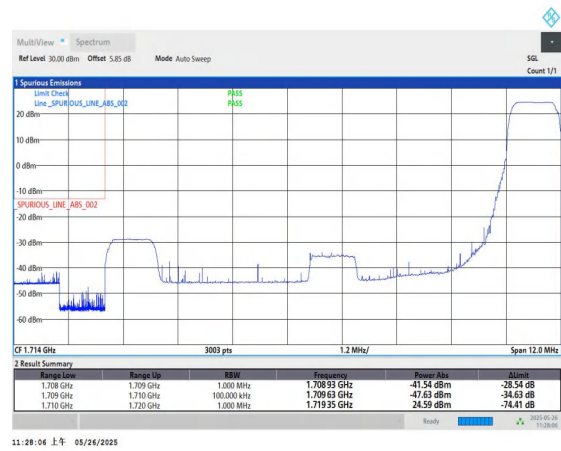
Band4-10MHz-QPSK-20000-1RB#49-PASS
