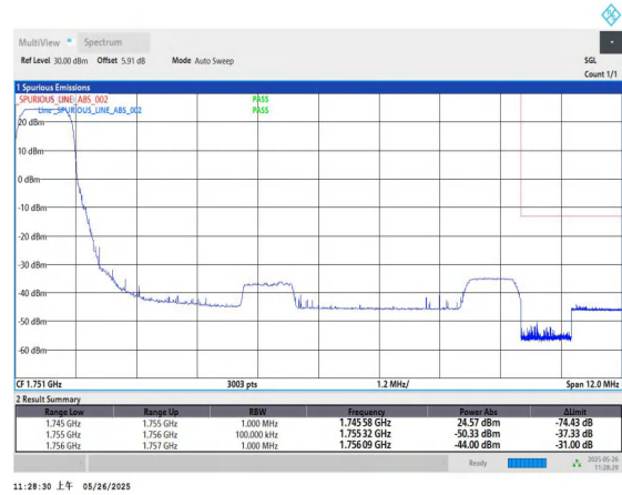
Band4-10MHz-QPSK-20350-1RB#0-PASS
