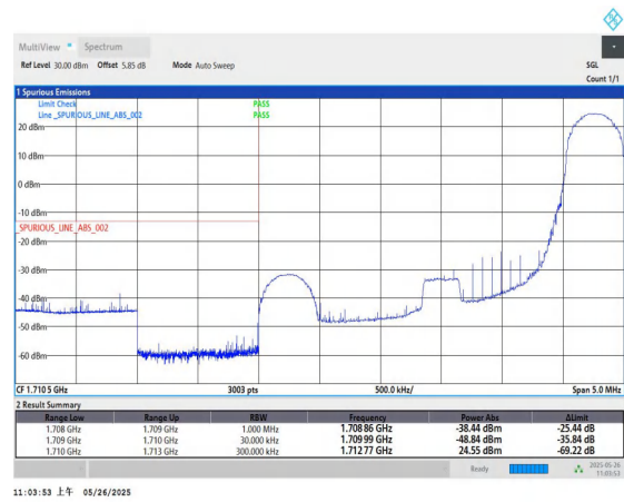
Band4-3MHz-QPSK-19965-1RB#14-PASS
