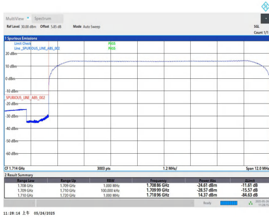
Band4-10MHz-QPSK-20000-50RB#0-PASS
