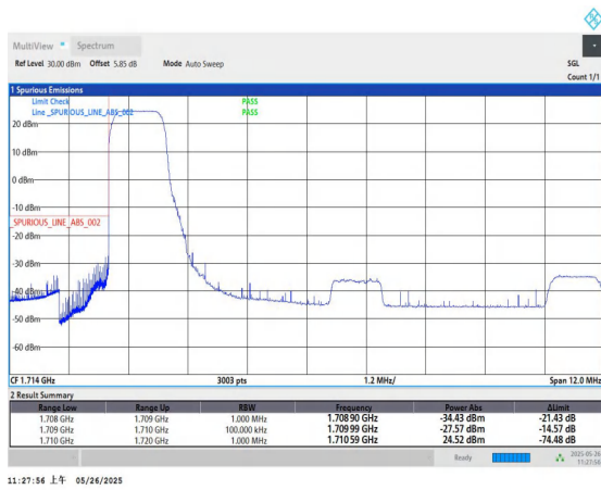
Band4-10MHz-QPSK-20000-1RB#0-PASS
