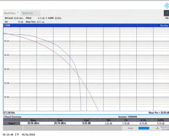
Band41-20MHz-QPSK-41490-1RB#0-PASS
