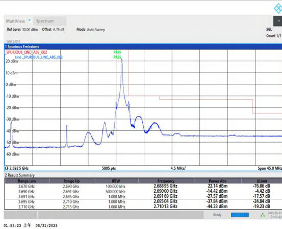
Band41-20MHz-QPSK-41490-1RB#99-PASS
