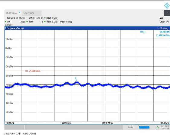
Band41-5MHz-16QAM-41565-1RB#0-18000~27000-PASS
