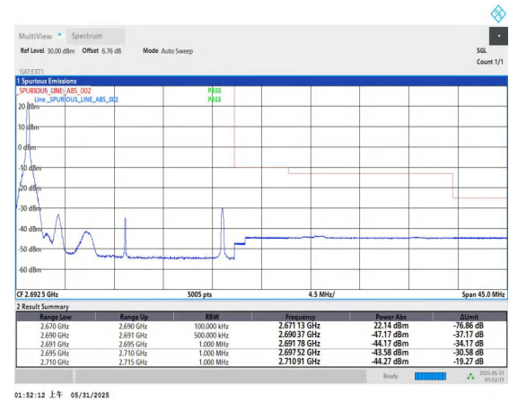
Band41-20MHz-QPSK-41490-1RB#0-PASS
