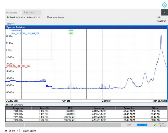
Band41-20MHz-QPSK-39750-1RB#99-PASS
