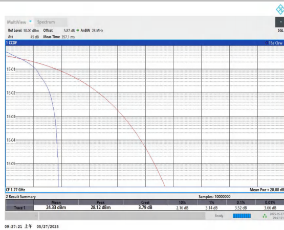
Band66-20MHz-QPSK-132572-1RB#0-PASS
