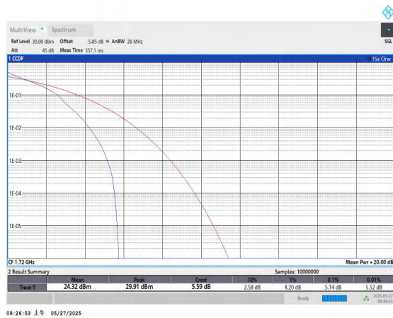
Band66-20MHz-QPSK-132072-1RB#0-PASS
