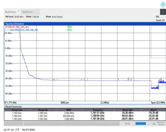
Band66-20MHz-QPSK-132572-1RB#0-PASS
