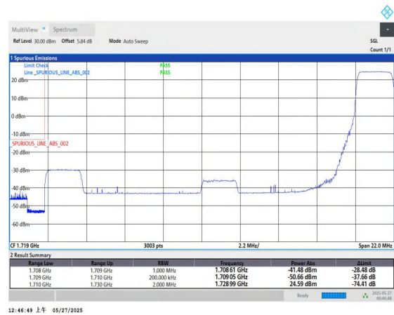
Band66-20MHz-QPSK-132072-1RB#99-PASS
