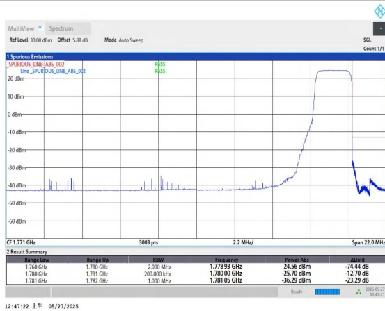
Band66-20MHz-QPSK-132572-1RB#99-PASS
