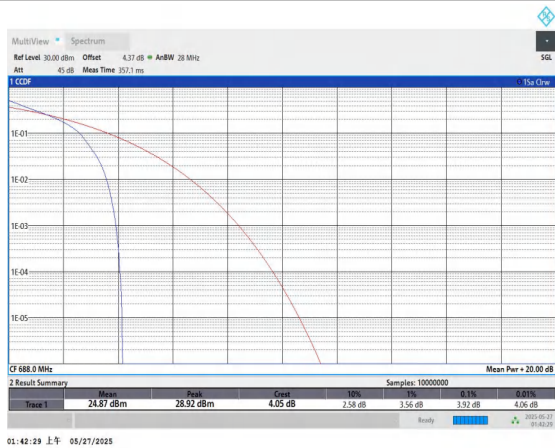
Band71-20MHz-QPSK-133372-1RB#0-PASS
