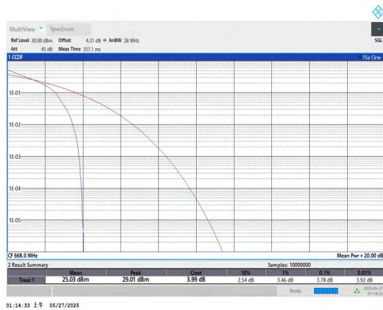
Band71-10MHz-QPSK-133172-1RB#0-PASS
