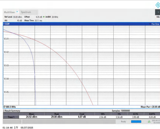
Band71-10MHz-QPSK-133297-1RB#0-PASS
