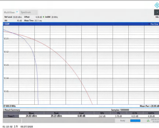
Band71-10MHz-QPSK-133422-1RB#0-PASS
