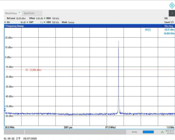
Band71-20MHz-QPSK-133372-1RB#0-30~1000-PASS
