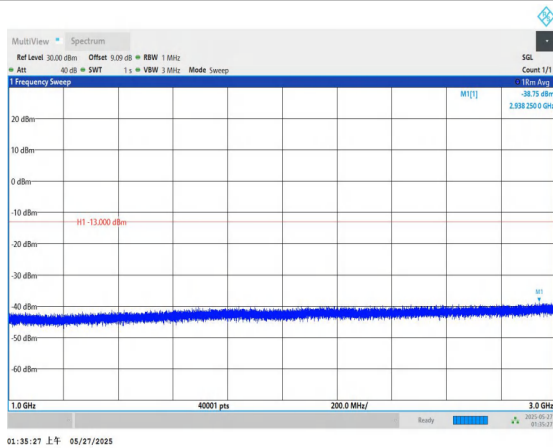
Band71-20MHz-QPSK-133372-1RB#0-1000~3000-PASS
