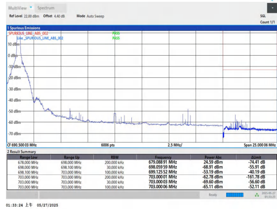
Band71-20MHz-QPSK-133372-1RB#0-PASS
