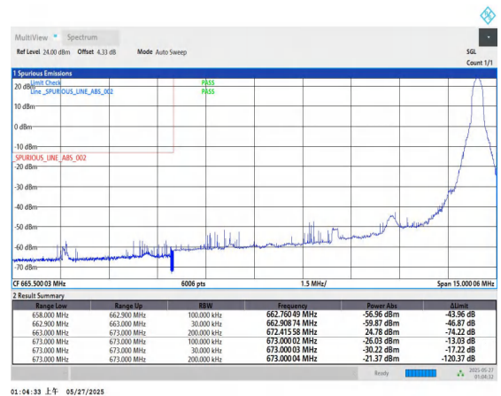
Band71-10MHz-QPSK-133172-1RB#49-PASS
