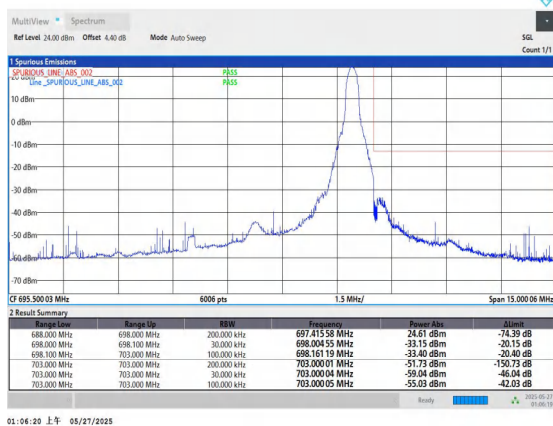
Band71-10MHz-QPSK-133422-1RB#49-PASS
