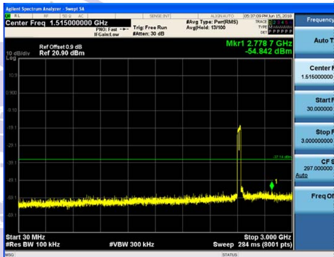
30MHz-3GHz
