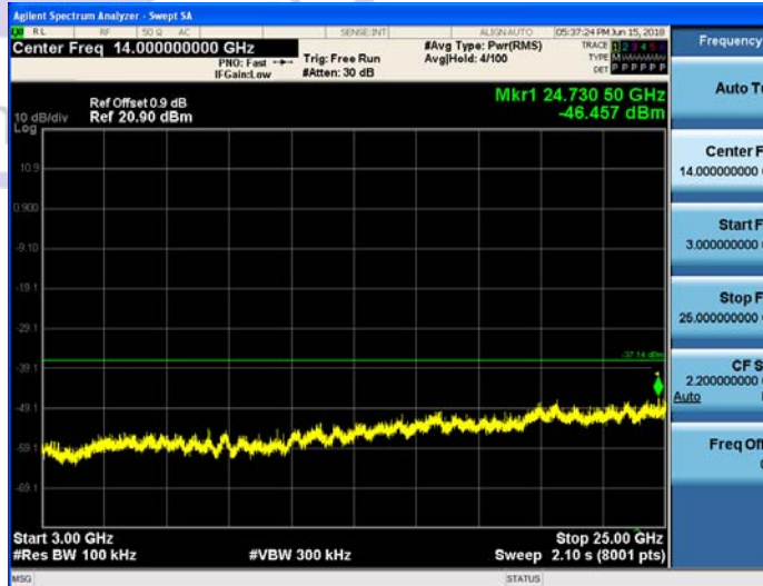
3GHz-25GHz
