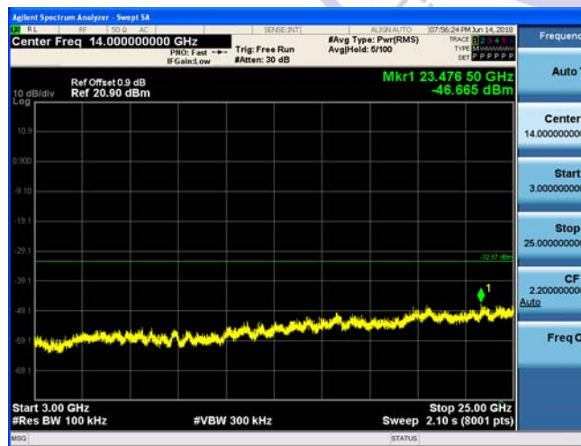
3GHz-25GHz
