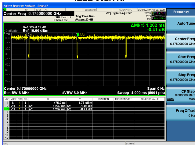
IEEE 802.11a
