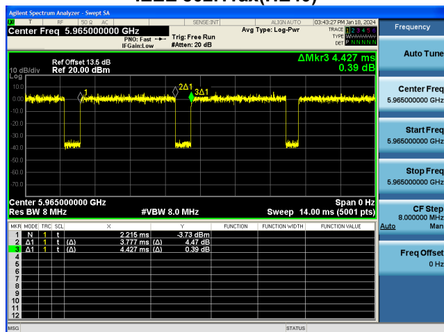
IEEE 802.11ax(HE40)
