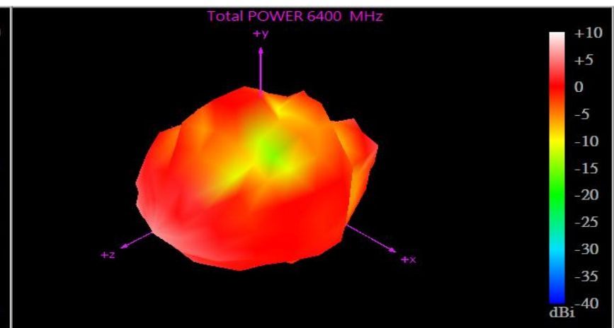
6400 MHz
