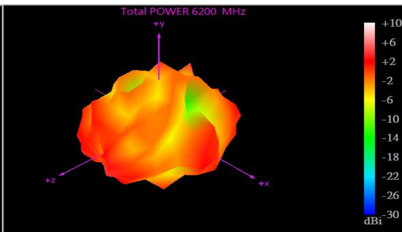
6200 MHz
