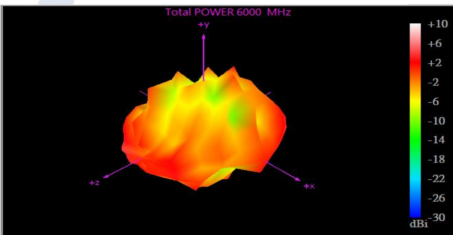
6000 MHz
