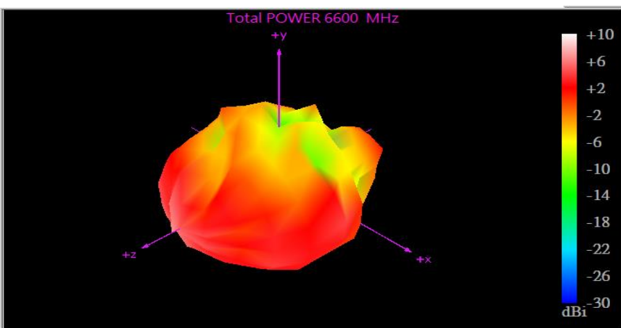
6600 MHz
