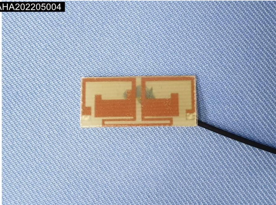
EUT Photo (12)
