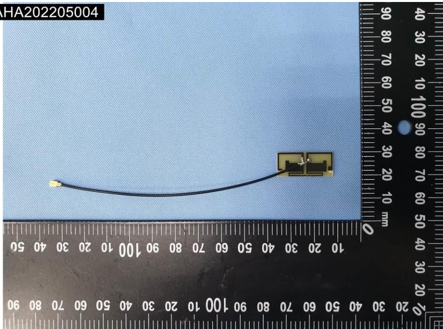
EUT Photo (8)
