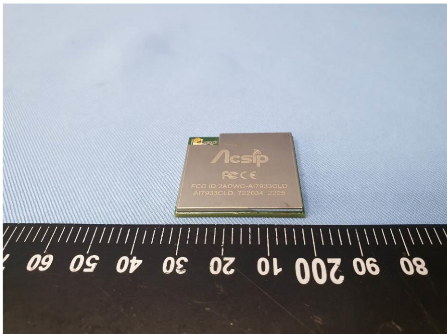
EUT Photo (4)
