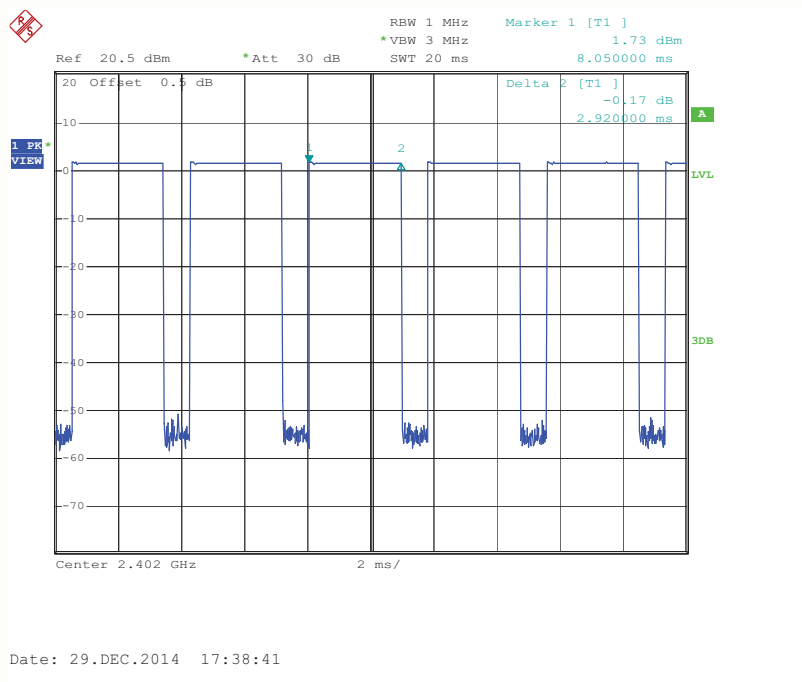
2402 MHz_DH5
